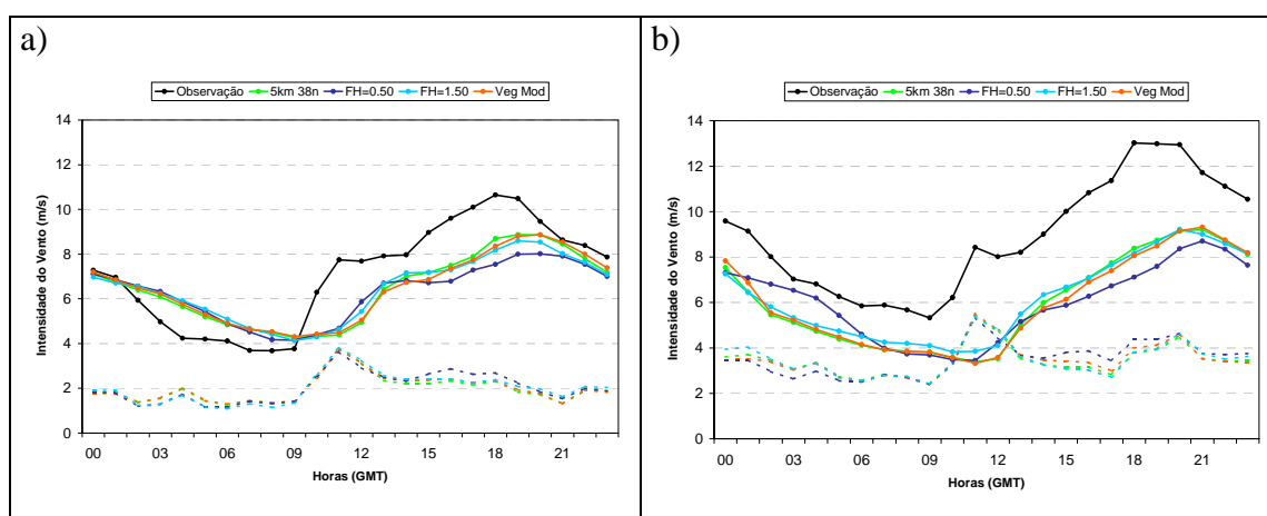
Figura 5.30 – Ciclo diário médio da velocidade do vento (m/s) (linha cheia) a (a) 10 m e (b) 50 m de altura observado e previsto de 24-48h pelos experimentos controle (linha verde), Eta5L38 FH=0,5 (linha azul escura), Eta5L38 FH=1,5 (linha azul clara) e Eta5L38 vegmod (linha laranja) para Macau. A linha tracejada indica o ciclo diário do RMSE para cada experimento.
