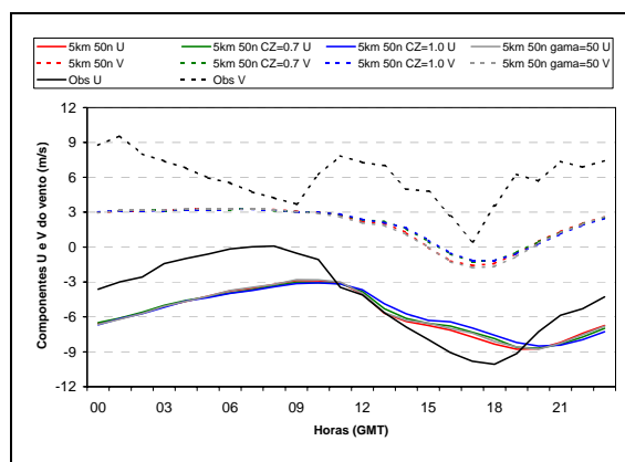
Figura 5.20 – Ciclo diário médio das componentes U (linhas sólidas) e V (linhas tracejadas) do vento (m/s) a 10 m de altura observado e previsto de 24-48h pelos experimentos Eta5L50 (linha vermelha), Eta5L50 CZ=0,7 (linha verde), Eta5L50 CZ=1,0 (linha azul) e Eta5L50 \gamma=50 (linha cinza) para Macau.
