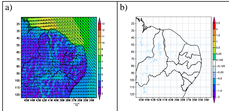
Figura 5.16 – (a) Média do campo de vento (m/s) a 10 m de altura das previsões de 24-48h para o período de 15 a 28 de setembro de 2005 do experimento Eta5L50 \gamma=50 , (b) diferença entre a magnitude do vento médio dos experimentos Eta5L50 \gamma=50 e controle.
