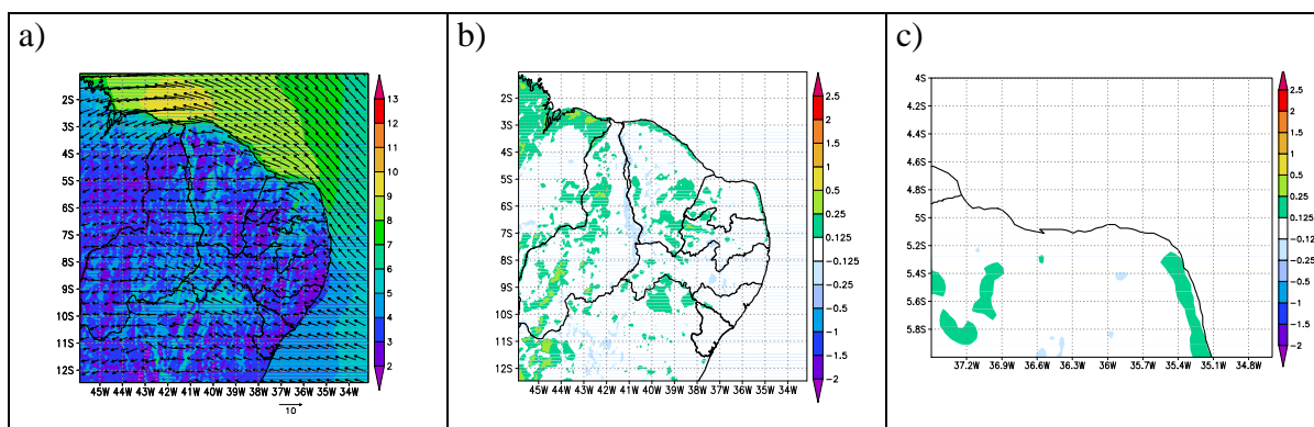
Figura 5.14 – (a) Média do campo de vento (m/s) a 10 m de altura das previsões de 24-48h para o período de 15 a 28 de setembro de 2005 do experimento Eta5L50 CZ=0,7, (b) diferença entre a magnitude do vento médio dos experimentos Eta5L50 CZ=0,7 e controle e (c) detalhe sobre RN.
