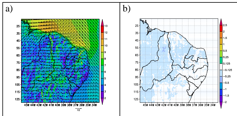
Figura 5.28 – (a) Média do campo de vento (m/s) a 50 m de altura das previsões de 24-48h para o período de 15 a 28 de setembro de 2005 do experimento Eta5L38 vegmod, (b) diferença entre a magnitude do vento médio dos experimentos Eta5L38 vegmod e controle.
