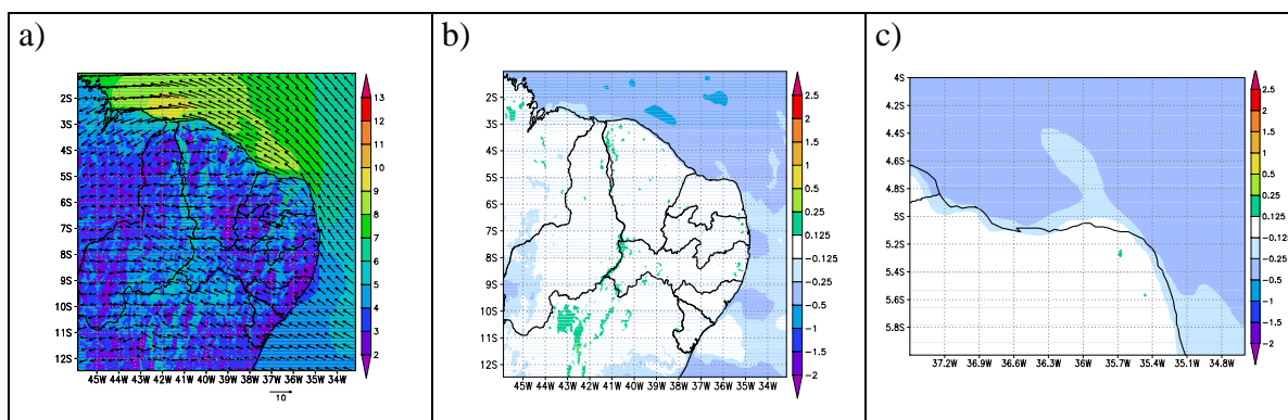
Figura 5.25 – (a) Média do campo de vento (m/s) a 10 m de altura das previsões de 24-48h para o período de 15 a 28 de setembro de 2005 do experimento Eta5L38 FH=1,5, (b) diferença entre a magnitude do vento médio dos experimentos Eta5L38 FH=1,5 e controle e (c) detalhe sobre RN.
