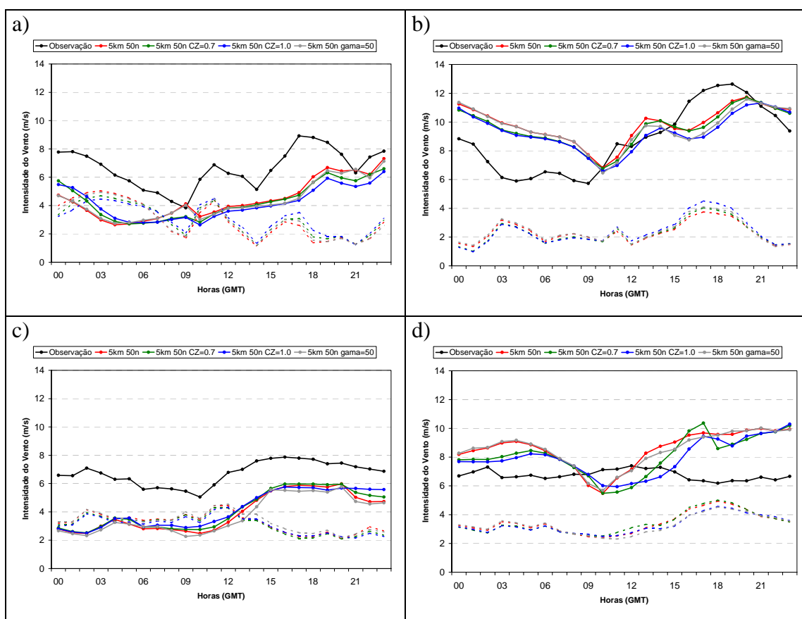
Figura 5.23 – Ciclo diário médio da velocidade do vento (m/s) (linha cheia) a 50 m de altura observado e previsto de 24-48h pelos experimentos \text{Eta5L50} (linha vermelha), \text{Eta5L50 } CZ=0,7 (linha verde), \text{Eta5L50 } CZ=1,0 (linha azul) e \text{Eta5L50 } \gamma=50 (linha cinza) para (a) Canto do Amaro, (b) Minhoto, (c) Pacatuba e (d) Alcântara. A linha tracejada indica o ciclo diário do RMSE para cada experimento.
