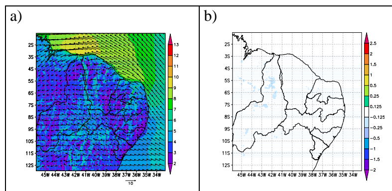
Figura 5.27 – (a) Média do campo de vento (m/s) a 10 m de altura das previsões de 24-48h para o período de 15 a 28 de setembro de 2005 do experimento Eta5L38 vegmod, (b) diferença entre a magnitude do vento médio dos experimentos Eta5L38 vegmod e controle.
