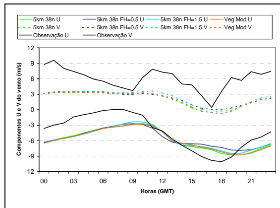
Figura 5.32 – Ciclo diário médio das componentes U (linha sólida) e V (linha tracejada) do vento (m/s) a 10 m de altura observado e previsto de 24-48h pelos experimentos controle (linha verde), Eta5L38 FH=0,5 (linha azul escura), Eta5L38 FH=1,5 (linha azul clara) e Eta5L38 vegmod (linha laranja) para Macau.
