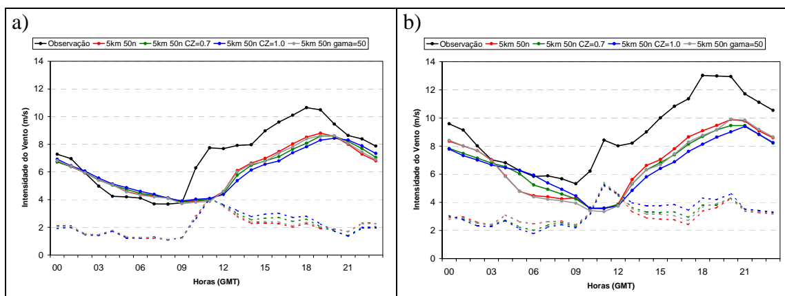
Figura 5.18 – Ciclo diário médio da velocidade do vento (m/s) (linha cheia) a (a) 10 m e (b) 50 m de altura observado e previsto de 24-48h pelos experimentos Eta5L50 (linha vermelha), Eta5L50 CZ=0,7 (linha verde), Eta5L50 CZ=1,0 (linha azul) e Eta5L50 \gamma=50 (linha cinza) para Macau. A linha tracejada indica o ciclo diário do RMSE para cada experimento.
