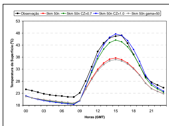
Figura 5.21 – Ciclo diário médio da temperatura da superfície ( ^{\circ}\text{C} ) observada e prevista de 24-48h pelos experimentos Eta5L50 (linha vermelha), Eta5L50 CZ=0,7 (linha verde), Eta5L50 CZ=1,0 (linha azul) e Eta5L50 \gamma=50 (linha cinza) para Macau.
