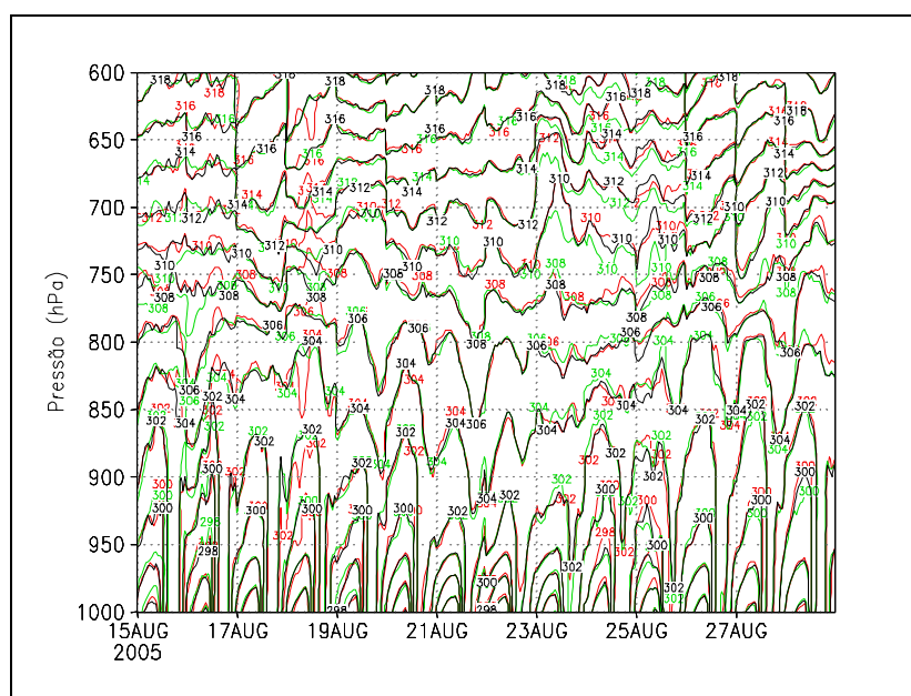
Figura 5.26 – Temperatura potencial (K) em Macau, prevista pelo C1 (linha preta) e pelo Eta5L38 FH=0,5 (linha vermelha) e pelo Eta5L38 FH=1,5 (linha verde), para o período de 15 a 28 de setembro de 2005.
