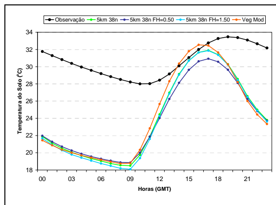
Figura 5.33 – Ciclo diário médio da temperatura do solo (°C) observada e prevista de 24-48h pelos experimentos controle (linha verde), Eta5L38 FH=0,5 (linha azul escura), Eta5L38 FH=1,5 (linha azul clara) e Eta5L38 vegmod (linha laranja) para Macau.
