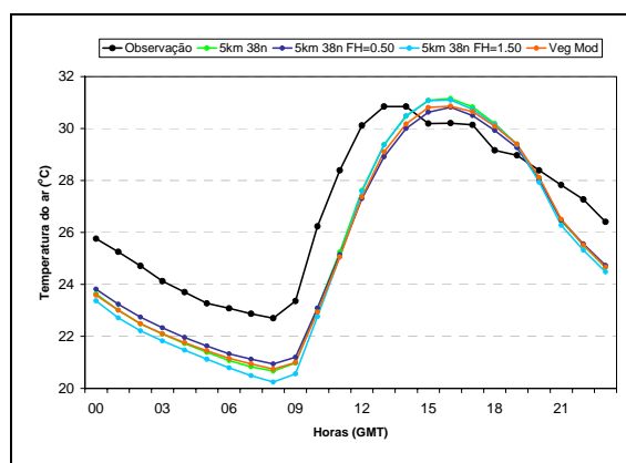
Figura 5.35 – Ciclo diário médio da temperatura do ar ( ^{\circ}\text{C} ) a 2 m de altura observada e prevista de 24-48h pelos experimentos controle (linha verde), Eta5L38 FH=0,5 (linha azul escura), Eta5L38 FH=1,5 (linha azul clara) e Eta5L38 vegmod (linha laranja) para Macau.
