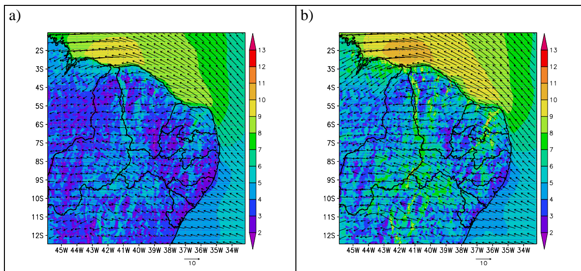
Figura 5.1 – Média da velocidade do vento (m/s) a: (a) 10 m de altura e (b) 50 m de altura para o experimento controle. Os campos médios se referem as previsões de 24-48h para o período de 15 a 28 de setembro de 2005.
