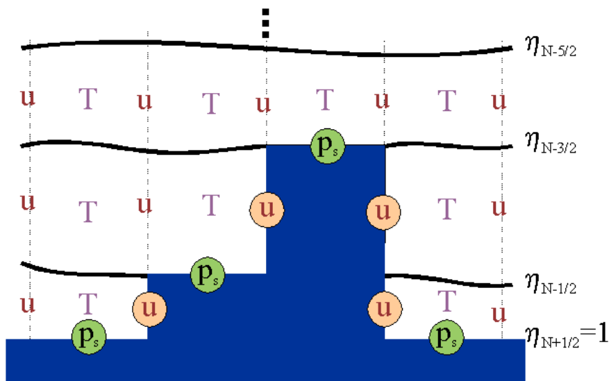
Figura 4.6 – Seção vertical idealizado da topografia do modelo Eta e distribuição das variáveis na vertical (u, T, Ps).
