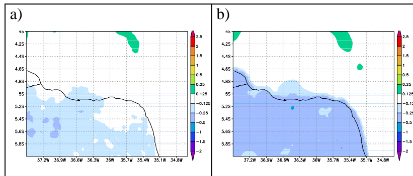
Figura 5.29 – Diferença entre a magnitude do vento médio a (a) 10 m e (b) 50 m de altura as 1500 GMT dos experimentos Eta5L38 vegmod e controle.
