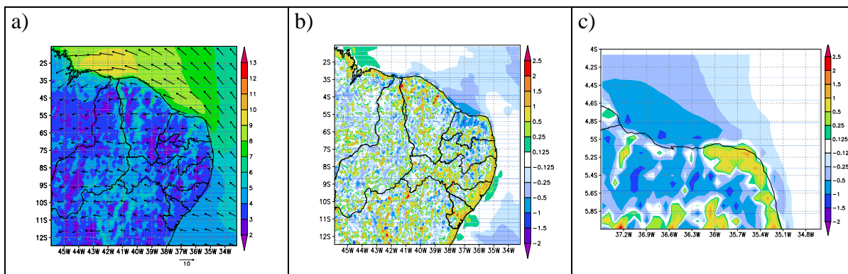
Figura 5.4 – (a) Média do campo de vento (m/s) a 10 m de altura das previsões de 24-48h para o período de 15 a 28 de setembro de 2005 do experimento Eta10L38, (b) diferença entre a magnitude do vento médio dos experimentos controle e Eta10L38 e (c) detalhe sobre RN.
