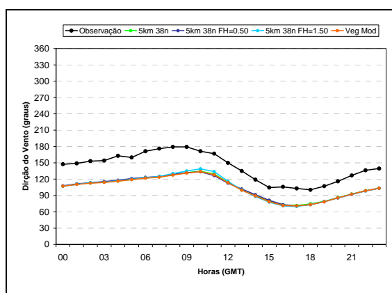
Figura 5.31 – Ciclo diário médio da direção do vento (graus) observado a 20,5 m de altura e previsto de 24-48h a 10 m de altura pelos experimentos controle (linha verde), Eta5L38 FH=0,5 (linha azul escura), Eta5L38 FH=1,5 (linha azul clara) e Eta5L38 vegmod (linha laranja) para Macau.
