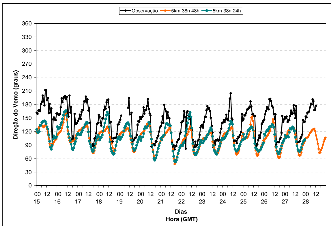
Figura 5.3 – Série temporal da direção do vento a 20,5 m de altura (graus) simulada para as 24 horas (linha azul) e 48 horas (linha laranja) de integração no experimento controle e observada (linha preta) em Macau.
