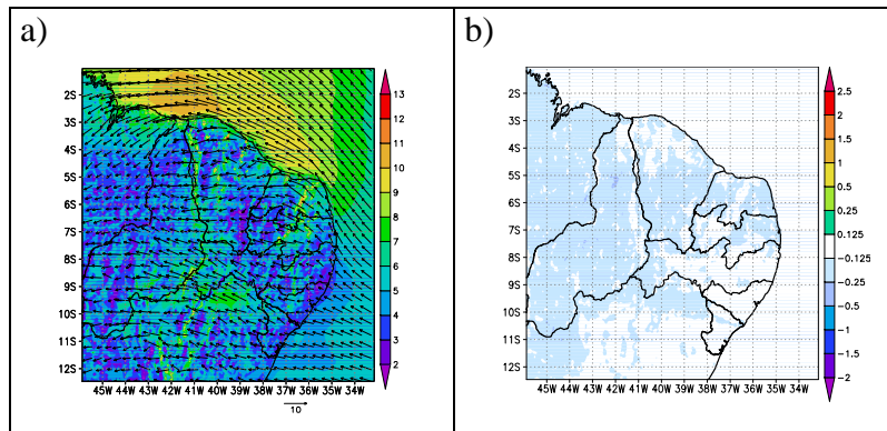
Figura 5.17 – (a) Média do campo de vento (m/s) a 50 m de altura das previsões de 24-48h para o período de 15 a 28 de setembro de 2005 do experimento Eta5L50 \gamma=50 , (b) diferença entre a magnitude do vento médio dos experimentos Eta5L50 \gamma=50 e controle.
