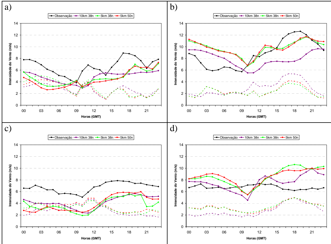
Figura 5.12 – Ciclo diário médio da velocidade do vento (m/s) (linha cheia) a 50 m de altura observado e previsto de 24-48h pelos experimentos controle (linha verde), Eta10L38 (linha roxa) e Eta5L50 (linha vermelha) para (a) Canto do Amaro, (b) Mínhoto, (c) Pacatuba e (d) Alcântara. A linha tracejada indica o ciclo diário do RMSE para cada experimento.
