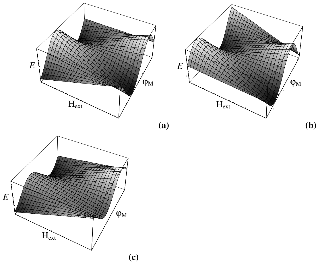
Figura 6: Gráficos da energia em função do campo H_{\text{ex}} e do ângulo \phi_M . Para o cálculo foi utilizado \theta_M = 90^\circ , M_s = 1200 \text{ emu/cm}^3 , K_1 = 500 \text{ ergs/cm}^3 e (a) \theta_H = 90^\circ e \phi_H = 90^\circ . (b) \theta_H = 90^\circ e \phi_H = 30^\circ . Para uma configuração onde o campo magnético é aplicado fora do plano do filme temos que: (c) \theta_H = 45^\circ e \phi_H = 90^\circ
