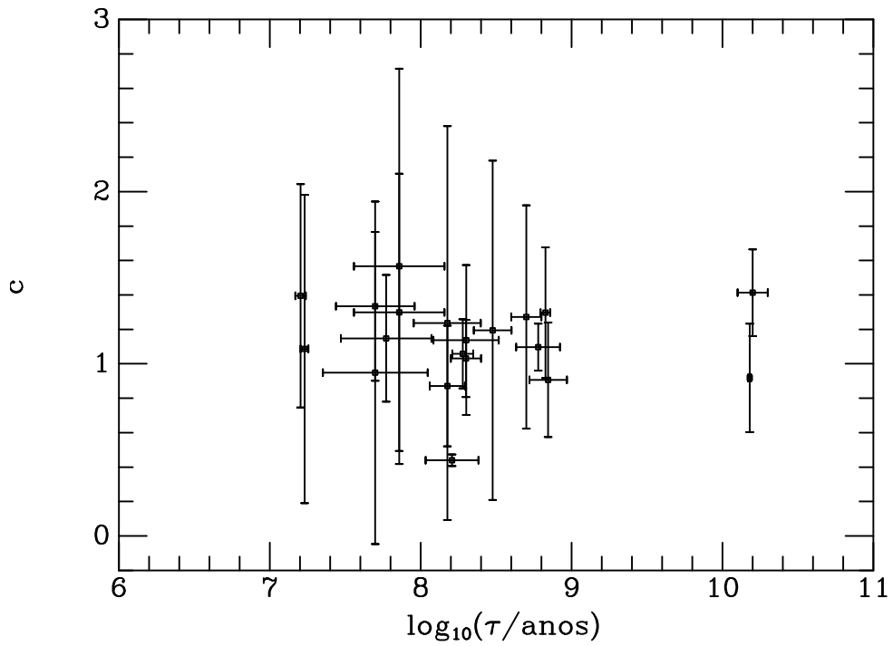
Figura 4.35: Parâmetro de concentração obtido neste trabalho contra a idade encontrada na literatura. Os dois pontos deslocados à direita correspondem aos aglomerados NGC 2210 e [H60b] 11.
