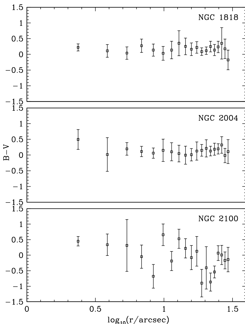
Figura 4.31: Perfis da cor B-V para os aglomerados NGC 1818, NGC 2004 e NGC 2100. Não é possível identificar gradientes de cor em nenhum deles, talvez devido ao seeing muito alto, a baixa resolução das imagens utilizadas neste trabalho, e a contaminação por estrelas de campo.
