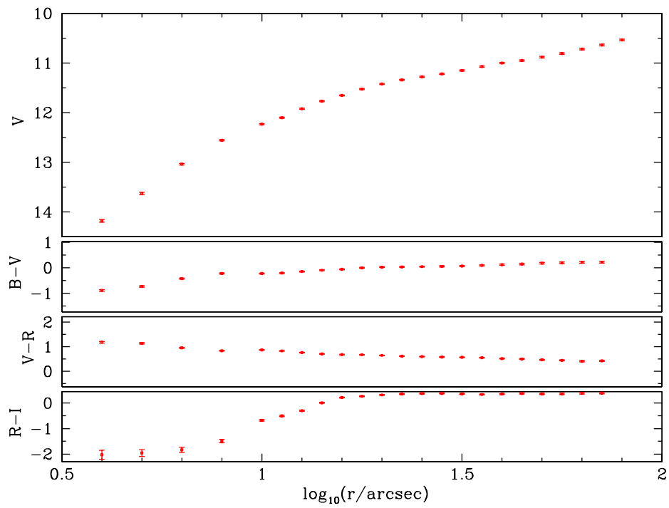
Figura 4.19: Brilho superficial e integrado para o aglomerado NGC 1847 apresentados da mesma maneira que a figura 4.1.
