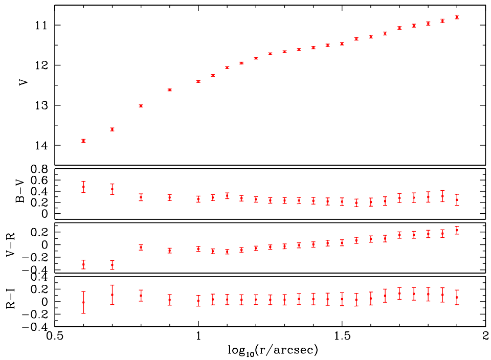
Figura 4.9: Brilho superficial e integrado para o aglomerado Lindsay 72 apresentados da mesma maneira que a figura 4.1.
