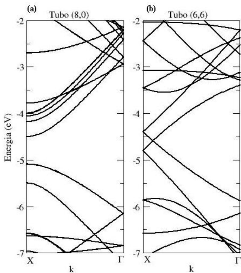
Figura 12: Estrutura de bandas de nanotubos (a) zigzag (8,0) semicondutor e (b) armchair (6,6) metálico.
