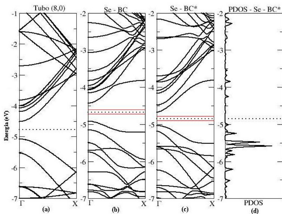
Figura 25: Estrutura de bandas e densidade de estados projetadas (PDOS) no átomo de Se. As linhas pontilhadas correspondem as energias de Fermi.
