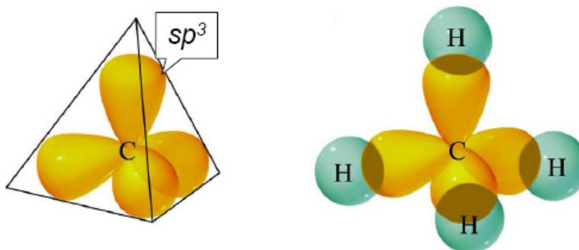
Figura 1: Orbitais híbridos sp^3 formando ligações \sigma . A direita temos o exemplo da molécula do metano (adaptado de [6]).
