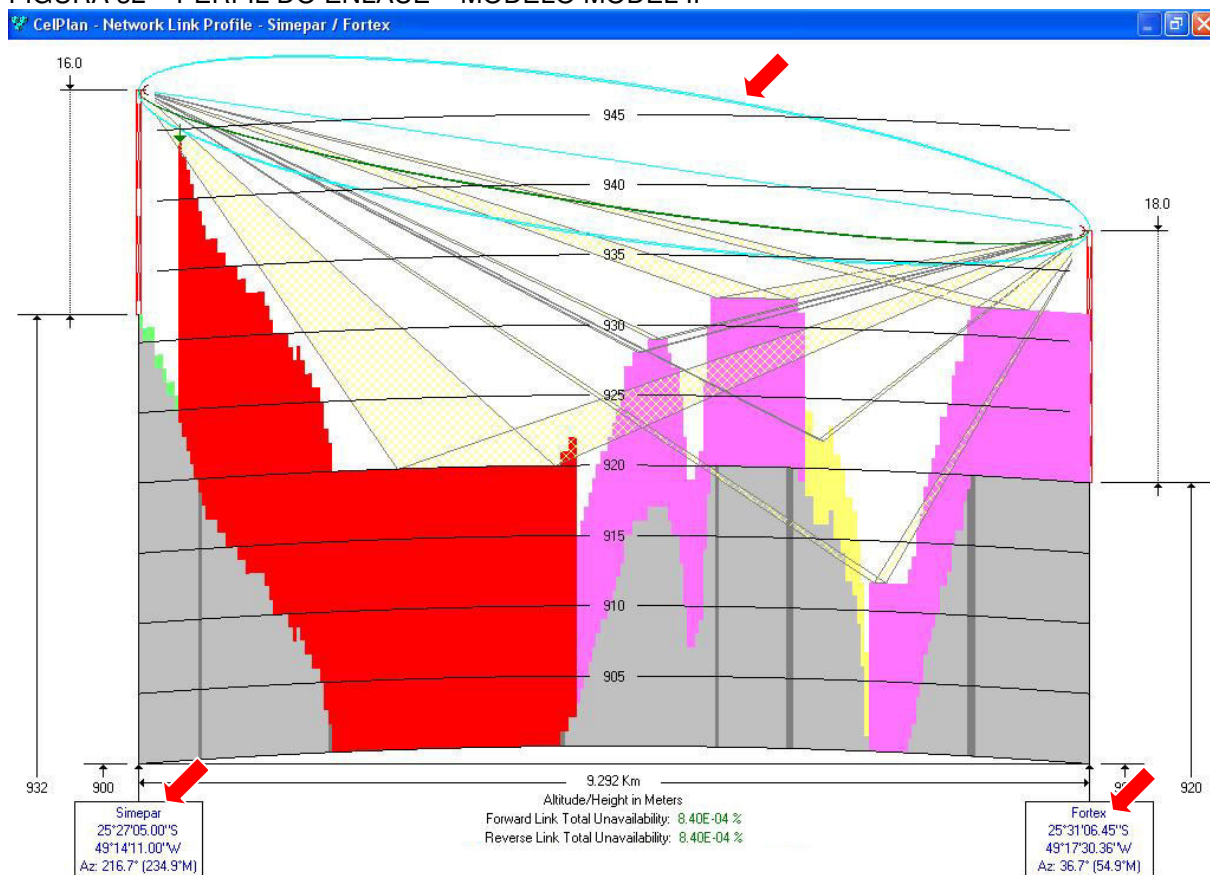
FIGURA 32 – PERFIL DO ENLACE – MODELO MODEL II
