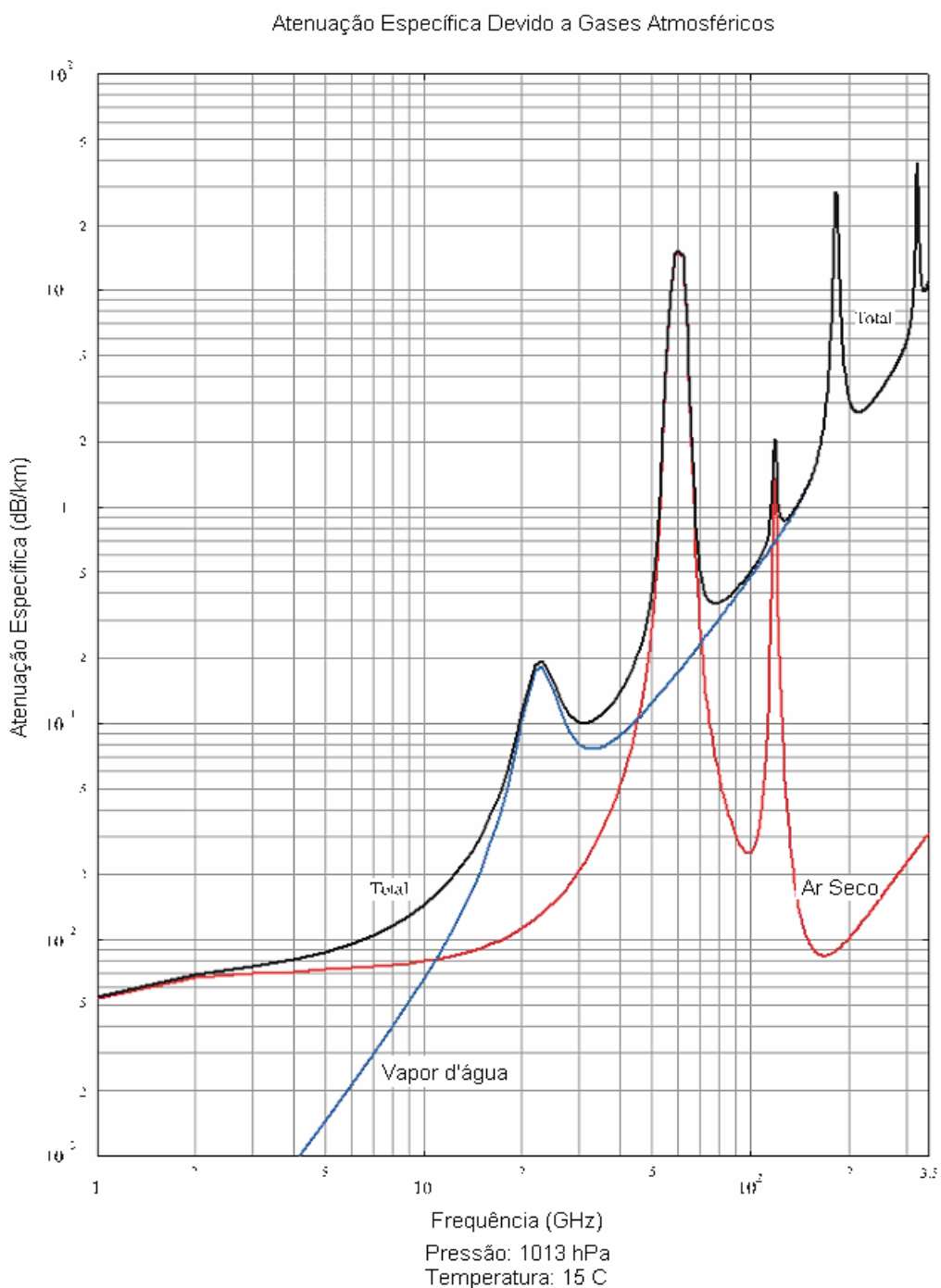
FIGURA 05 – ATENUAÇÃO ESPECÍFICA DEVIDO A GASES ATMOSFÉRICOS
