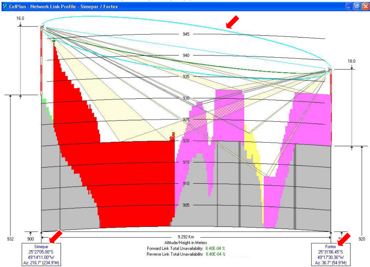
FIGURA 30 – PERFIL DO ENLACE – MODELO LOS
