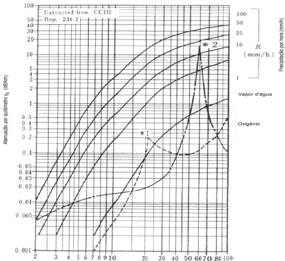
FIGURA 2 – ATENUAÇÃO DEVIDO À CHUVA VERSUS PRECIPITAÇÃO HORÁRIA Atenuação devido ao Oxigênio, Vapor d'água e Chuva
