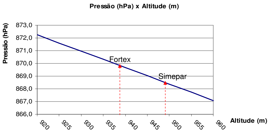
FIGURA 23 – VARIAÇÃO DA PRESSÃO ATMOSFÉRICA EM FUNÇÃO DA ALTITUDE
