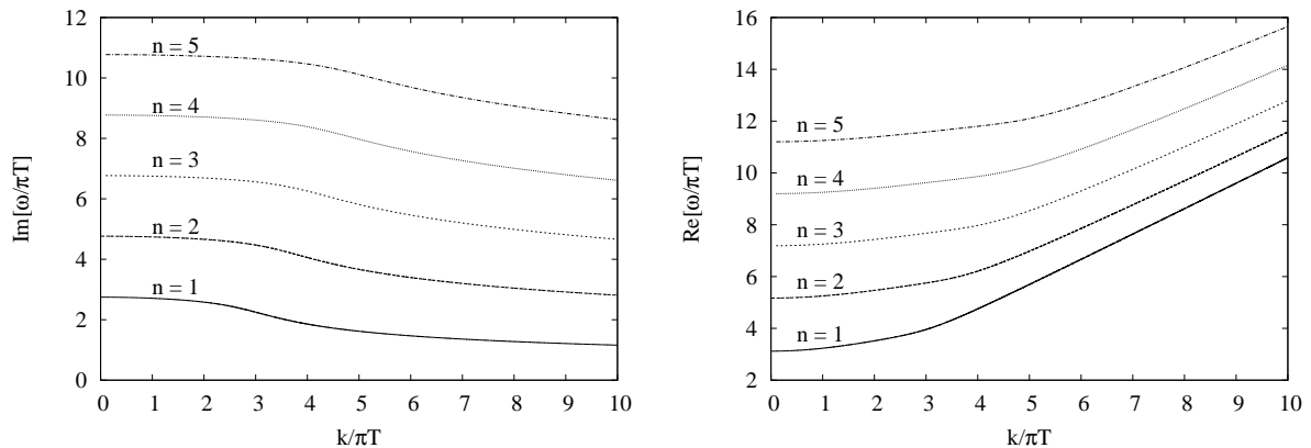
Figura 5.5: Relações de dispersão para modos vetoriais em cinco dimensões.
