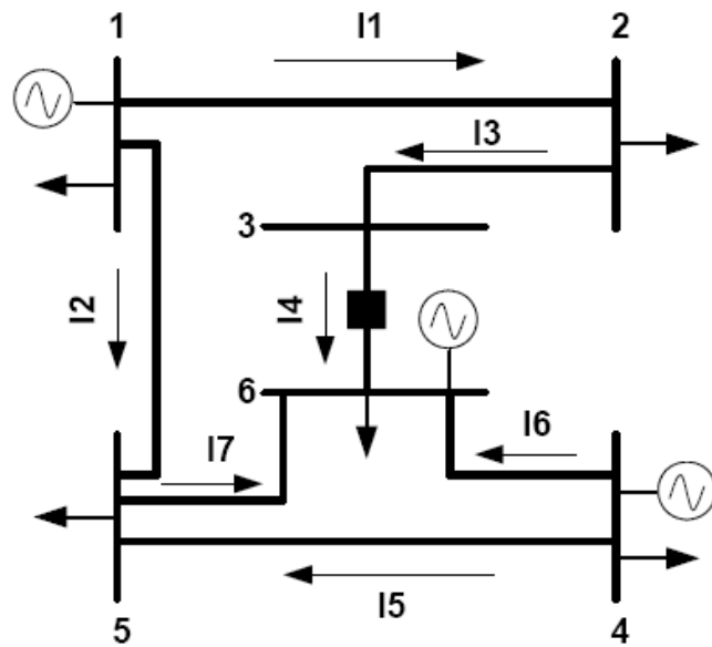
FIGURA 5 – MODELO DE SEP (NSE) FLUXOS DE POTÊNCIA
