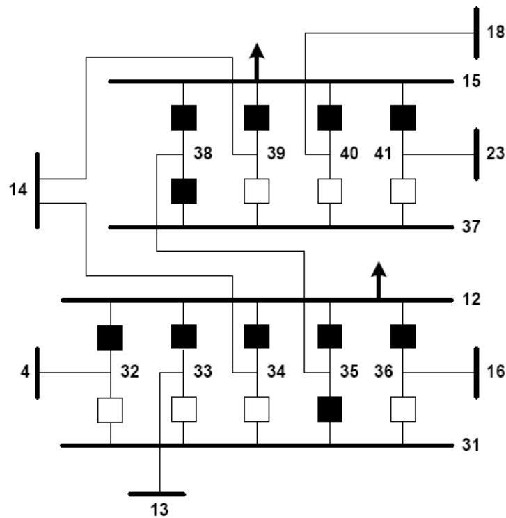
FIGURA 9 - SEP 41 BARRAS MODELAGEM NÍVEL DE SUBESTAÇÃO
