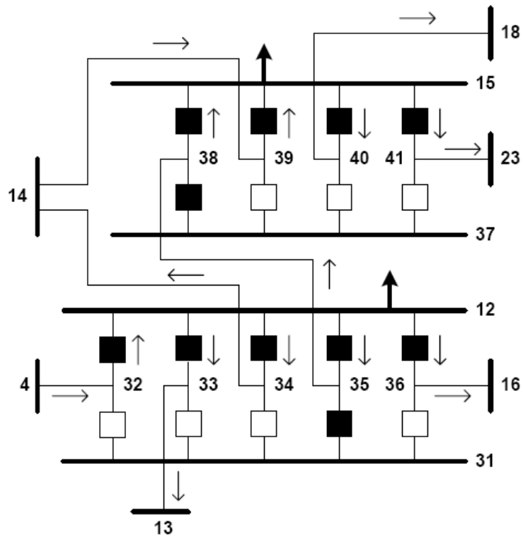
FIGURA 11 - SEP 41 BARRAS MODELAGEM NSE – FLUXOS DE POTÊNCIA
