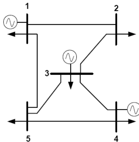
FIGURA 3 – MODELO DE SEP (MODELAGEM BARRA-RAMO)
