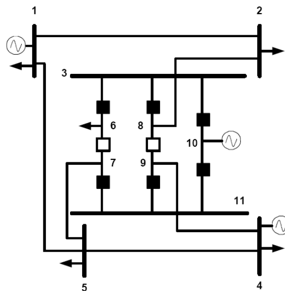
FIGURA 7 - SEP 11 BARRAS MODELAGEM NÍVEL DE SUBESTAÇÃO
