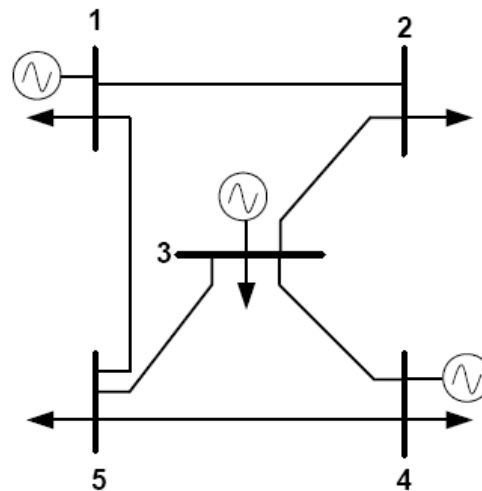
FIGURA 6 – DIAGRAMA UNIFILAR SEP 5 BARRAS
