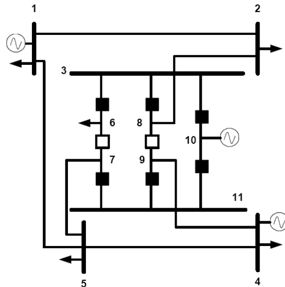
FIGURA 2 – EXEMPLO DE MODELAGEM NO NÍVEL DE SUBESTAÇÃO
