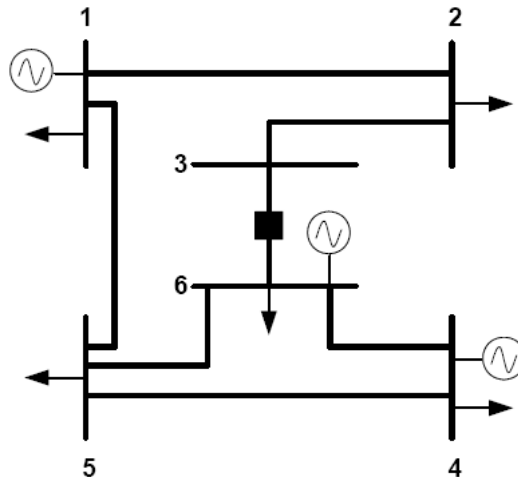
FIGURA 4 – MODELO DE SEP (MODELAGEM NÍVEL DE SUBESTAÇÃO)
