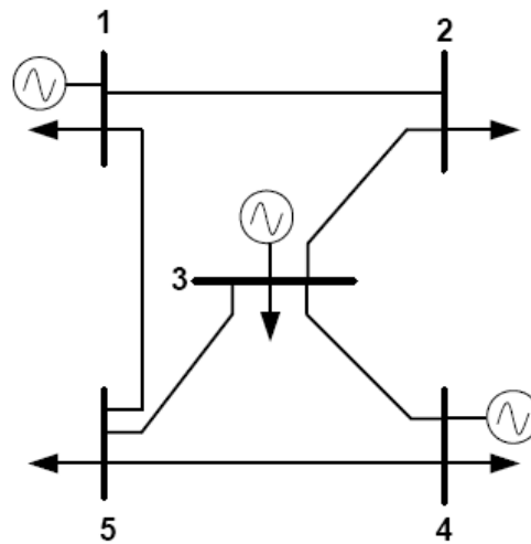
FIGURA 1 – EXEMPLO DE MODELAGEM BARRA-RAMO
