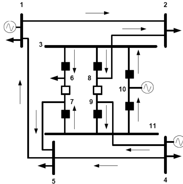
FIGURA 10 - SEP 11 BARRAS MODELAGEM NSE – FLUXOS DE POTÊNCIA
