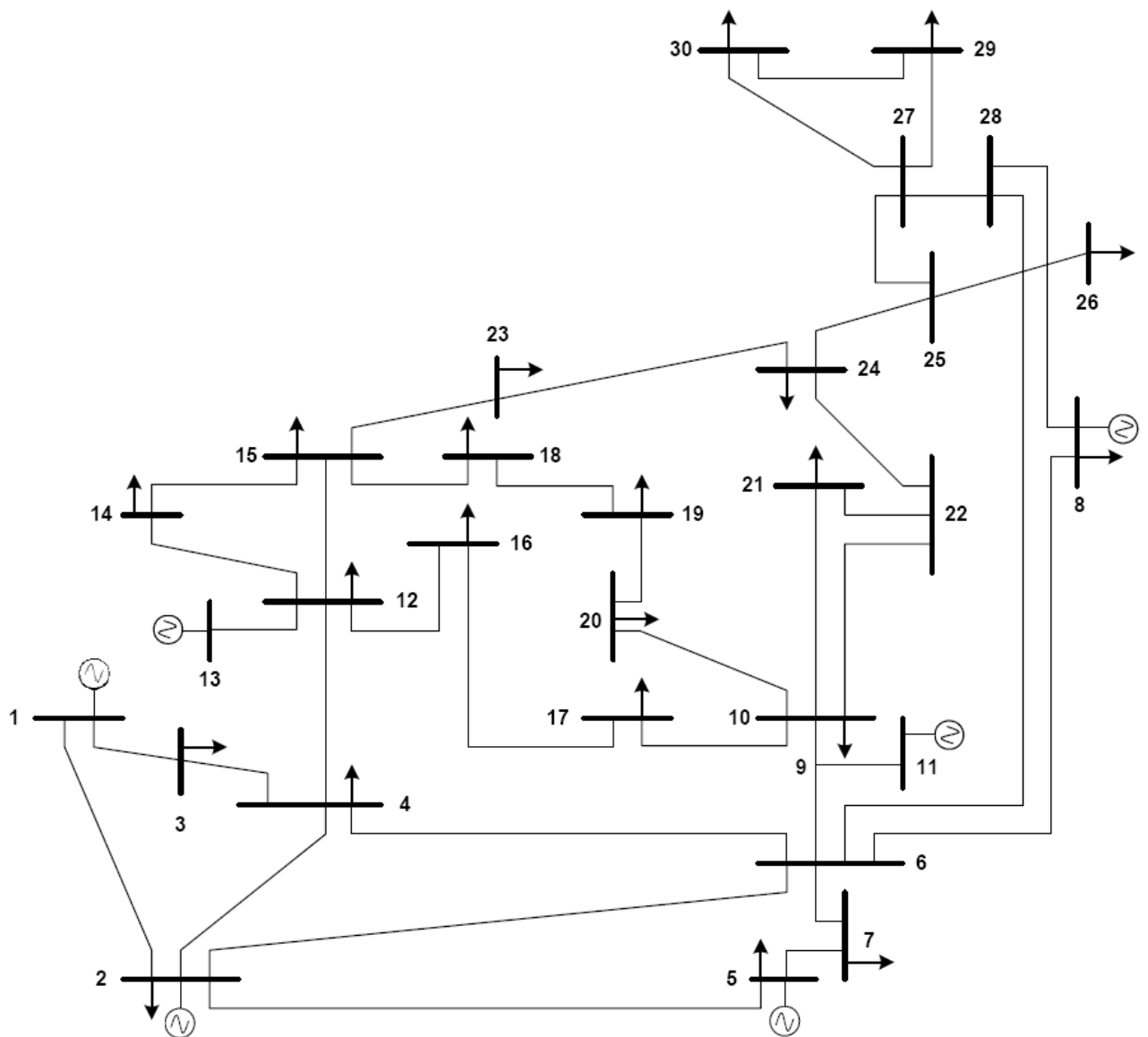
FIGURA 8 – DIAGRAMA UNIFILAR SEP IEEE 30 BARRAS
