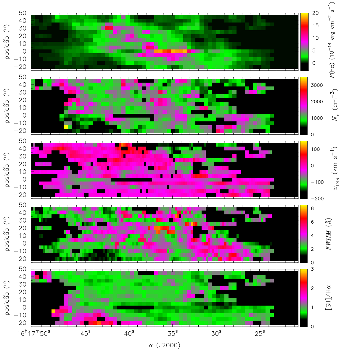
Figura 3.8: Mapas finais das propriedades físicas de RCW 103. O primeiro mapa, de cima para baixo, é o dos fluxos da linha H \alpha ; o segundo, o mapa da densidade eletrônica; o terceiro, o mapa da velocidade radial LSR; o quarto é o mapa da largura de H \alpha a meia altura; e, por fim, o quinto deles é o mapa da razão [SII]/H \alpha . Em cada um dos mapas o eixo horizontal indica a ascensão reta e, o vertical, a declinação em relação à estrela de referência. Para a esquerda, aponta a direção Leste, e, para cima, a direção Norte.
