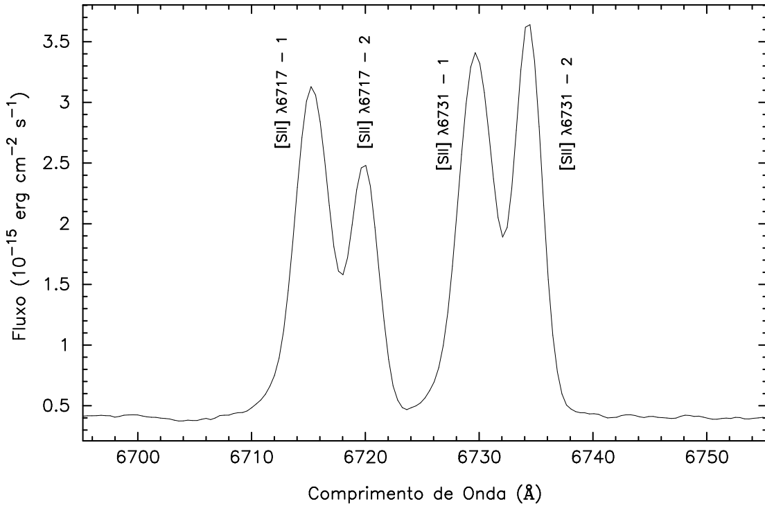
Figura 3.2: Espectro de emissão de RCW 103 evidenciando as duas componentes das linhas do duplete [SII] \lambda\lambda 6717,6731 e a grande variação de densidade entre as componentes 1 e 2. Esse é o espectro obtido com a fenda orientada sobre a estrela de referência e correspondente à abertura de número 23.
