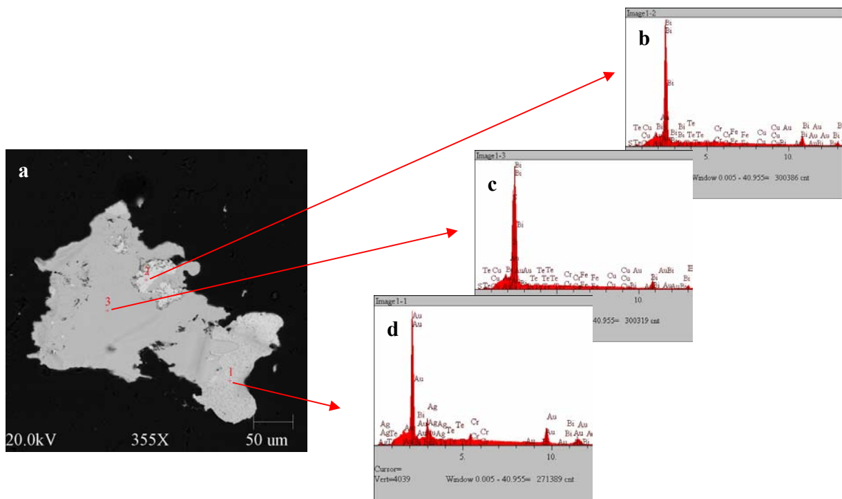
Figura 74: a-Imagem de elétrons retroespalhados, obtida em MEV, de cristal de ouro associado à bismutinita e bismuto nativo. b- Espectrograma EDS do Bi nativo mostrando os picos do Bi. c- Espectrograma EDS da bismutinita mostrando os picos do S e Bi. d- Espectrograma EDS do ouro mostrando os picos do Au.
