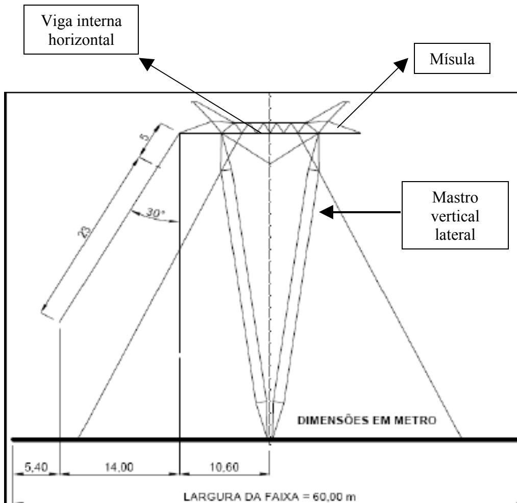
Figura 3 – Largura da faixa de servidão onde é implantada a torre. As setas assinalam os locais típicos de posicionamento de ninhos sobre as torres: viga interna horizontal, mísula e dois masts verticais laterais.
