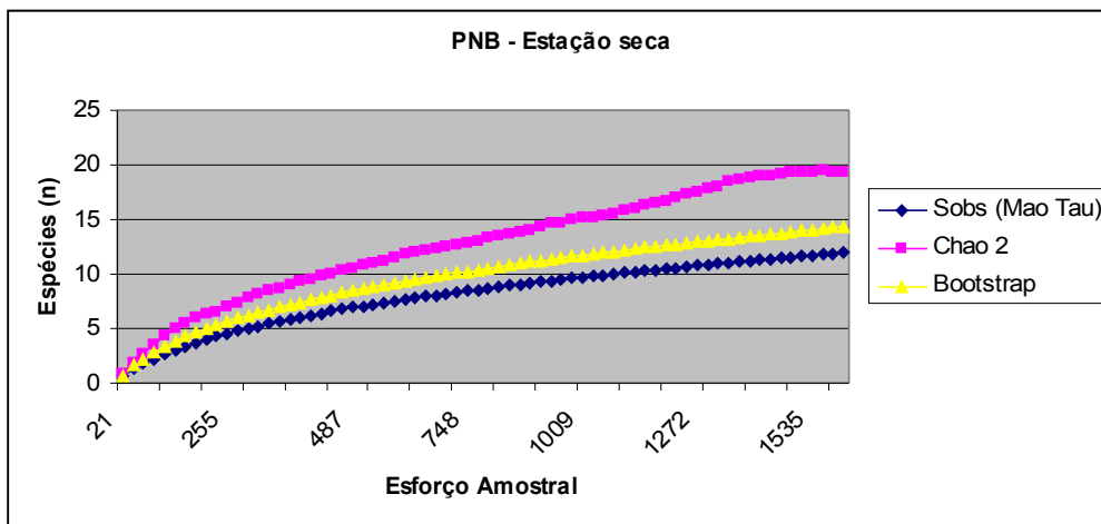
Figura 7 – Curvas de acumulação de espécies (Sobs – Mao Tau) e curvas obtidas pelos métodos não-paramétricos (Bootstrap, Chao 2, Jack 1 e Jack 2) relativas ao levantamento na estação seca, no PNB
