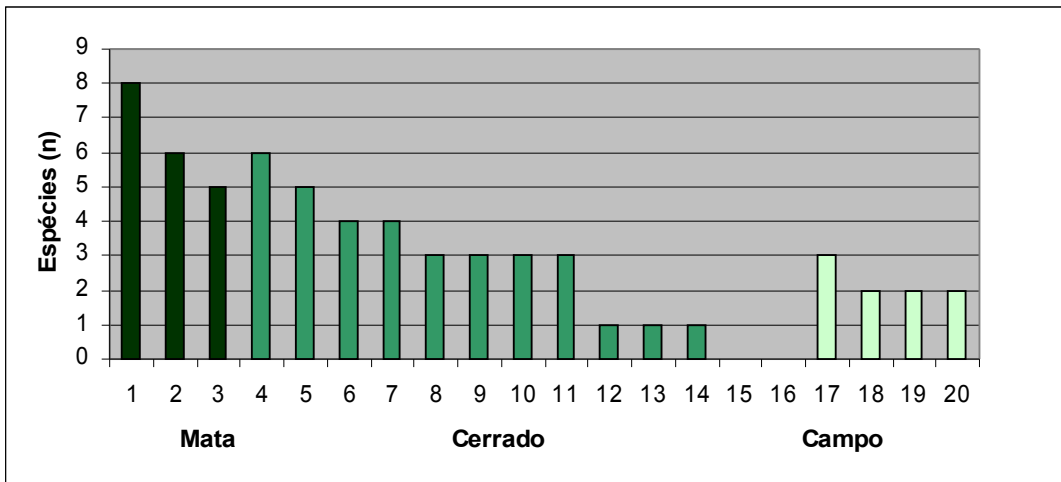
Figura 5 – Número de espécies fotografadas por ponto de amostragem na ESECAE (verde escuro na classe Mata; verde na classe Cerrado e verde claro na classe Campo), pontos 15 e 16 localizados em áreas de cerrado.
