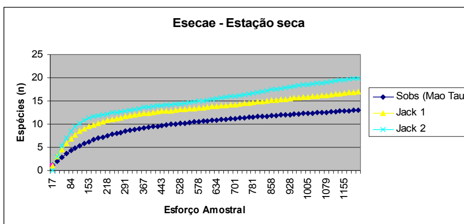
Figura 3 – Curvas de acumulação de espécies (Sobs – Mao Tau) relativas aos levantamentos nas estações seca e chuvosa, e curvas obtidas pelos métodos não-paramétricos (Bootstrap, Chao 2, Jack 1 e Jack 2) relativas ao levantamento na estação seca, na ESECAE.
