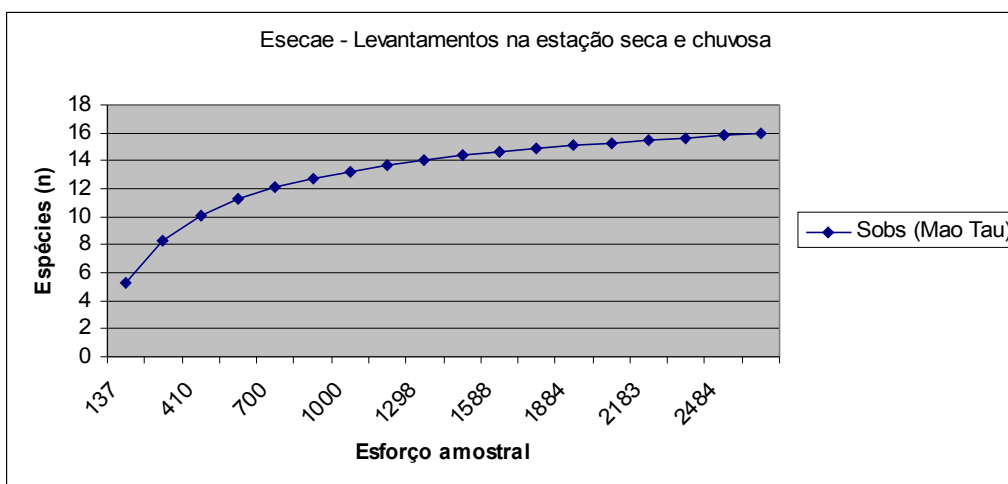
Figura 4 – Curva de acumulação de espécies (Sobs – Mao Tau) relativa aos dois levantamentos realizados na ESECAE, durante as estações seca e chuvosa.
