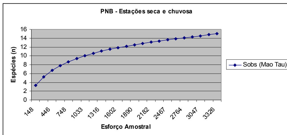
Figura 8 – Curva de acumulação de espécies (Sobs – Mao Tau) relativa a dois levantamentos realizados no Parque Nacional de Brasília, durante as estações seca e chuvosa.
