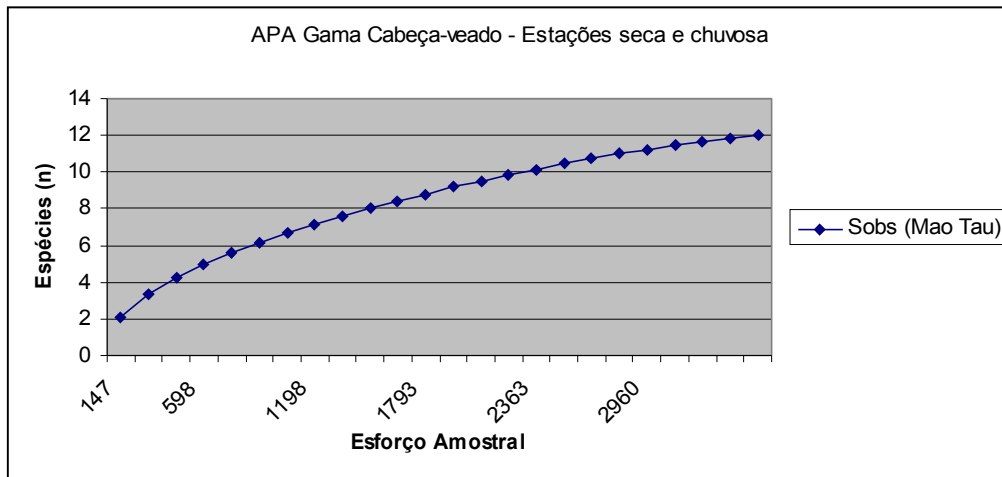
Figura 6 – Curva de acumulação de espécies (Sobs – Mao Tau) relativa a dois levantamentos realizados na APA GCV, durante as estações seca e chuvosa.
