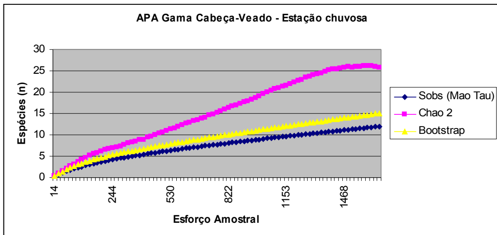
Figura 5 – Curvas de acumulação de espécies (Sobs – Mao Tau) relativas aos levantamentos nas estações seca e chuvosa, e curvas obtidas pelos métodos não-paramétricos (Bootstrap, Chao 2, Jack 1 e Jack 2) relativas ao levantamento na estação chuvosa, na APA GCV.
