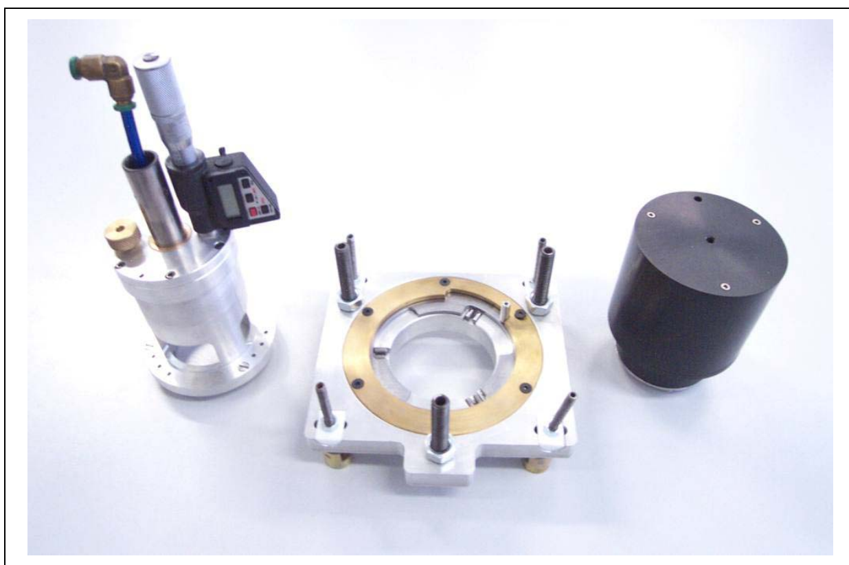
Figura 5.2 MTRES Modular ou M2TRES - Dispositivo para medição de tensões mecânicas e tensões residuais por holografia eletrônica.
