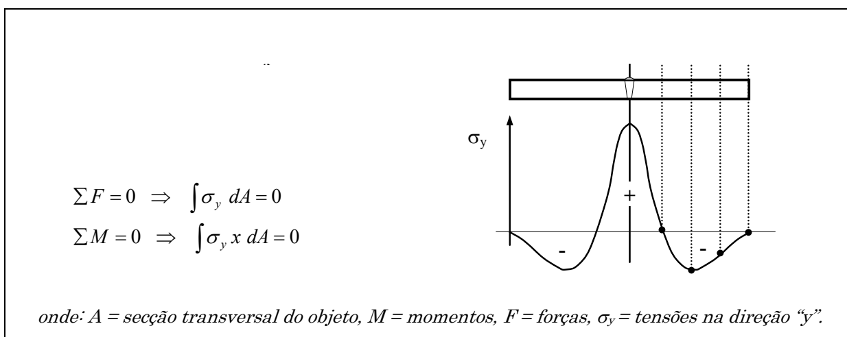
Figura 2.1 Esquema do comportamento das tensões residuais nas proximidades de união por soldagem de chapas [73] .
