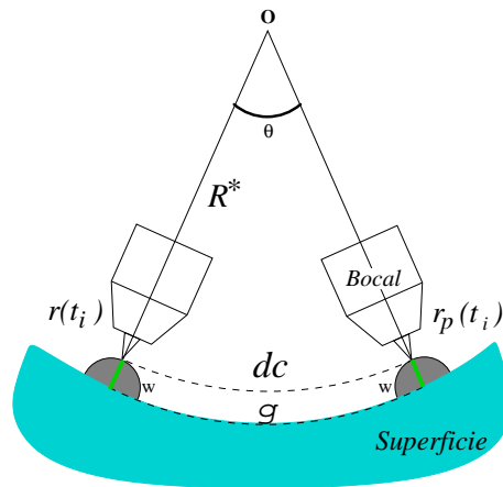
Figura 2.11: Obtenção de g para uma superfície com curvatura positiva.
