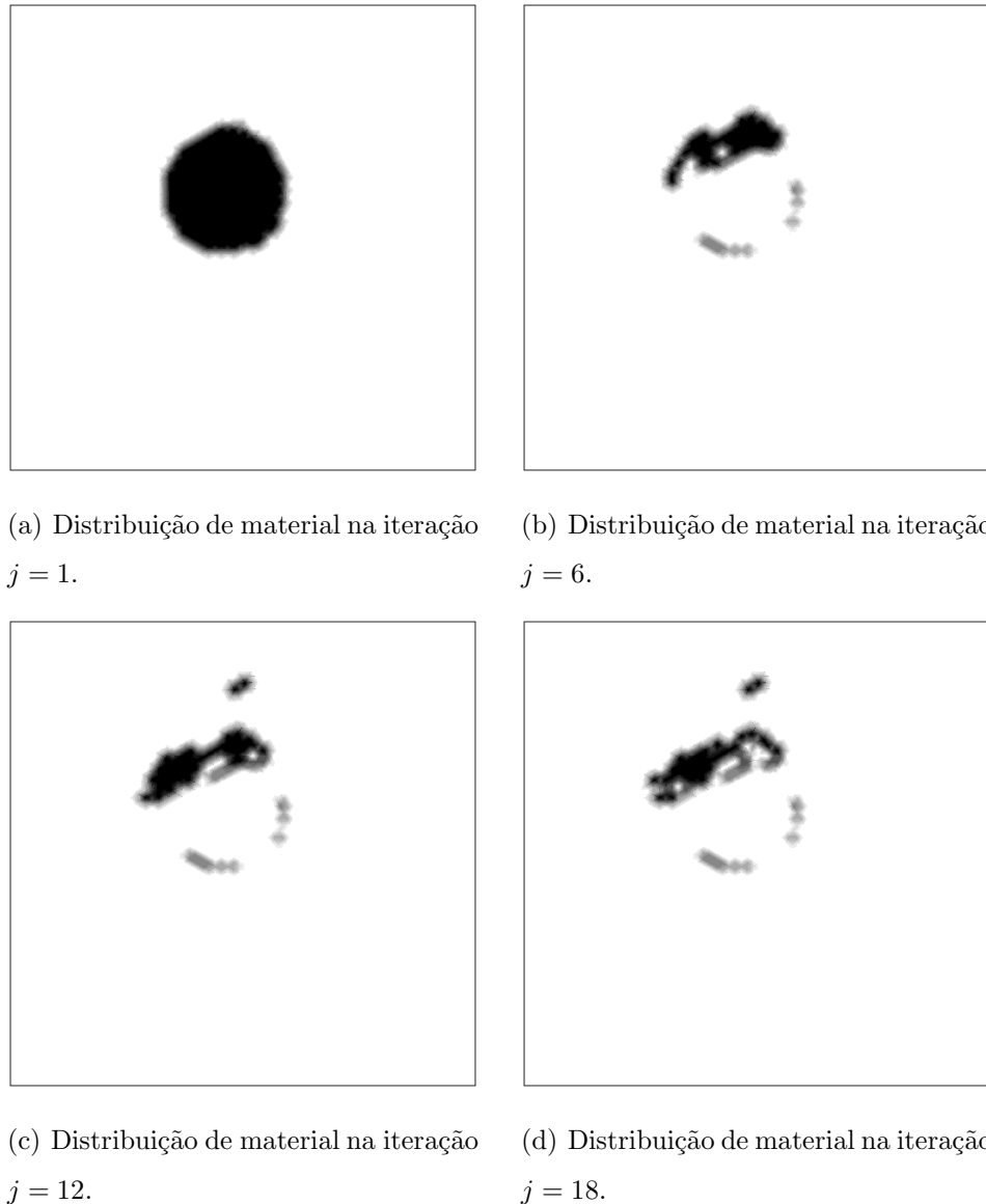
Figura 5.26: Exemplo 4 - Distribuição de material obtida para as iterações j = 1, 6, 12, 18 .
