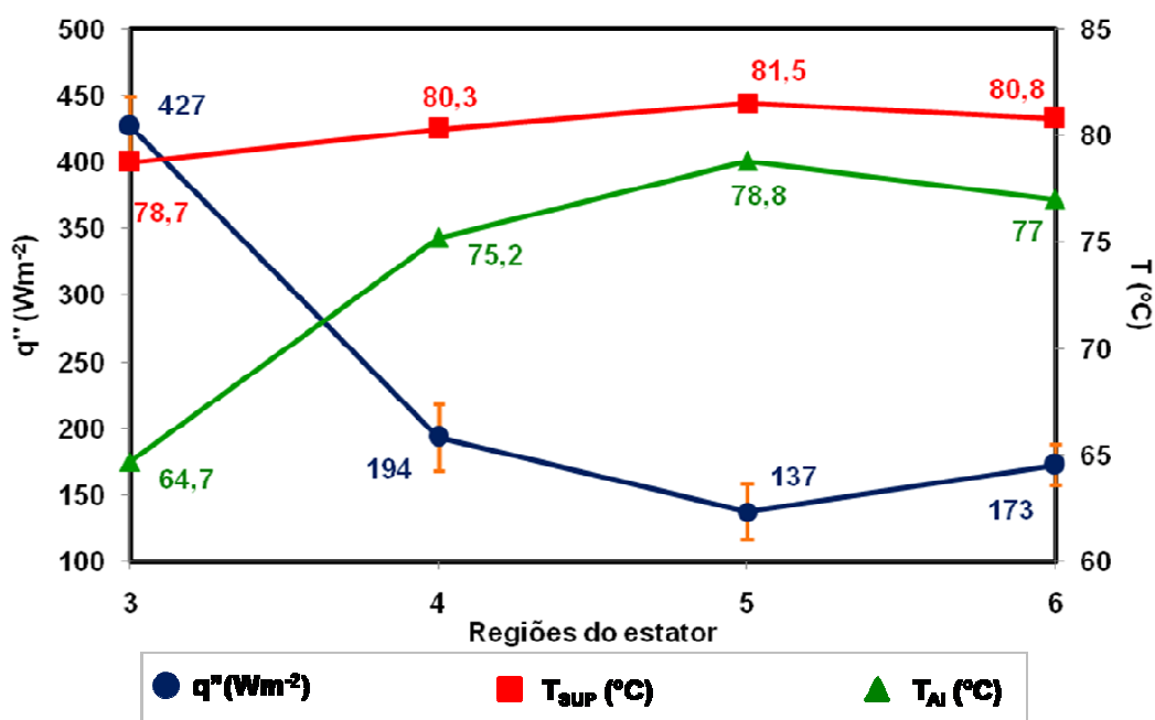
Figura 6.22 - Fluxo de calor e potenciais de temperatura no estator.
