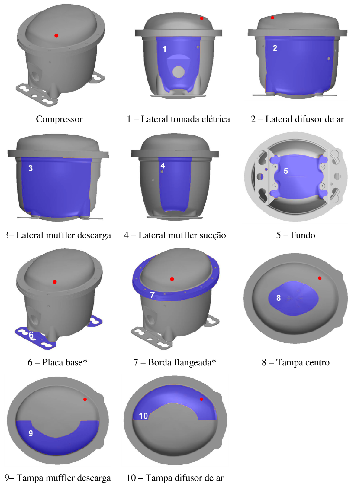
Figura 5.2 – Parede externa da carcaça do compressor dividida em regiões. A marcação feita nestas imagens, e nas demais que serão exibidas adiante, atua como referência para melhor entendimento das rotações aplicadas a cada vista do compressor.
