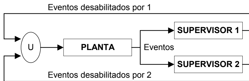
Figura 3.7 - Esquema de controle modular (QUEIROZ e CURY, 2000).
