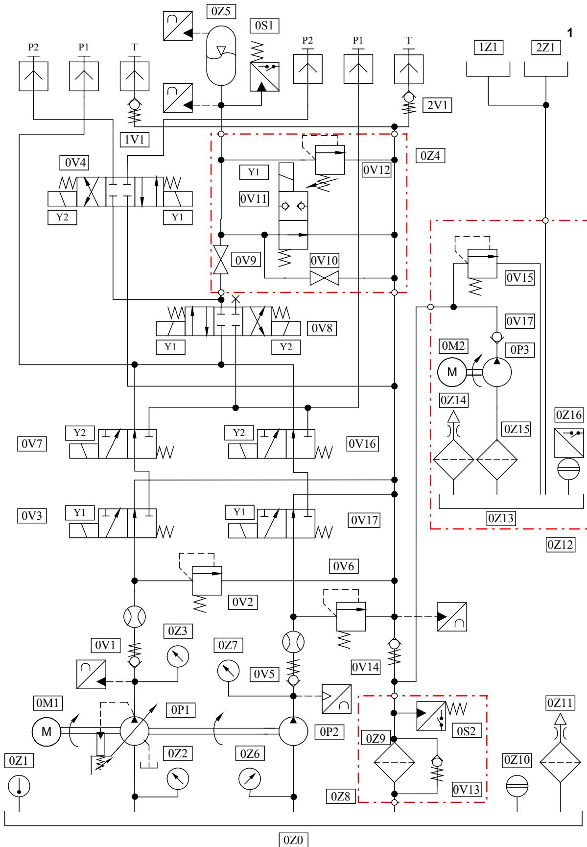
Figura 8.2 - Circuito hidráulico da unidade de potência.
