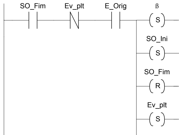
Figura 6.10 - Diagrama escada para implementação de transição não controlável - Autolaço (self-loop).
