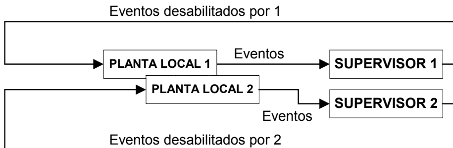
Figura 3.10 - Esquema de controle modular local (QUEIROZ e CURY, 2000).
