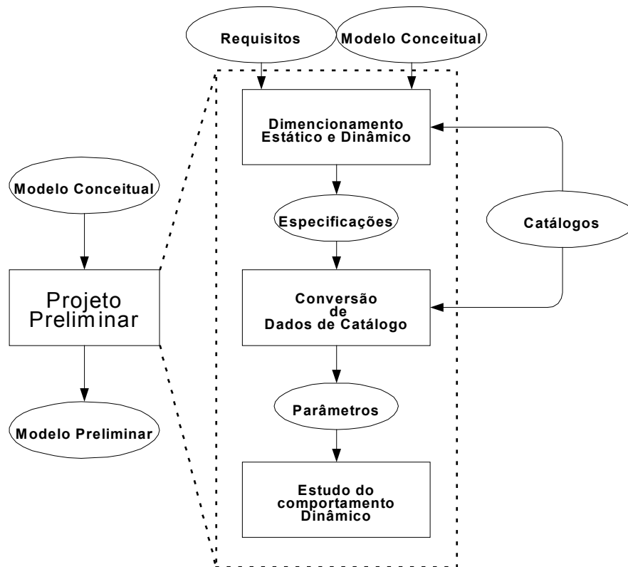
Figura 2.13 - Etapas do projeto preliminar de sistemas hidráulicos de controle de posição (FURST e DE NEGRI, 2002).
