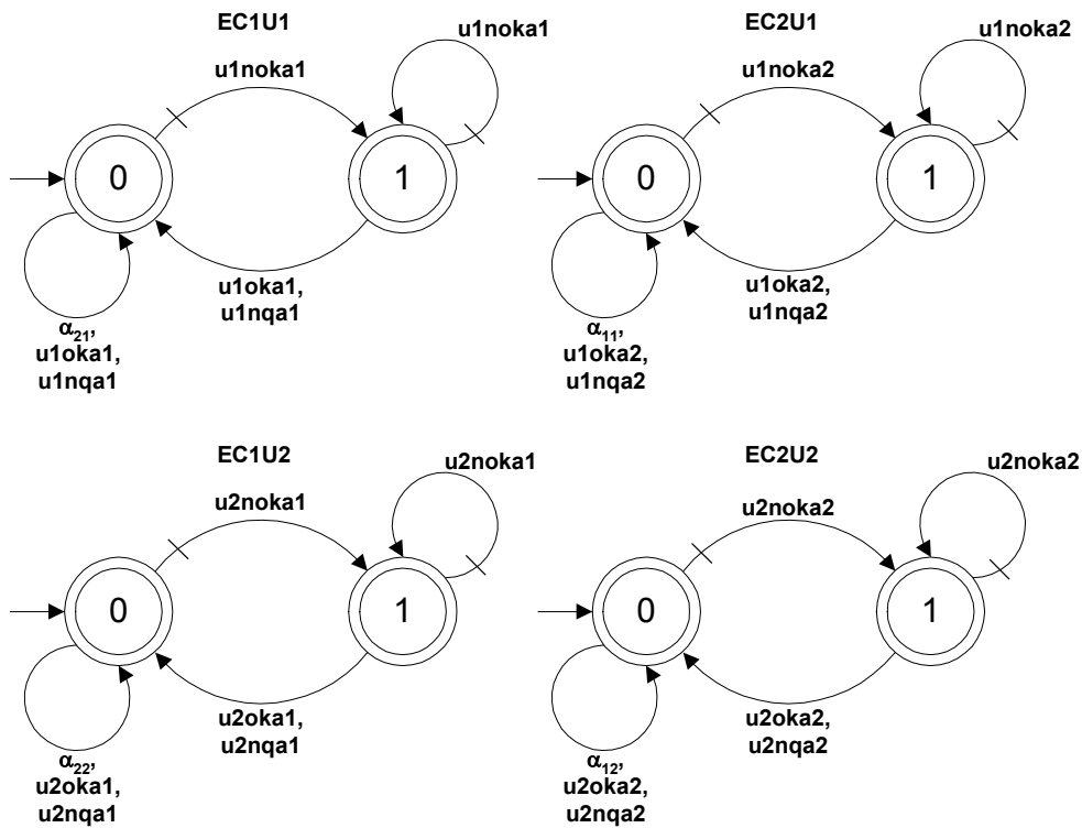
Figura 7.18 - Especificações complementares para evitar acionamento parcial.
