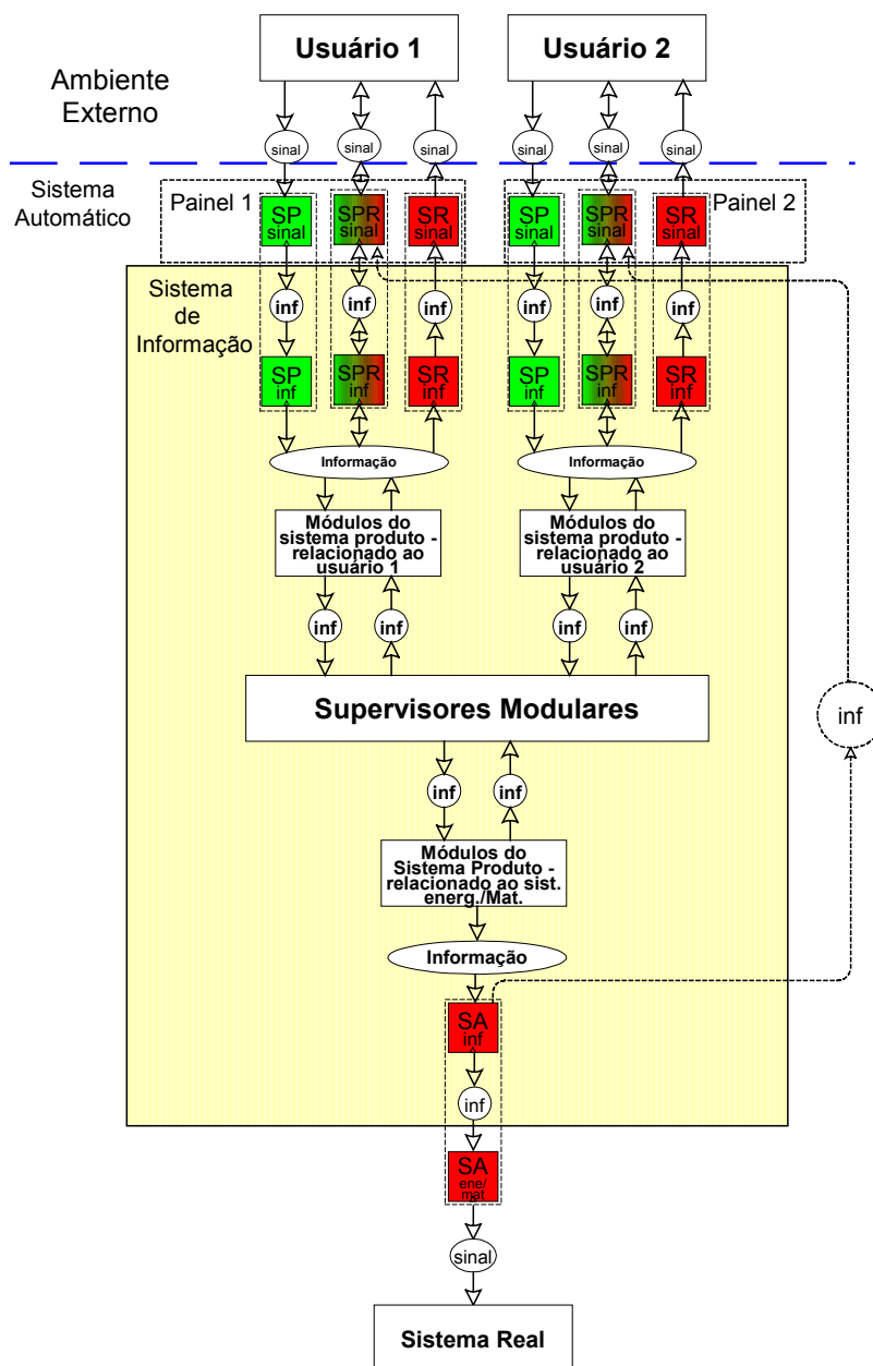
Figura 7.12 - C/A do sistema de informação do projeto teste.
