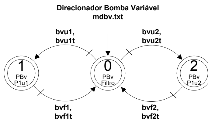
Figura 8.8 - Autômato do direcionador da bomba variável.
