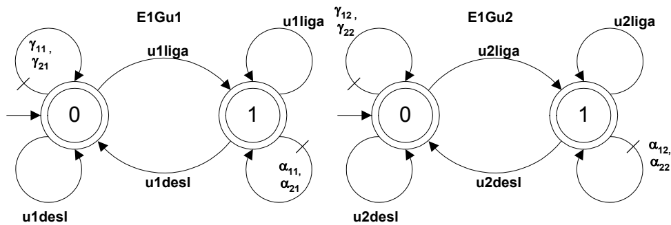
Figura 7.11 - Especificações de acionamento de Ag1 e Ag2, relativas aos comandos de ligar dos usuários.
