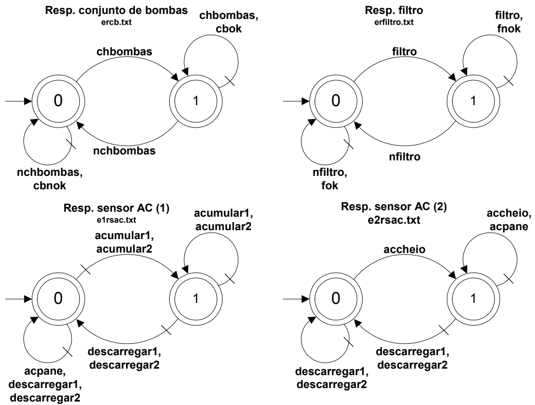
Figura 8.23 - Especificações para a resposta de erros críticos.
