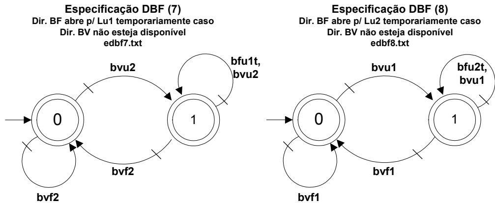
Figura 8.14 - Especificação para preferência de BV no enchimento do acumulador.
