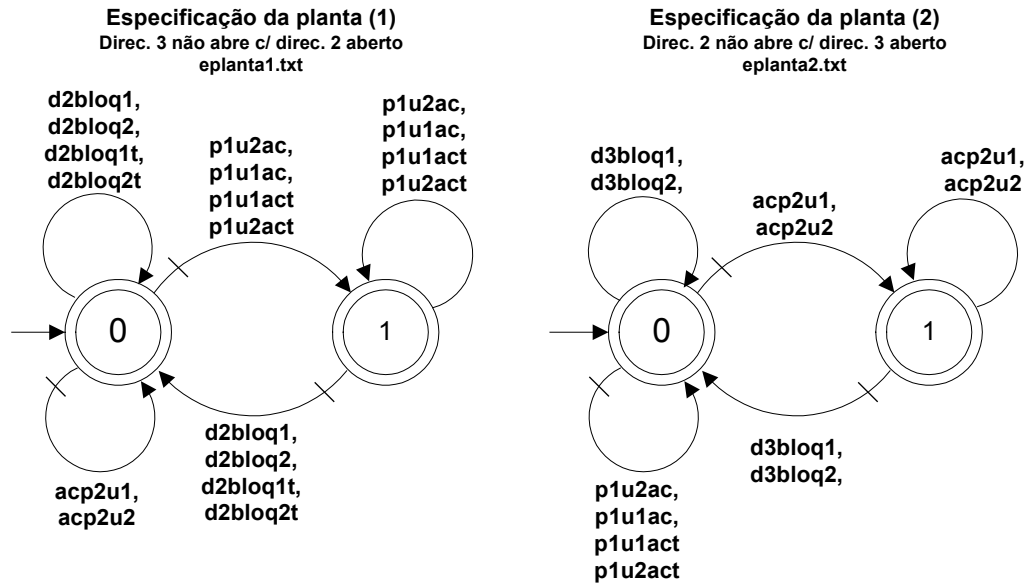
Figura 8.13 - Especificações da planta sem a comunicação com o ambiente externo.
