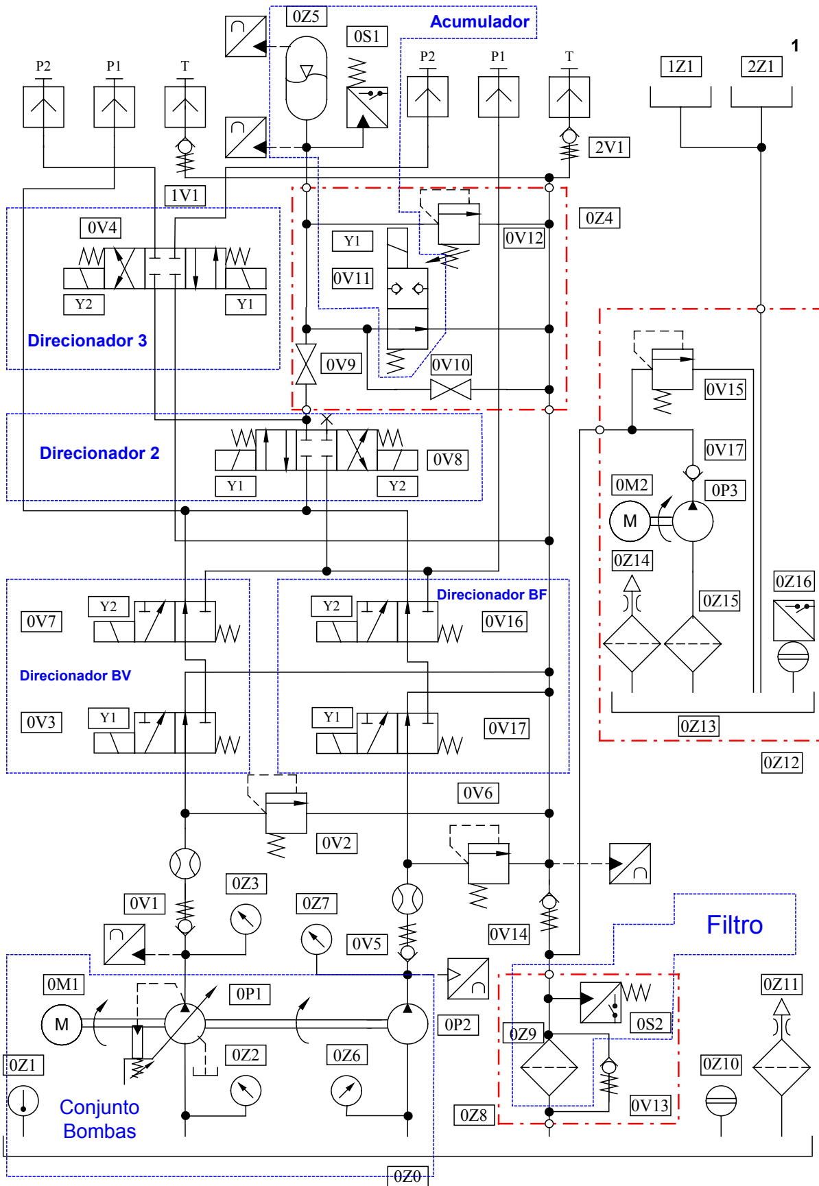
Figura 8.5 - Entidade do circuito hidráulico importantes ao controle.
