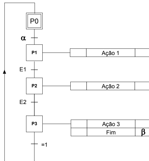
Figura 3.12 - Sequência operacional modelada através de um SFC.
