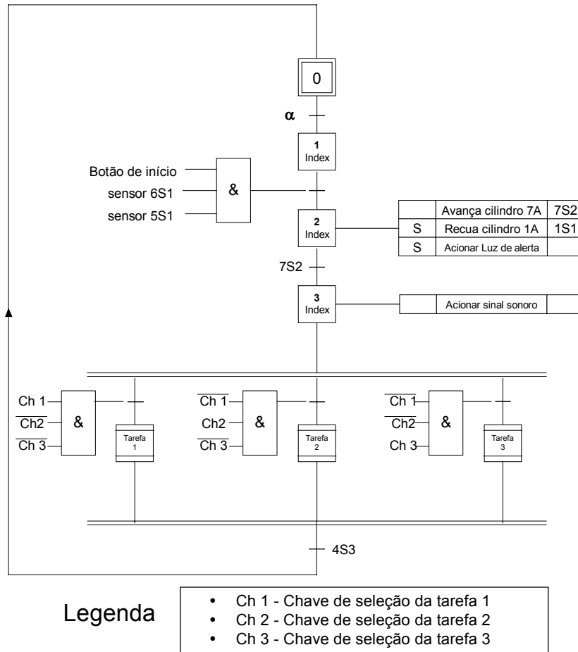
Figura 5.3 – Exemplo de seqüência operacional implementada em diagrama de funcionamento (SFC) – Entradas e saídas ao ambiente externo.
