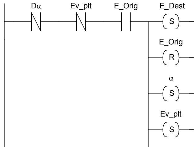
Figura 6.11 - Diagrama escada para implementação de transição controlável.
