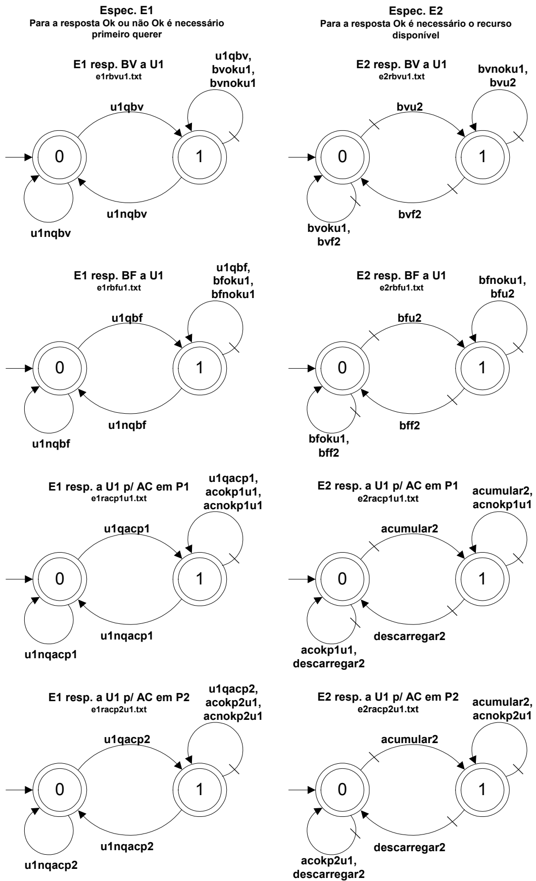
Figura 8.21 - Especificações das respostas de BV, BF e AC.
