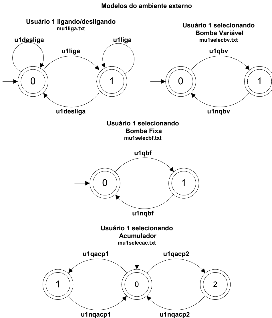
Figura 8.18 - Modelos dos pedidos do usuário 1.
