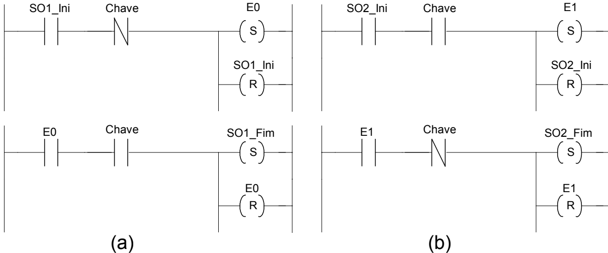
Figura 6.13 - Diagrama escada da interface de entrada de uma chave comum.
