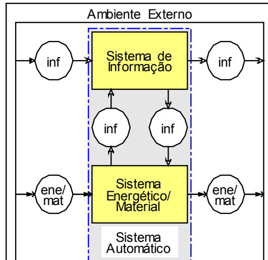
Figura 5.2 - Modelo funcional/estrutural condensado de um sistema automático.
