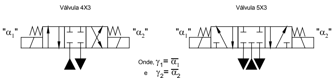
Figura 7.9 - Princípios de solução para Ag1' .
