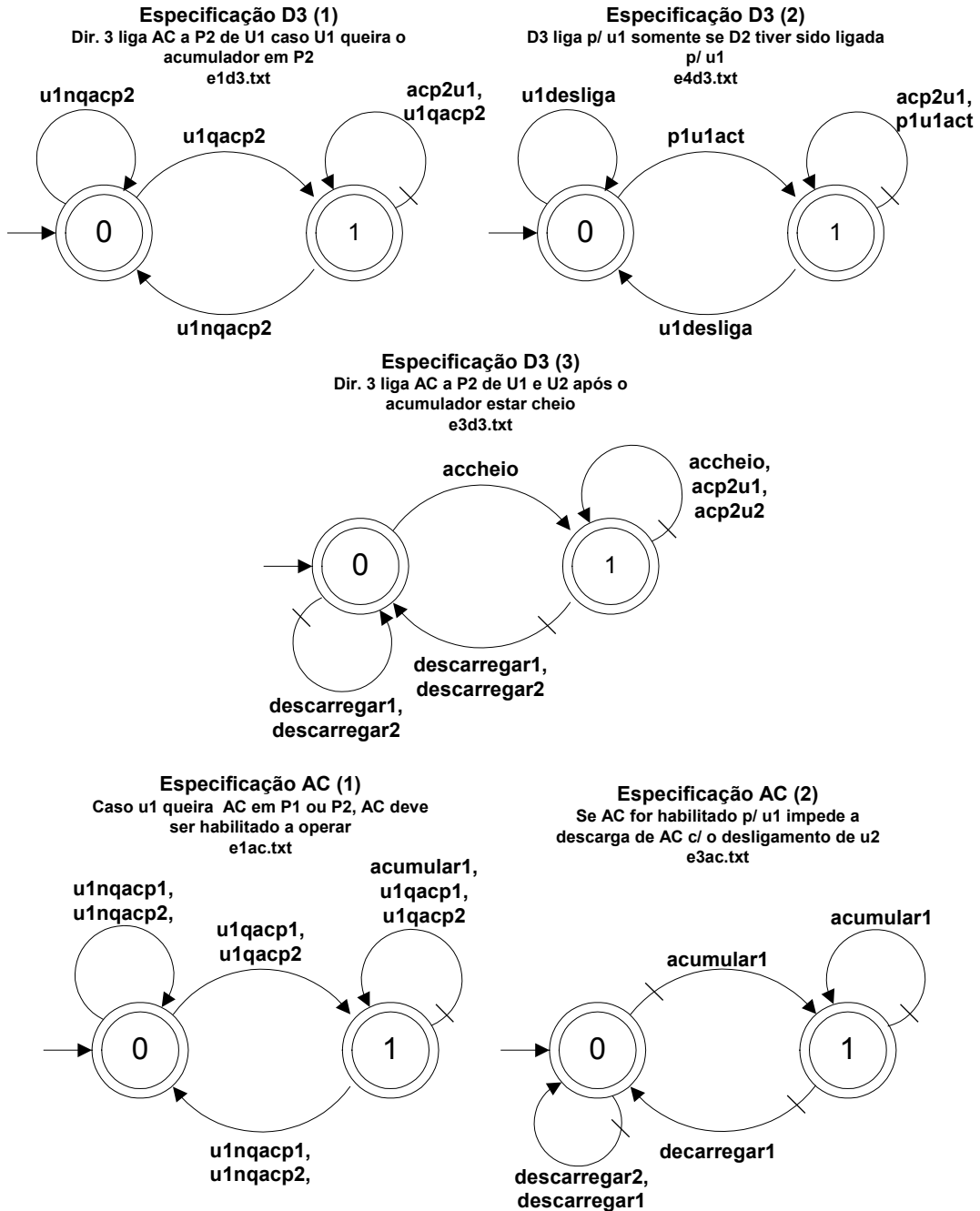
Figura 8.17 - Especificação do direcionador 3 e do acumulador.
