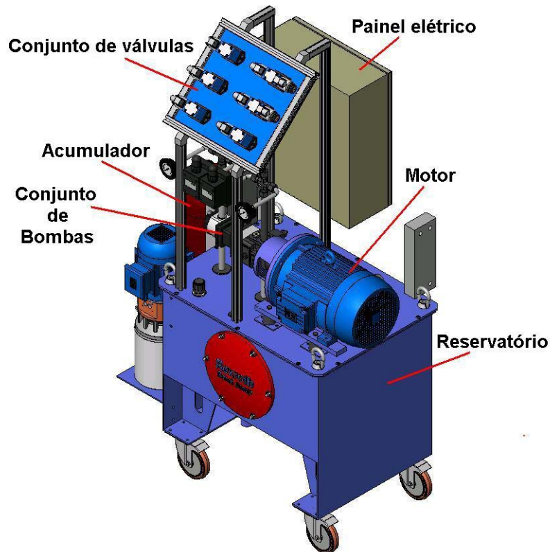
Figura 8.1 - Desenho da unidade hidráulica de potência.
