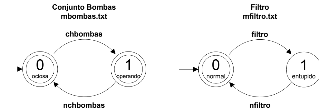
Figura 8.7 - Autômatos do conjunto de bombas e do filtro.
