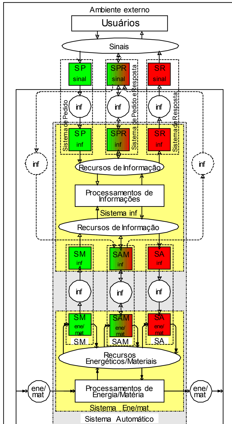
Figura 5.7 – Modelo estrutural e funcional de um sistema automático estendido – caso de um usuário.
