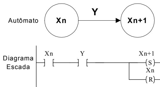
Figura 3.13 - Estrutura de interpretação de um Autômato em Diagrama Escada.
