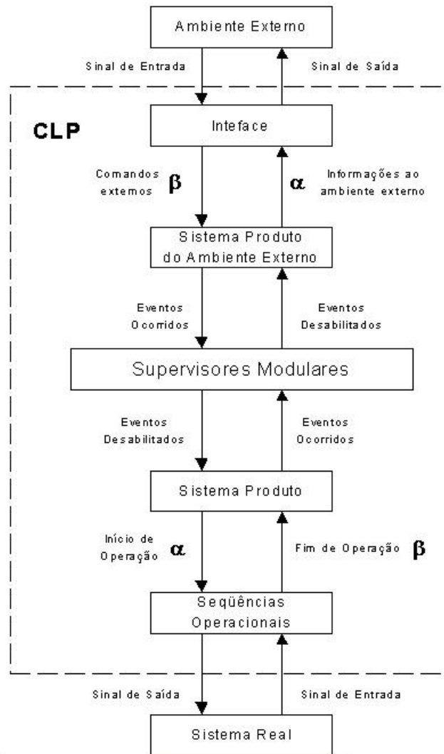
Figura 5.8 – Diagrama de blocos da estrutura de controle estendida ao ambiente externo.
