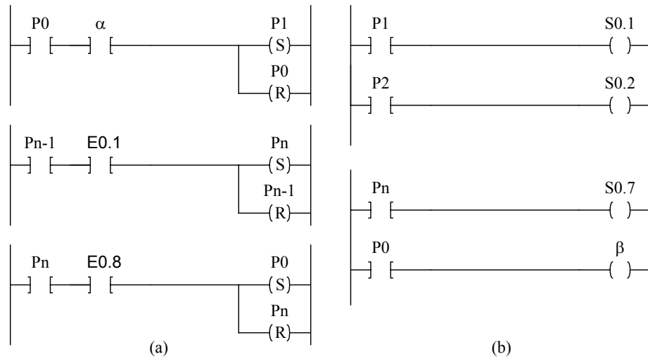
Figura 3.17 - Exemplo de diagrama escada de uma seqüência operacional onde, (a) – Bloco de passos e (b) - Bloco de saídas.
