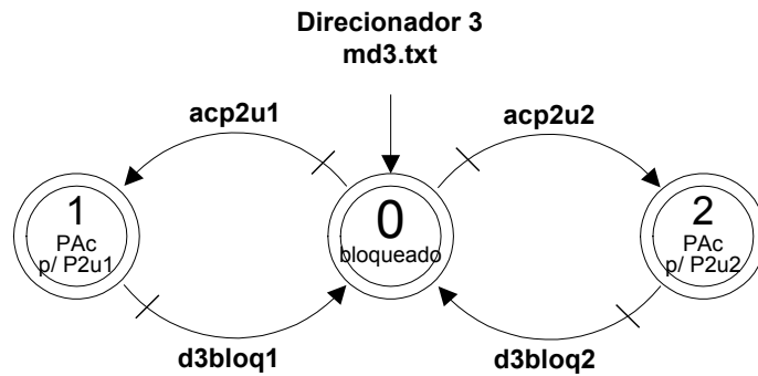
Figura 8.11 - Autômato do direcionador 3.
