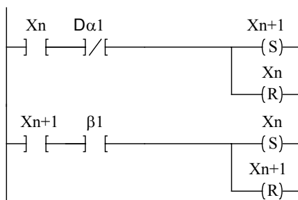
Figura 3.15 - Representação do sistema produto onde \alpha 1 é controlável e \beta 1 é não controlável.
