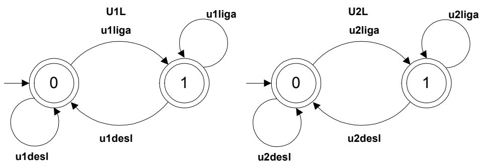
Figura 7.14 - Modelos de comportamento dos pedidos dos usuários 1 e 2 - comando liga/desliga.
