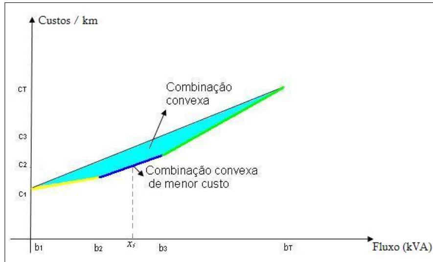
Figura 3.4: Combinação convexa de x_i
