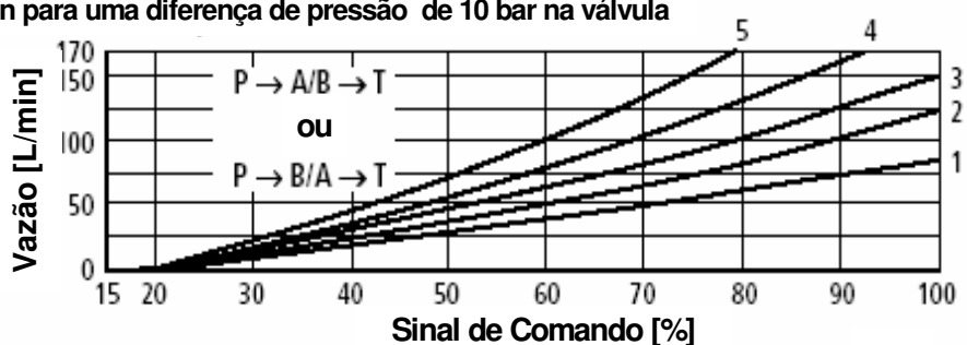
Figura 4.7 - Gráfico Vazão x Tensão fornecido no catálogo (BOSCH REXROTH, 2002a)
