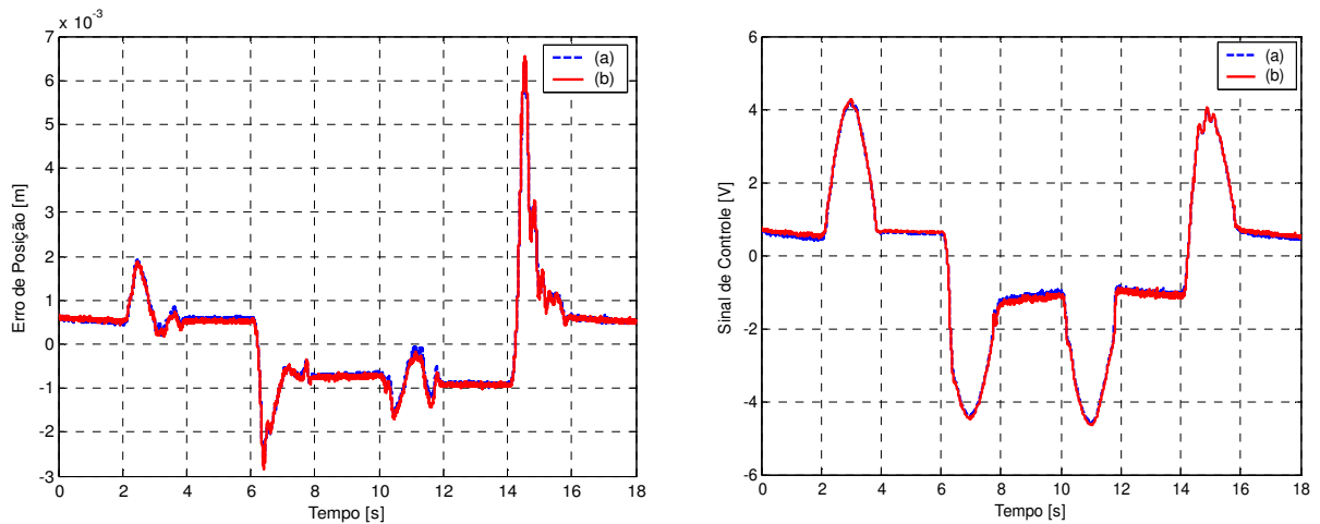
Figura 7.22 - Resposta do sistema com o controlador em cascata: (a) Sem compensação do vazamento, (b) Com compensação do vazamento, curso longo, com carga, K_p = 170 ,
