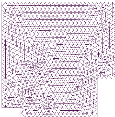
Figura 5.10: Discretização do domínio: 1900 elementos e 900 nós
