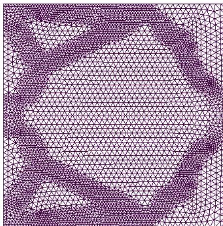
Figura 3.8: Domínio completo discretizado e refinado com 4486 nós e 8720 elementos.
