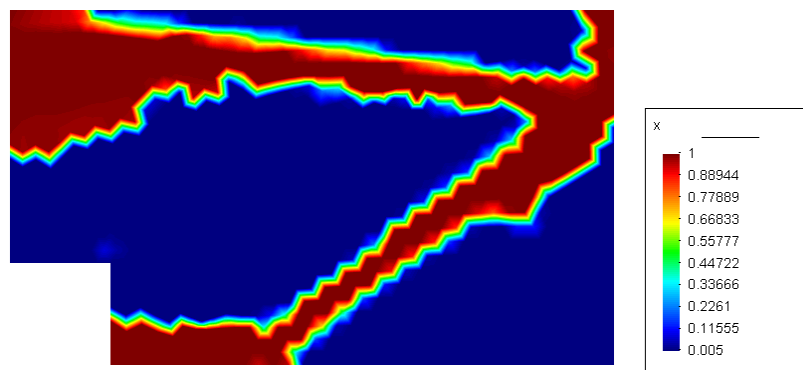
Figura 5.23: Topologia ótima obtida
