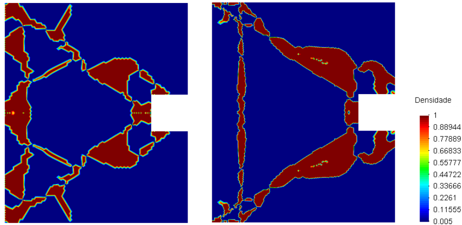
Figura 3.31: Topologias ótimas obtidas utilizando outros algoritmos de otimização: o MMA à esquerda e o de região de confiança à direita.
