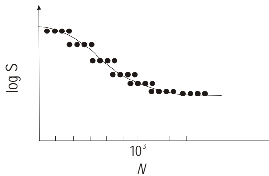
Figura 4.3: Diagrama de Wöhler
