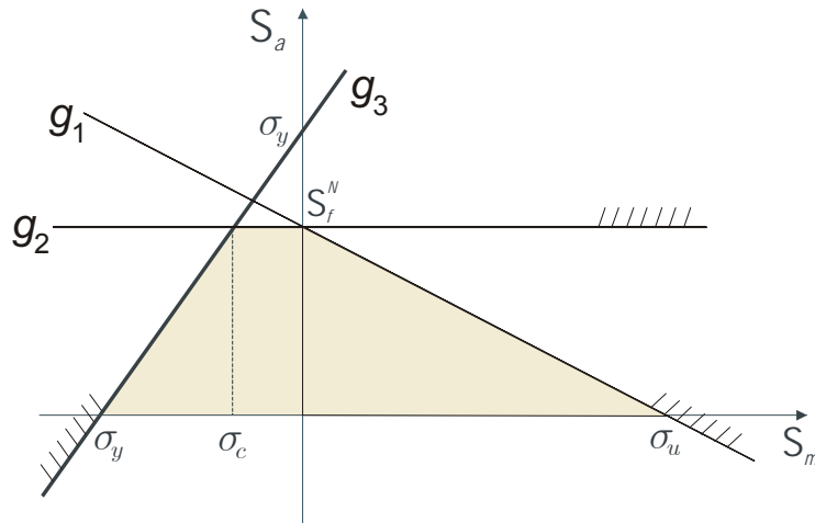
Figura 4.9: Restrições que delimitam a região de segurança no diagrama de Goodman modificado
