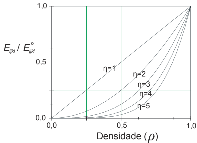
Figura 1.15: Curvas do modelo SIMP
