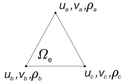
Figura 1.17: Elemento finito Tri3
