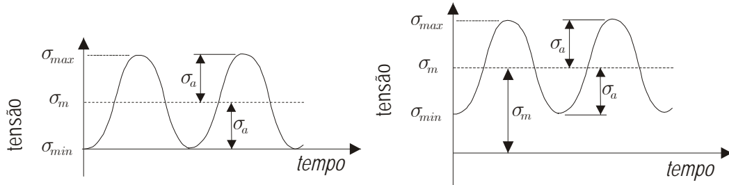
Figura 4.6: Exemplos de condições de carregamento com tensões flutuantes, comuns em mecanismos flexíveis
