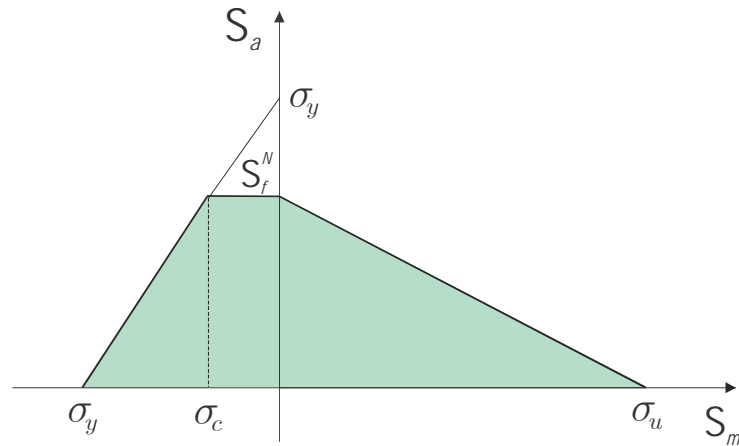
Figura 5.1: Diagrama de Goodman modificado
