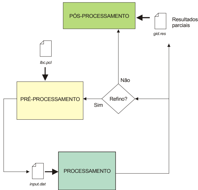
Figura A.1: Etapas do projeto de mecanismos flexíveis
