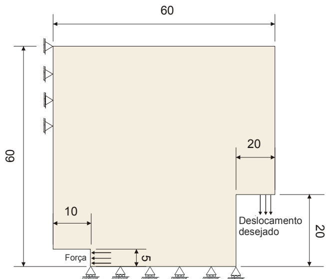
Figura 5.9: Domínio inicial do projeto: mecanismo de agarrar
