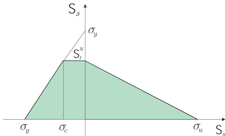
Figura 4.8: Diagrama de Goodman modificado
