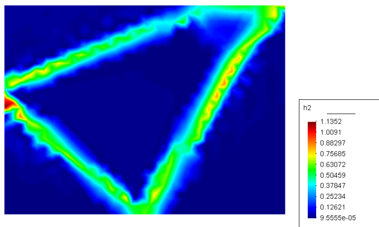
Figura 5.19: Função de falha h2
