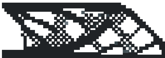
Figura 1.21: Topologia apresentando instabilidades de tabuleiro.
