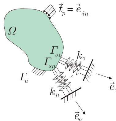
Figura 5.2: Definição do problema distribuído para \vec{u}_o(\vec{x})
