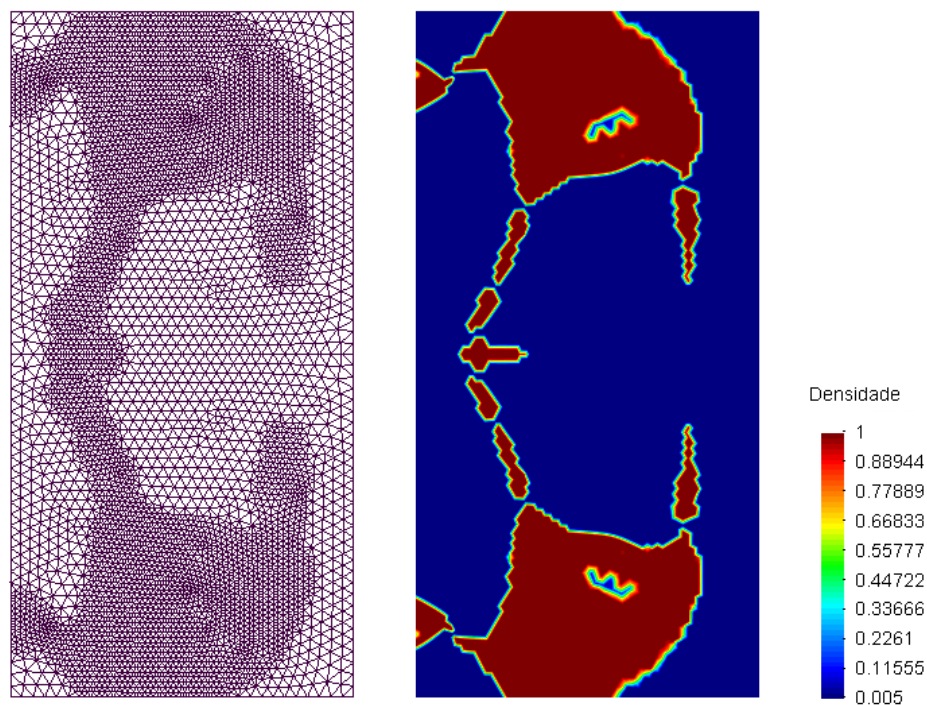
Figura 3.25: Malha refinada com 10174 elementos e 5196 nós e topologia final com restrição de quantidade de material de 30 %.
