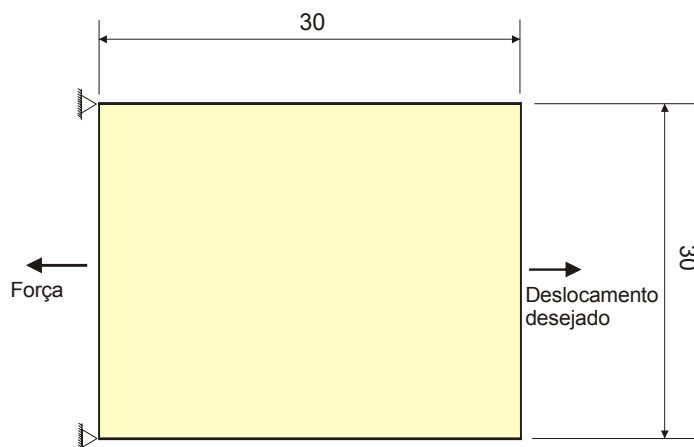
Figura 3.5: Inversor de deslocamento
