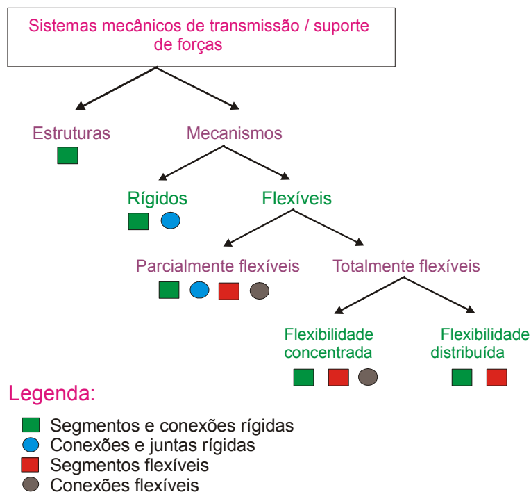
Figura 1.5: Classificação geral dos sistemas mecânicos
