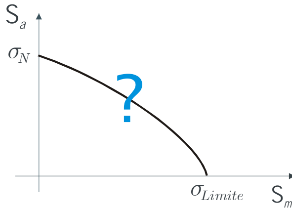
Figura 4.7: Estimativa do diagrama \sigma_a - \sigma_m
