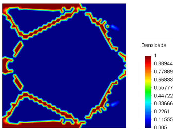
Figura 3.7: Topologia inicial obtida para o inversor
