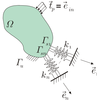
Figura 2.14: Definição do problema distribuído para \vec{u}_o(\vec{x})
