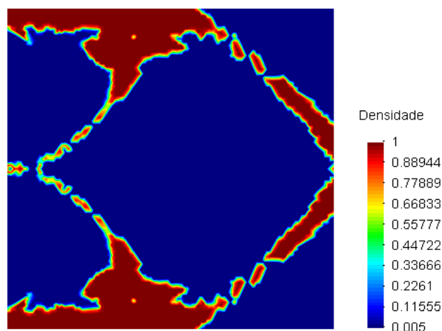
Figura 3.13: Topologia obtida considerando a restrição de gradientes.
