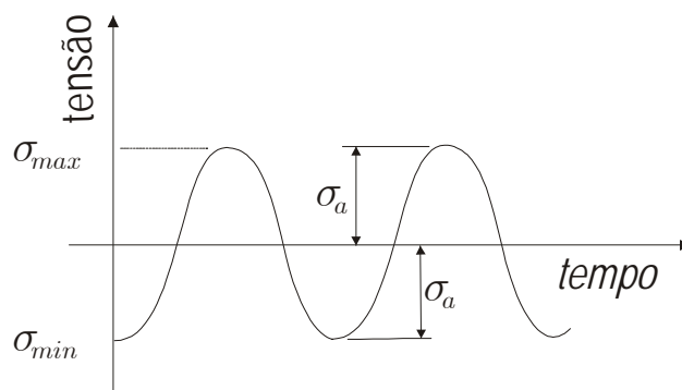
Figura 4.5: Gráfico tensão x tempo para um carregamento completamente reverso
