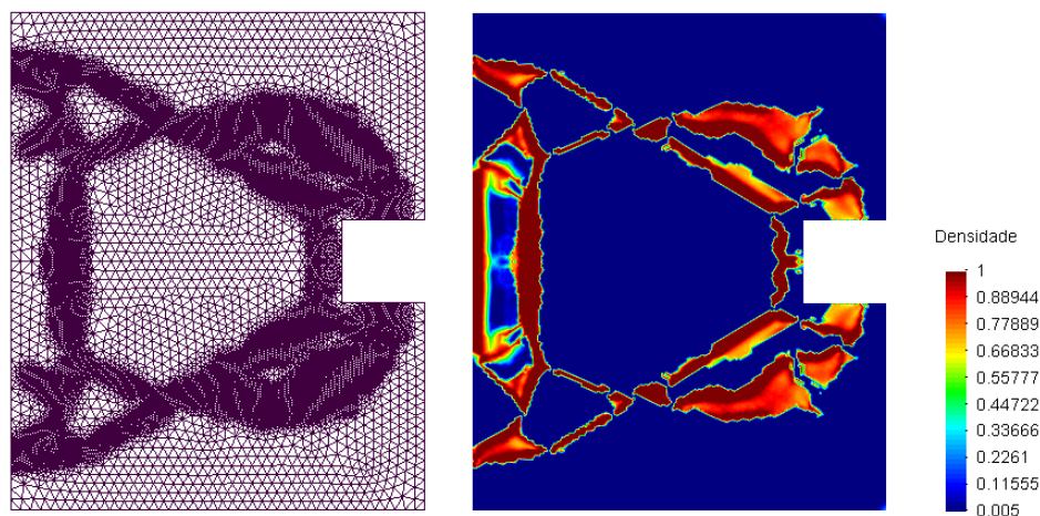
Figura 3.30: Malha refinada com 29530 elementos e 14898 nós e topologia ótima obtida
