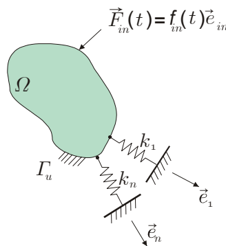
Figura 4.10: Carregamento e molas discretas
