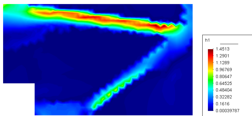
Figura 5.24: Função de falha h_1
