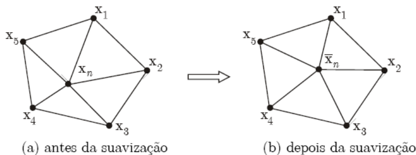
Figura 3.4: Processo de suavização Laplaciano no elemento Tri3
