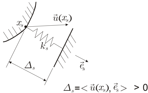
Figura 2.5: Deformação da mola (compressão)
