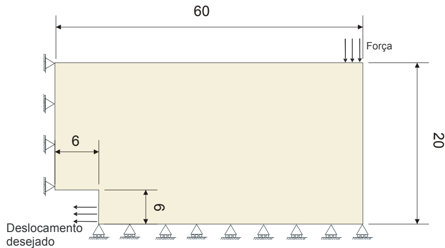
Figura 5.21: Domínio inicial do projeto
