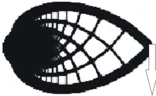
Figura 1.12: Resultado obtido pela otimização topológica para o problema de Michell
