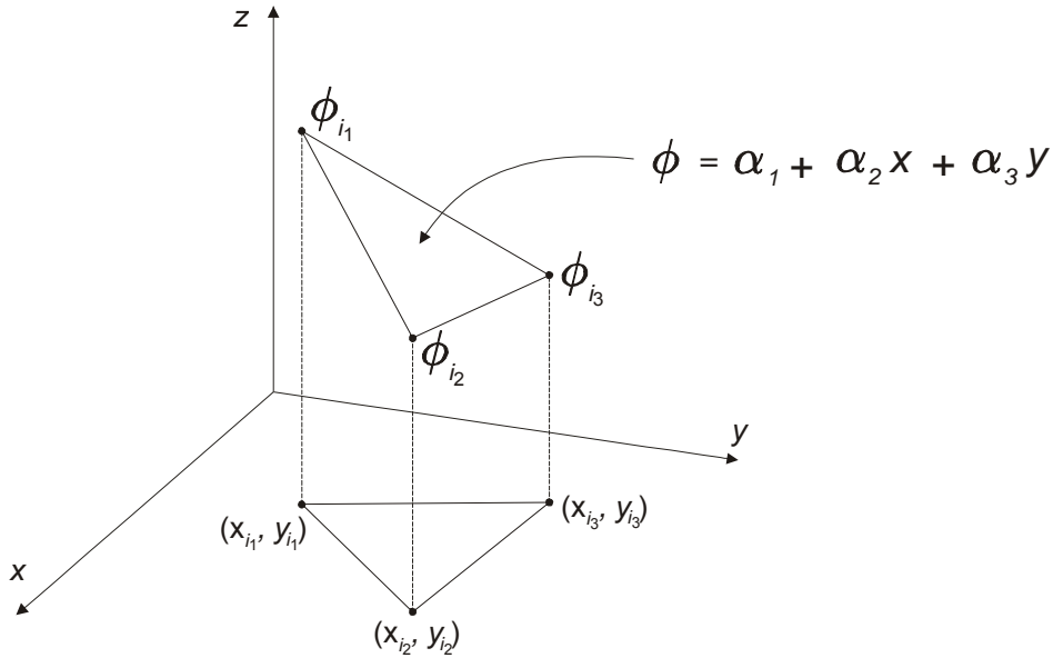
Figura 2.9: Elemento bidimensional triangular
