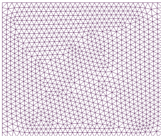
Figura 5.4: Discretização do domínio do projeto: malha com 1900 elementos e 900 nós
