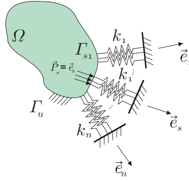
Figura 2.8: Definição do problema distribuído para \vec{u}_s(\vec{x})
