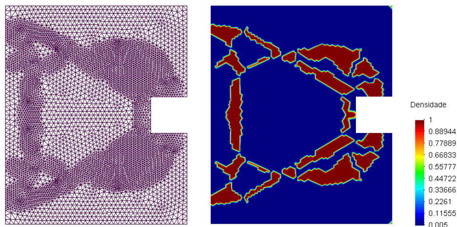
Figura 3.29: Malha refinada com 10830 elementos e 5530 nós e topologia ótima parcial.
