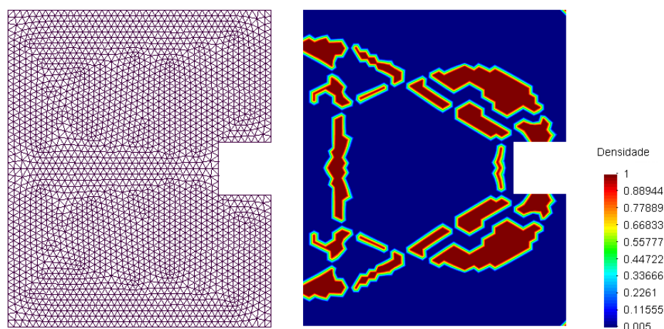
Figura 3.28: Malha inicial com 4702 elementos e 2452 nós e topologia ótima parcial
