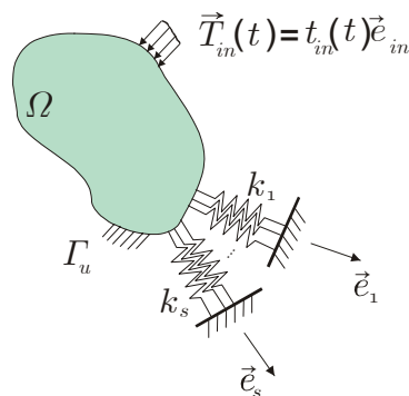
Figura 4.11: Carregamento e molas distribuídas
