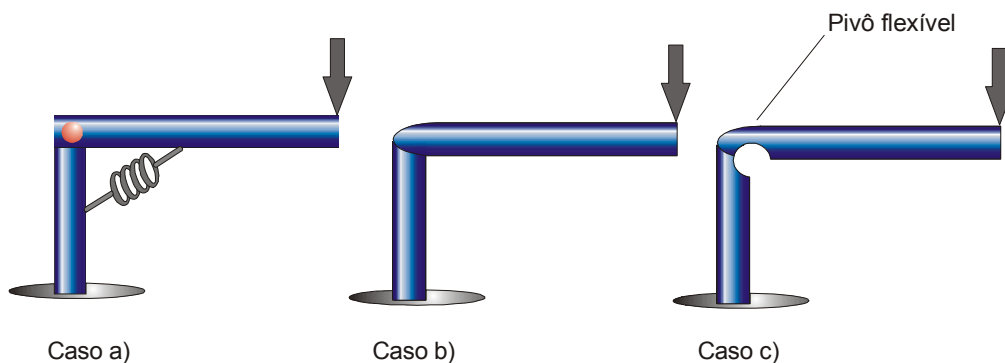
Figura 1.4: Tipos de mecanismos: (a) mecanismo de corpo rígido convencional; (b) de flexibilidade distribuída e (c) de flexibilidade concentrada.
