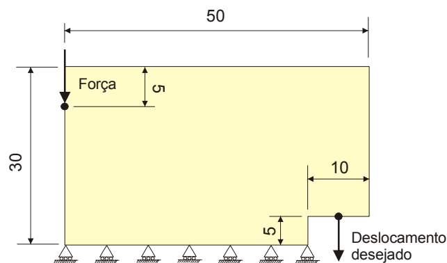
Figura 3.27: Domínio inicial do projeto do alicate flexível
