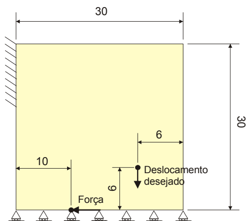
Figura 3.21: Mecanismo de agarrar
