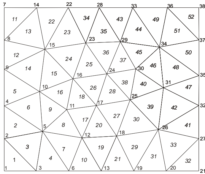
Figura 4.14: Domínio discretizado: 52 elementos e 38 nós
