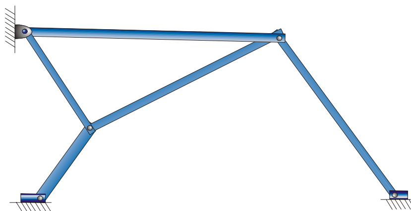
Figura 3.12: Mecanismo inversor de corpo rígido convencional
