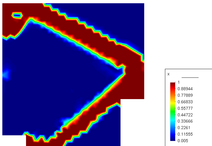
Figura 5.11: Topologia ótima final do mecanismo de agarrar
