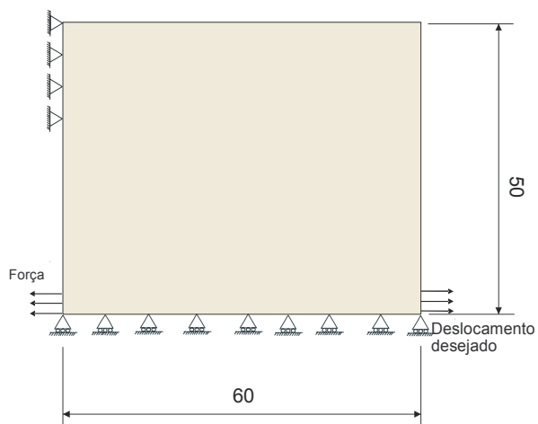
Figura 5.3: Domínio inicial do projeto do mecanismo inversor de deslocamento
