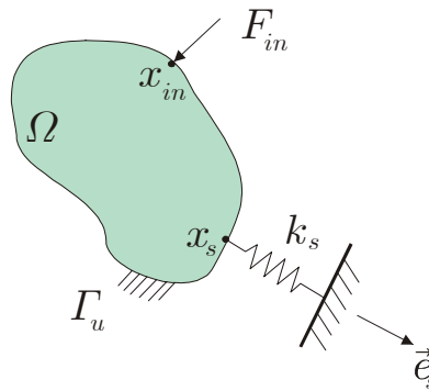
Figura 2.13: Modelo de mecanismo
