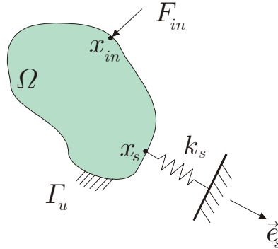
Figura 3.1: Modelo de mecanismo
