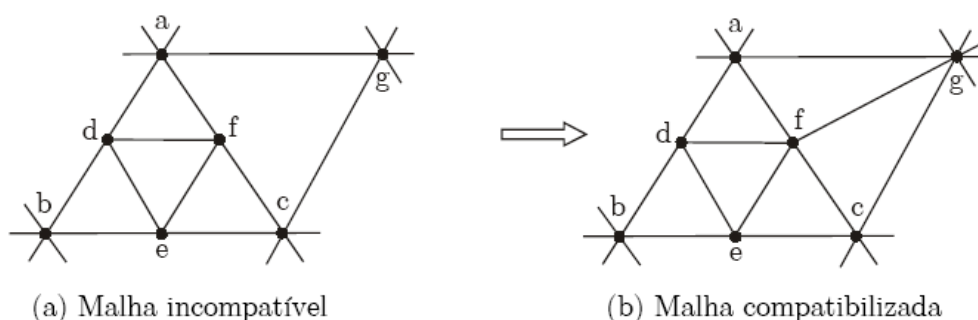
Figura 3.3: Elemento de transição compatibiliza a malha.
