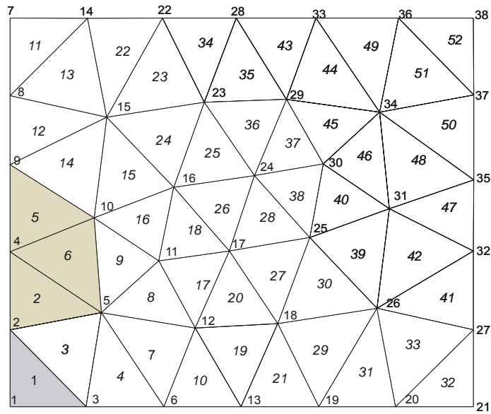
Figura 4.16: Segundo patch nodal
