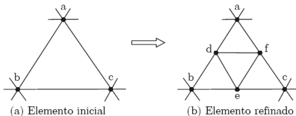
Figura 3.2: Estratégia de refinamento para elementos Tri3
