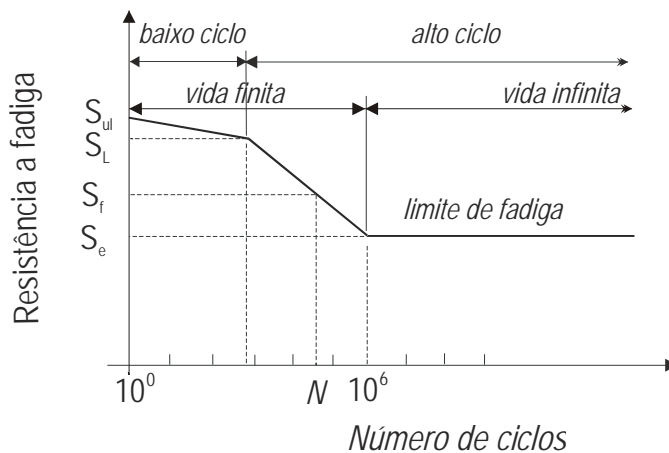
Figura 4.4: Diagrama S - N típico para um aço
