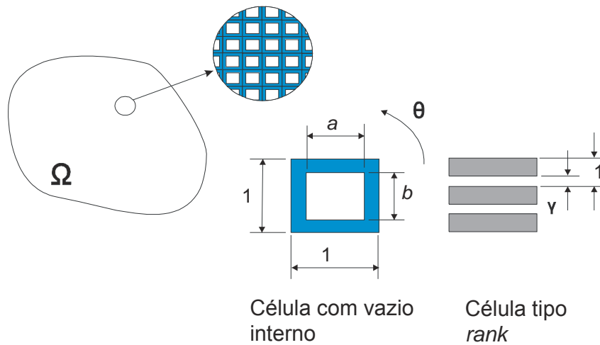
Figura 1.14: Microestruturas para o método de homogeneização
