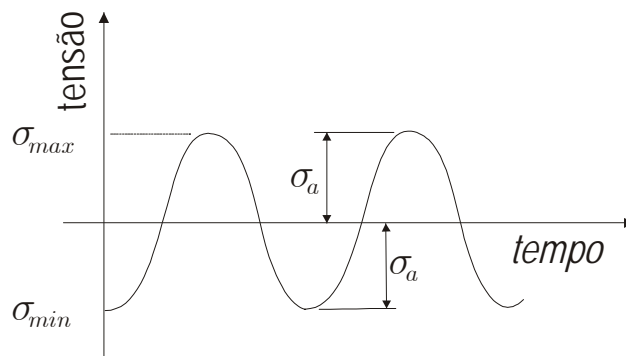
Figura 4.2: Variação da tensão em um ensaio de flexão rotativa
