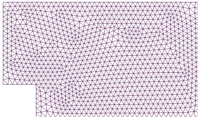
Figura 5.22: Domínio discretizado: malha com 2122 elementos e 1127 nós
