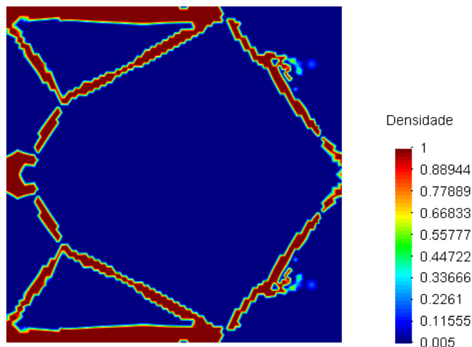
Figura 3.9: Topologia obtida no primeiro refino, malha com 8720 elementos
