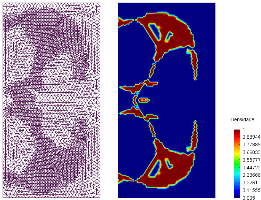
Figura 3.23: Malha final com 9119 elementos e 4690 nós e topologia ótima
