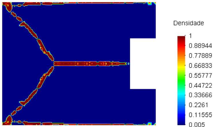
Figura 3.19: Mecanismo sem penalização adequada da restrição de material.
