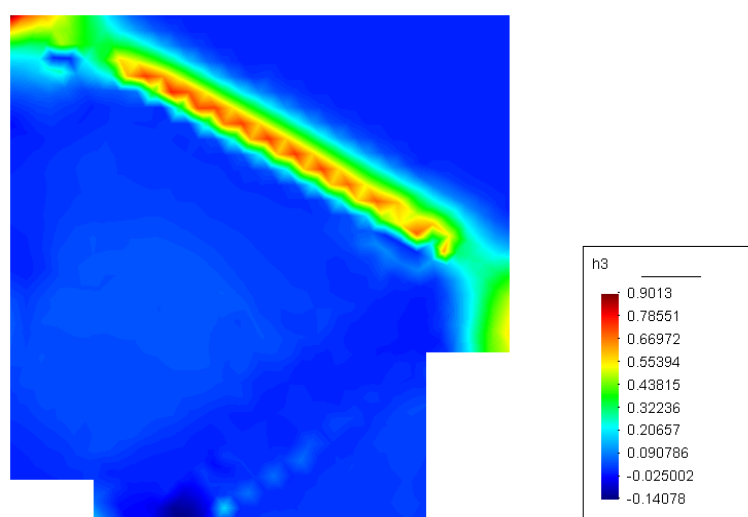
Figura 5.14: Função de falha h3
