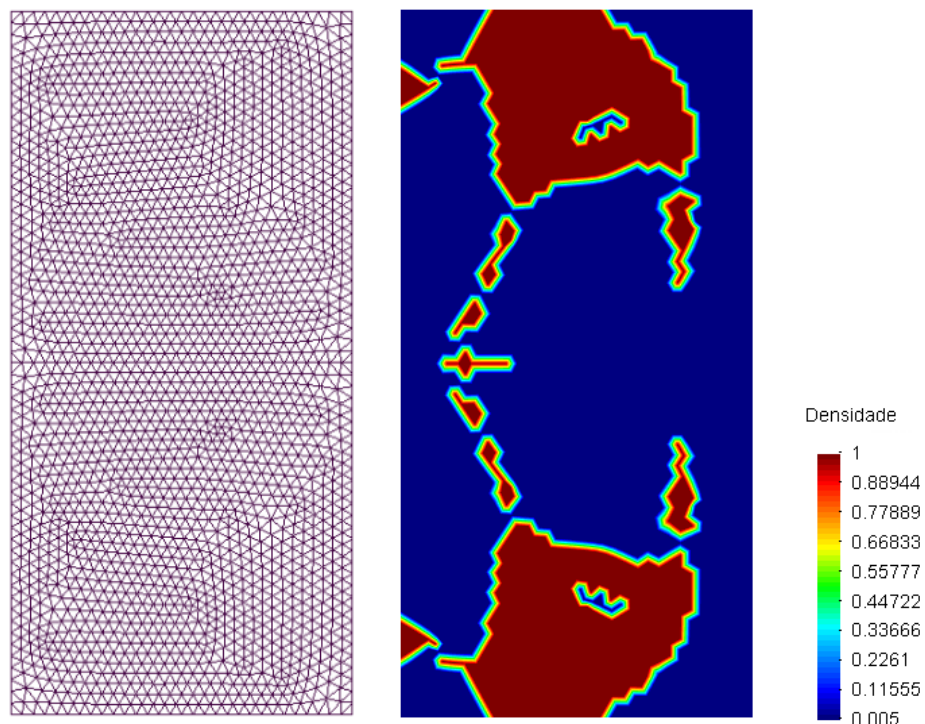
Figura 3.24: Malha e topologia inicial com restrição de material de 30%
