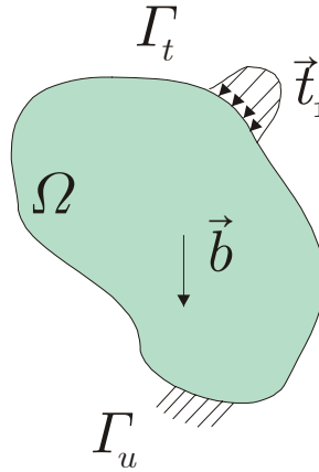
Figura 2.2: Um corpo elástico submetido a um carregamento \vec{t}_1
