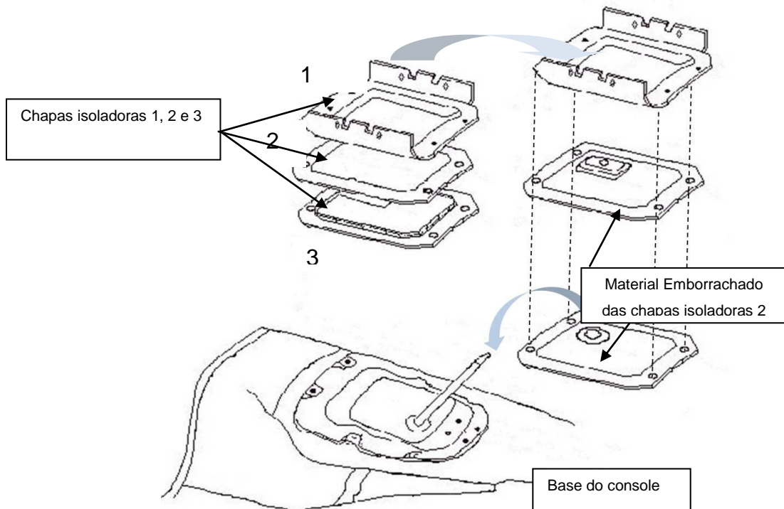
FIGURA 16 - MONTAGEM DO CONJUNTO DE CHAPAS ISOLADORAS DA BASE CONSOLE CENTRAL DO VEÍCULO ANTES DA MODIFICAÇÃO – MODELO 4X2
