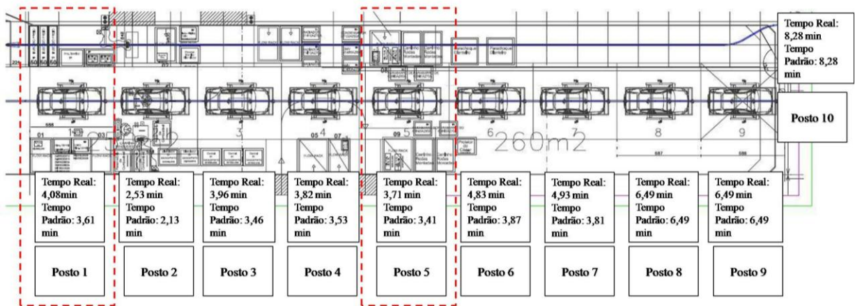
FIGURA 15 - TEMPOS REAL E PADRÃO DOS POSTOS DE MONTAGEM COMPREENDIDOS PELA ETAPA DE PROCESSO ESCOLHIDA
