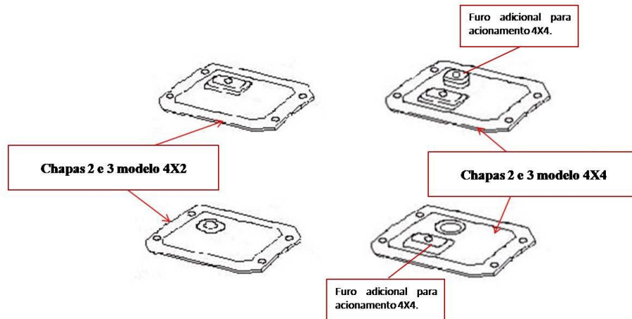
FIGURA 17 - DIFERENÇAS ENTRE AS CHAPAS ISOLADORAS 2 E 3, MODELOS 4X2 E 4X4
