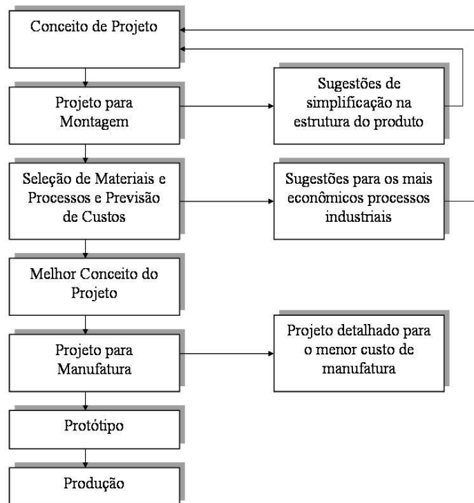
FIGURA 11 - ESTÁGIOS DO DFMA
