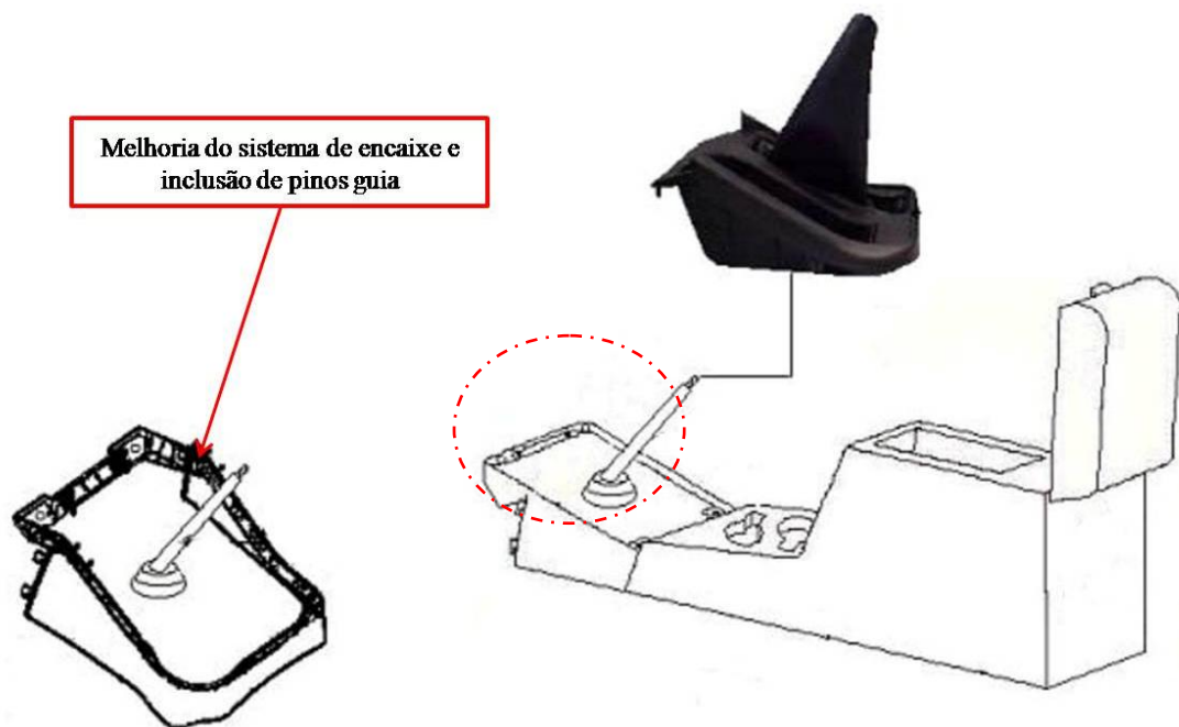
FIGURA 22 - MELHORIA DO SISTEMA DO SISTEMA DE FIXAÇÃO DA COIFA DA ALAVANCA DE MUDANÇAS
