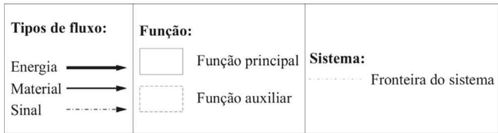
FIGURA AP 6.1 – Símbolos para a elaboração de uma estrutura de funções (Pahl e Beitz, 1996).
