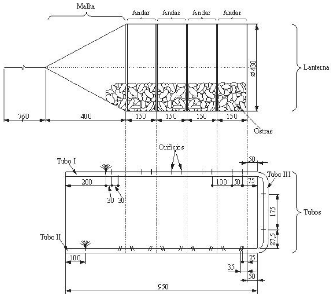
FIGURA 5.3 – Localização dos orificios nos tubos.
