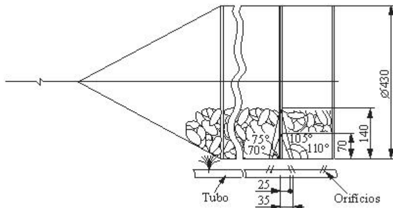
FIGURA 5.4 – Orificios para limpeza das partes inferior e superior das bandejas.
