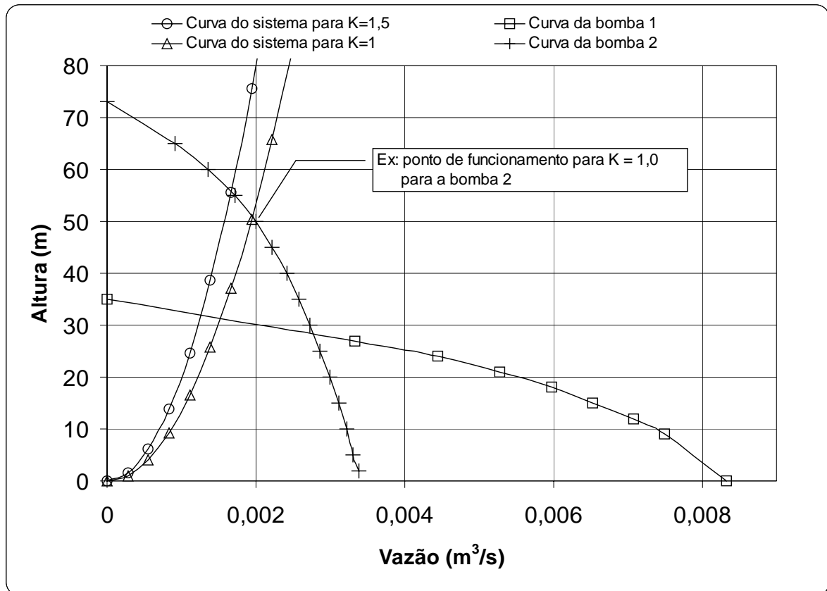
FIGURA 5.8 – Curvas das bombas X curvas de perda de carga do sistema.
