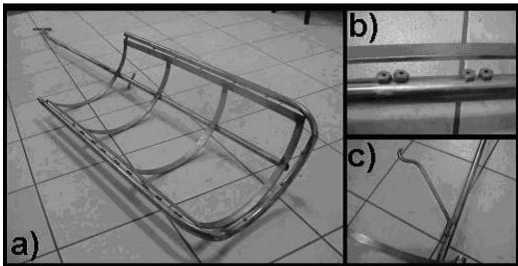
FIGURA 5.14 – Protótipo de lavagem de lanternas. a) conjunto, b) detalhe dos bicos e c) gancho.
