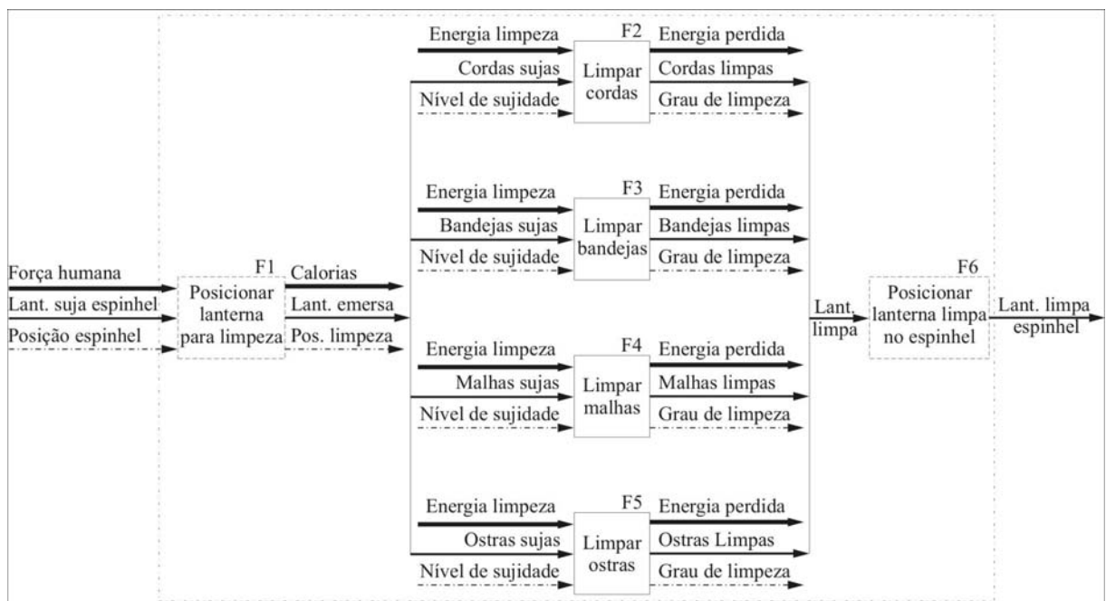
FIGURA AP 6.3 – Nível 1 da estrutura funcional: funções principais e auxiliares.
