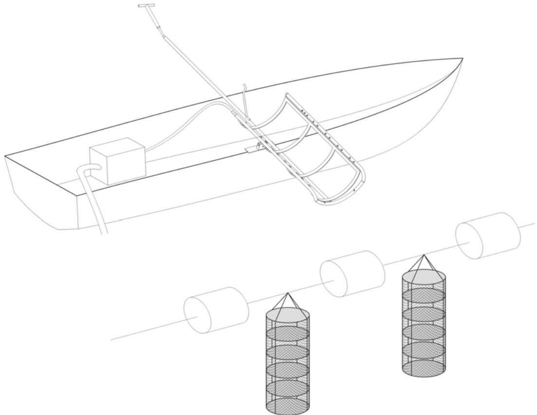
FIGURA 5.15 – Esquema de funcionamento do protótipo.
