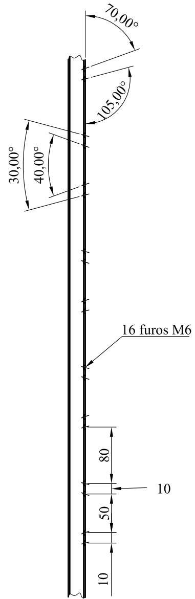
Corte AA
