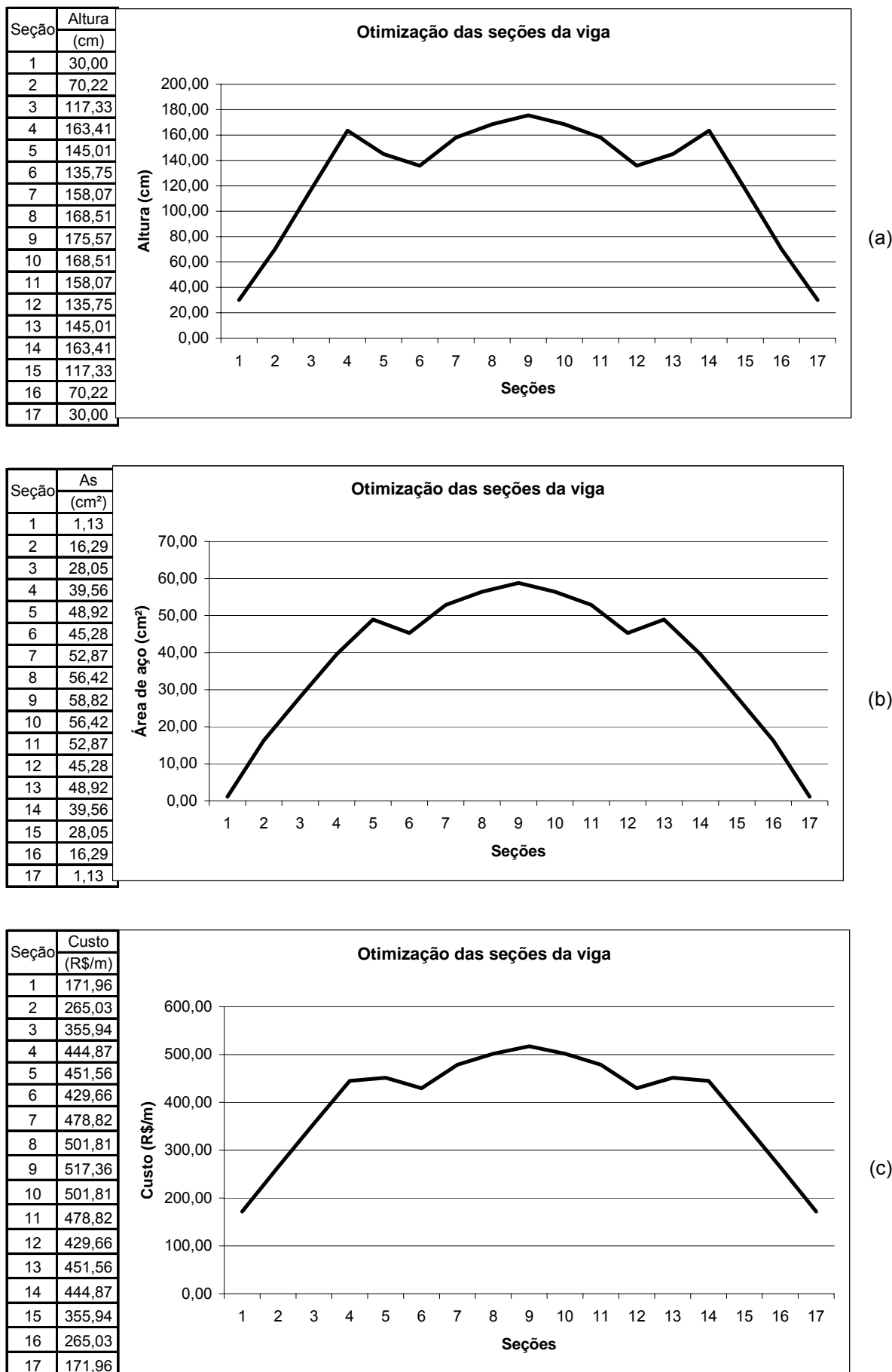
Figura 6.3.11 – Resultados para viga otimizada
