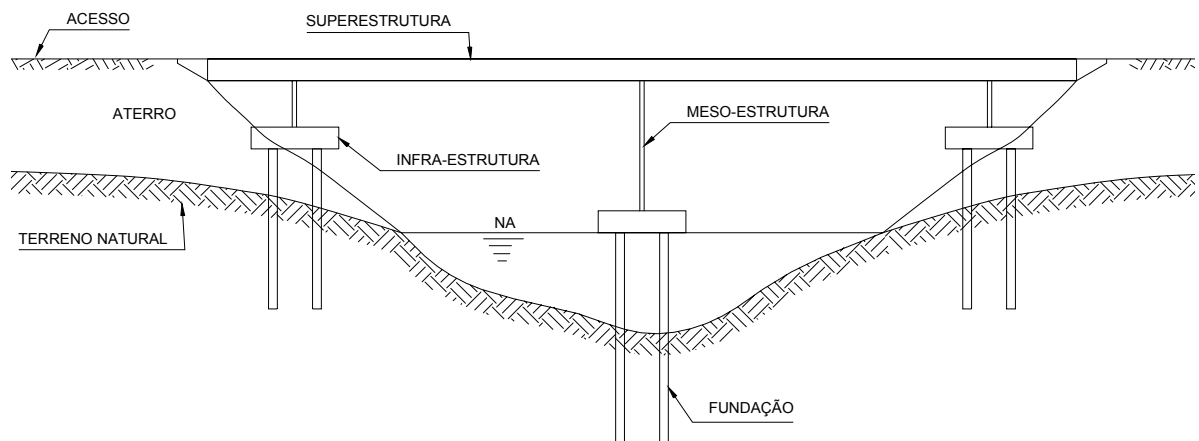
Figura – 2.2.1 Elementos de uma ponte - MASON
