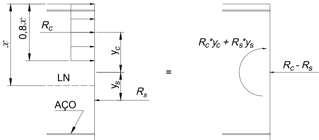
Figura 3.2.2 – Esforços resistentes
