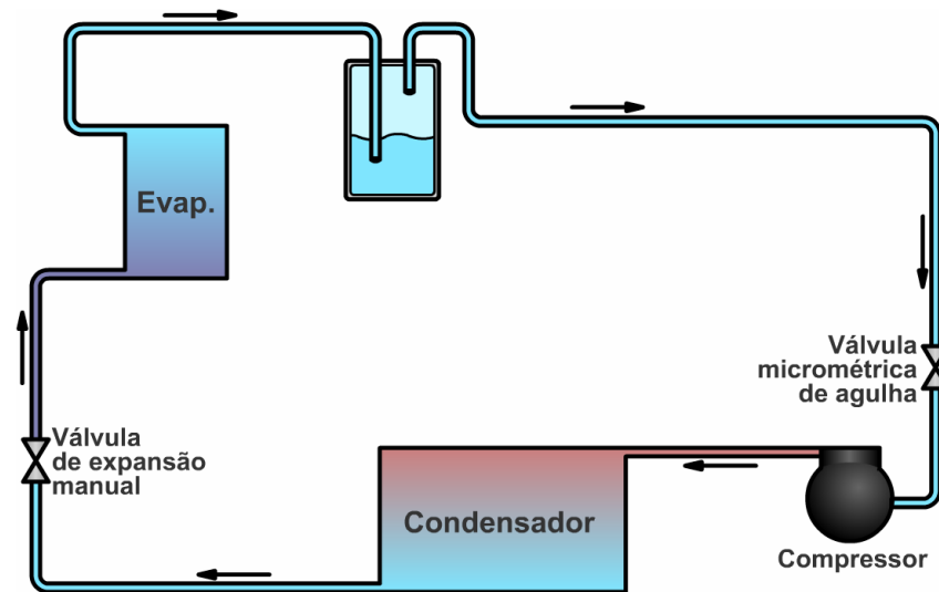
Figura 3.11 – Sistema de refrigeração auxiliar.
