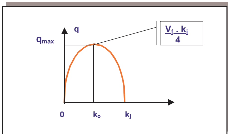
Figura 2.3 – Relação entre a concentração e fluxo – Equação de Greenshields
