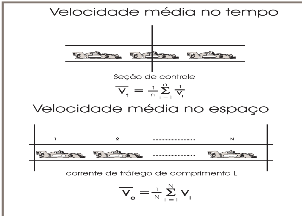
Figura 2.1 – Velocidades Médias no Tempo e no Espaço
