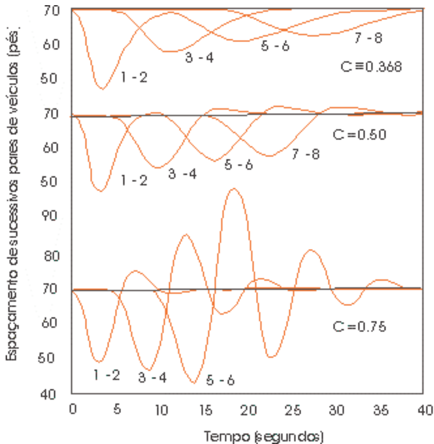
Figura 2.11 – Espaçamento entre pares de veículos, Pereira (2002)
