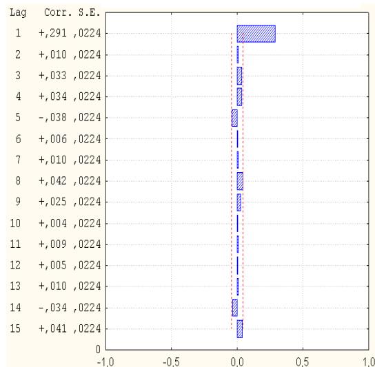
Figura 4.3 – Função de Auto-Correlação Parcial (PACF).
