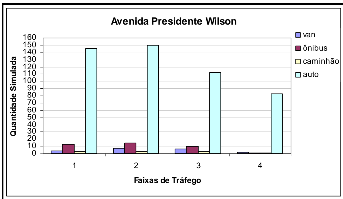
Figura 5.23 – Contagem de campo classificada – tamanho da fila simulada
