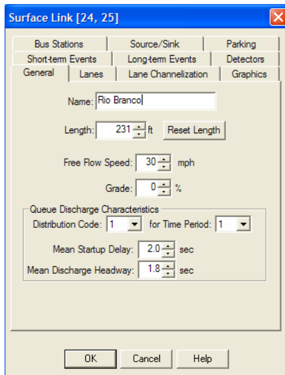
Figura 5.16. – Janela de entrada dos dados dos links.
