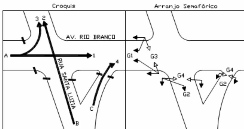
Figura 5.8. – Croqui referente aos grupos semafóricos de uma interseção do modelo.
