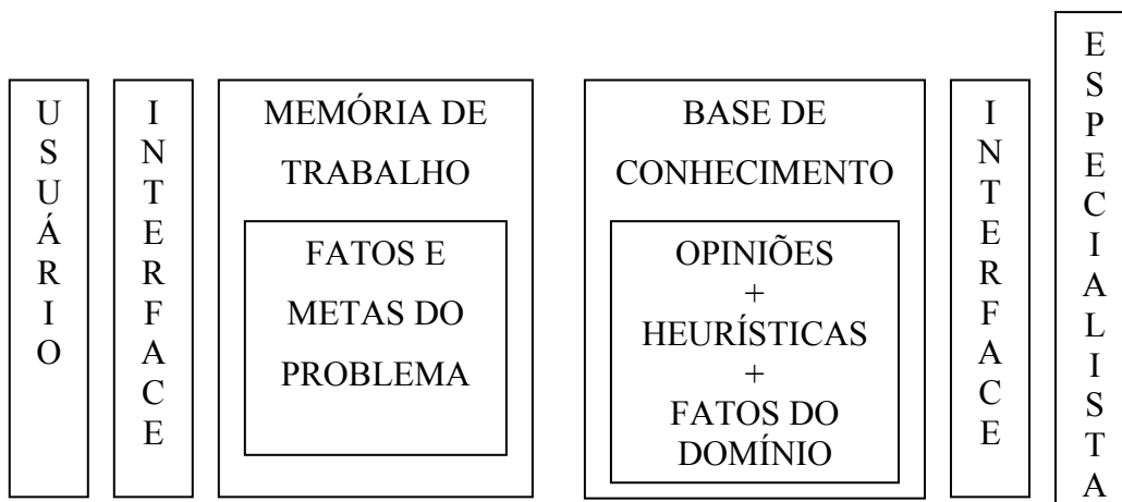
Figura 3.1. Arquitetura Básica dos Sistemas Especialistas.
