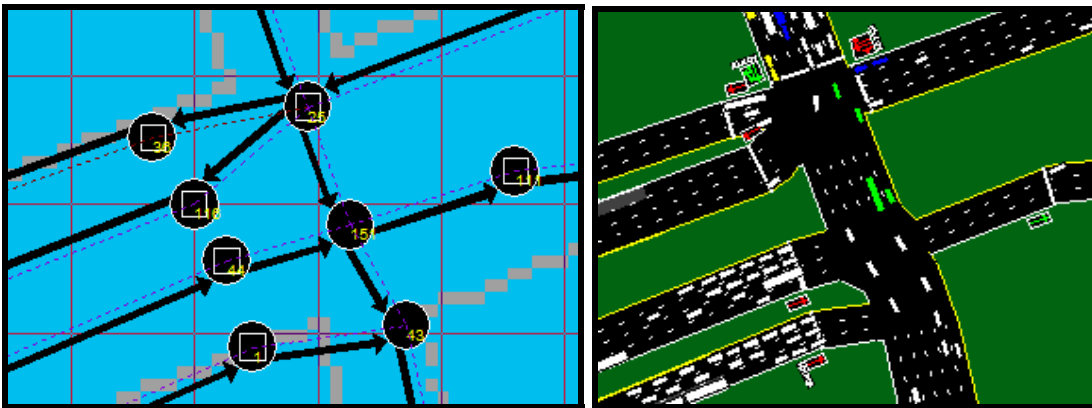
Figura 5.12. Composição de nós de uma interseção: Av. Rio Branco x Av. Pres. Vargas
