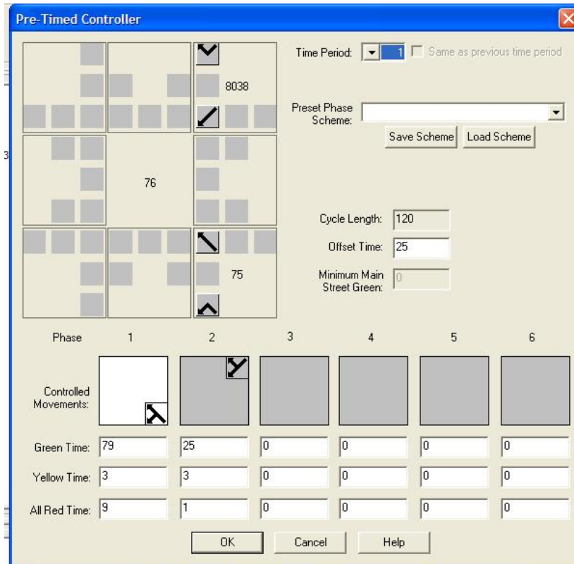
Figura 5.17. – Janela de entrada dos dados dos semáforos.
