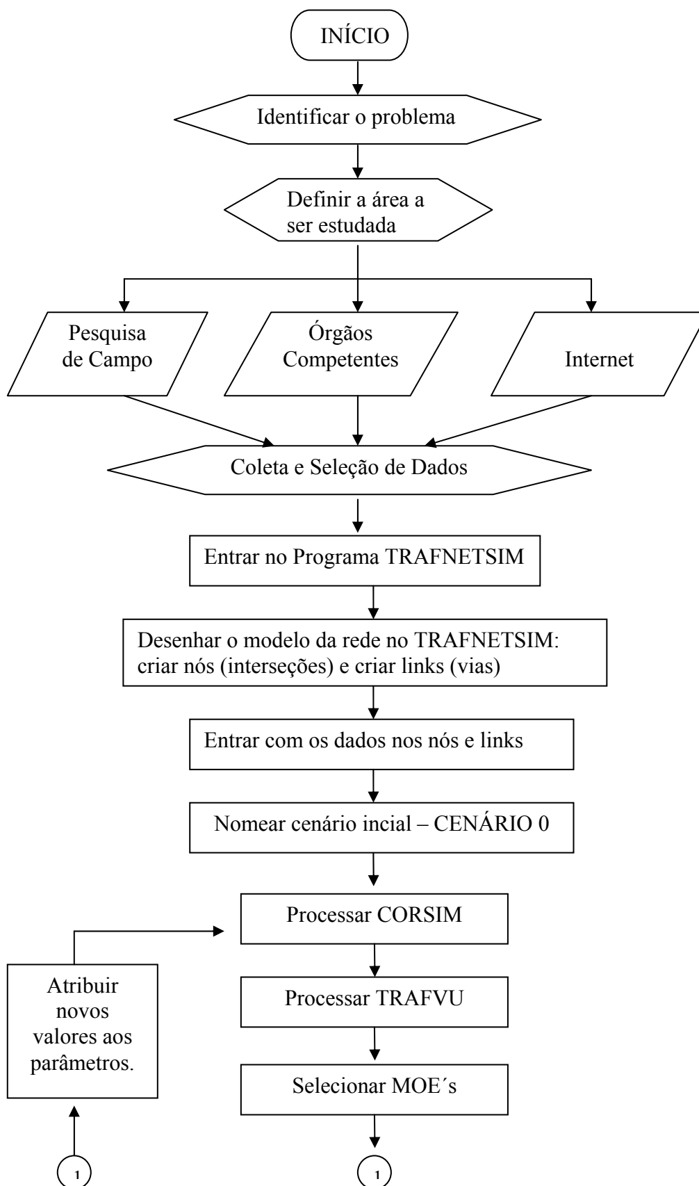
Figura 4.5. – Fluxograma do procedimento para desenvolver alternativas de tráfego em centros urbanos devido à incidentes.
