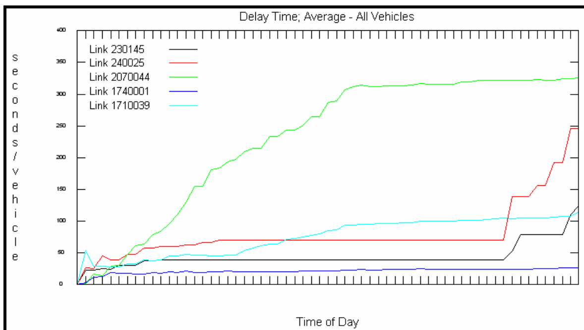
Figura 5.24 – Exemplo de resultados de saída.
