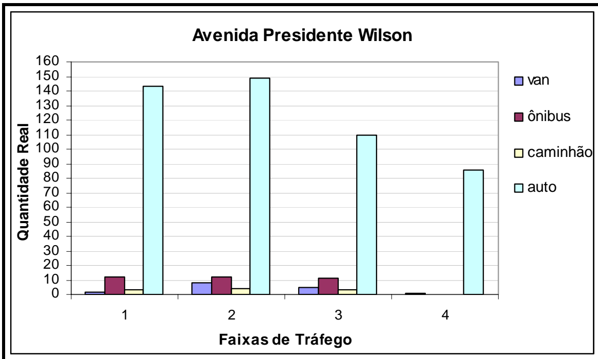
Figura 5.22 – Contagem de campo classificada – tamanho da fila real
