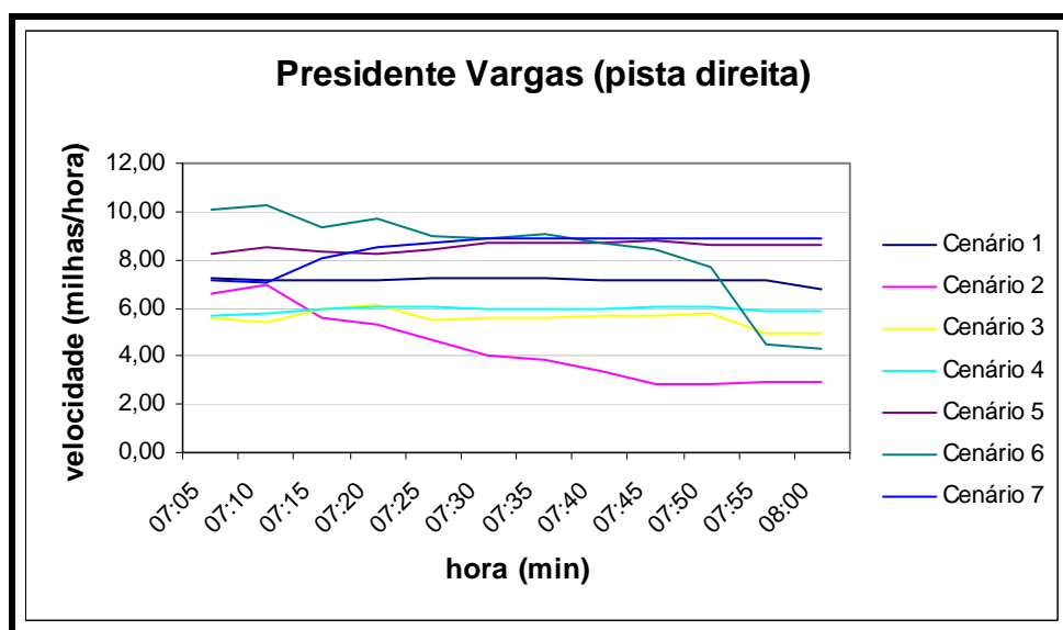
Figura 4.4. – Comparação dos diversos cenários – resultado de uma das variáveis (velocidade) em uma determinada via do modelo.
