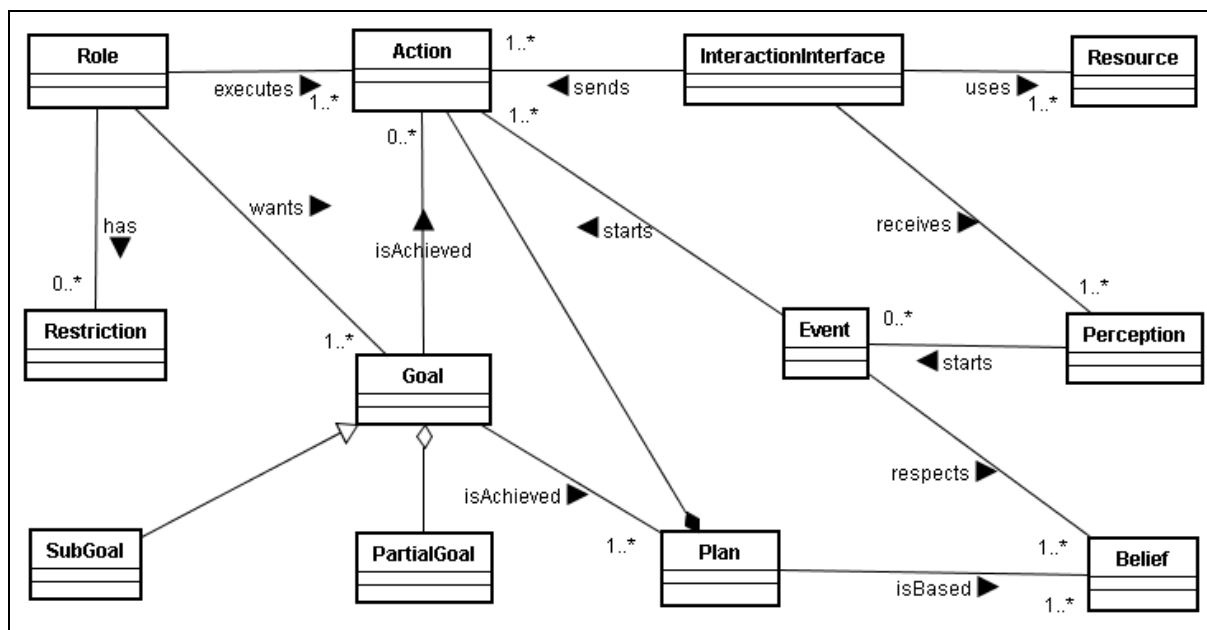
Figura 3.1 – Meta-modelo inicial proposto.
