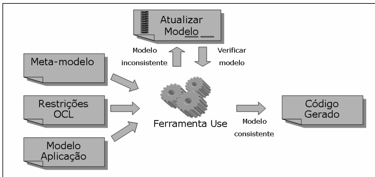
Figura 4.1 – Processo de Consistência de Modelos e Geração de Código.
