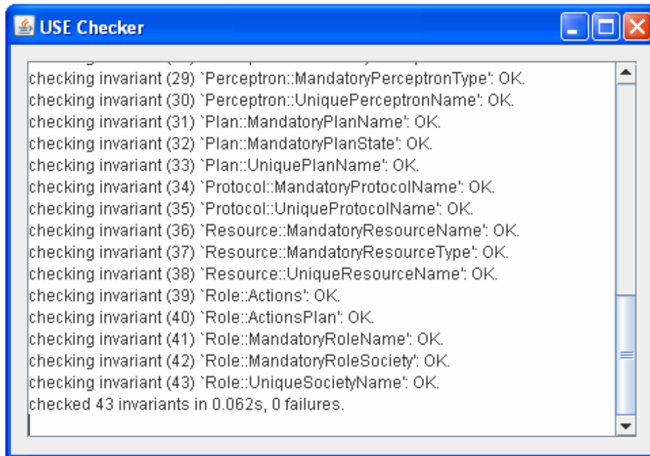
Figura 5.5 – Modelo Consistente com as Restrições Aplicadas.
