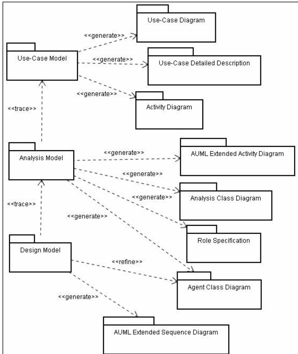
Figura 2.4 – Modelos do MASUP e artefatos [BAS05].
