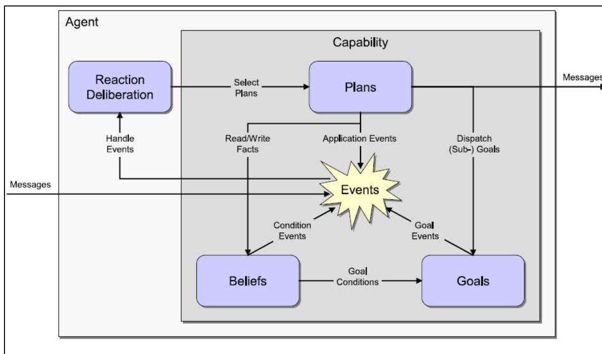
Figura 2.17 – Visão Geral da Arquitetura Abstrata Jadex [POK05].
