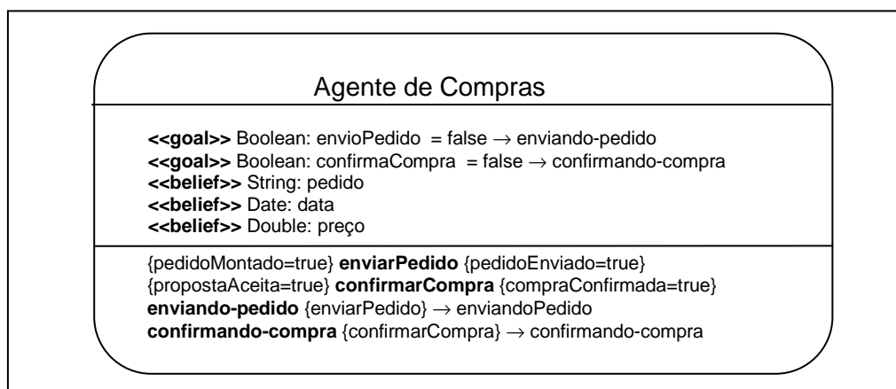
Figura 2.14 – AgentClass – Agente de Compras.
