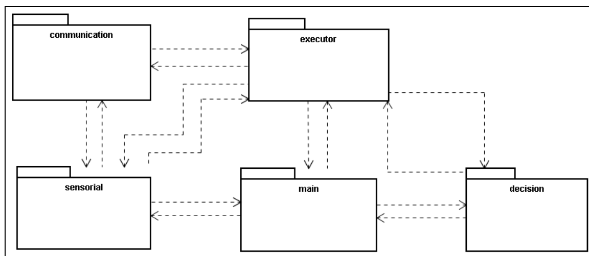
Figura 3.3 – Visão Geral dos Pacotes do Meta-modelo.
