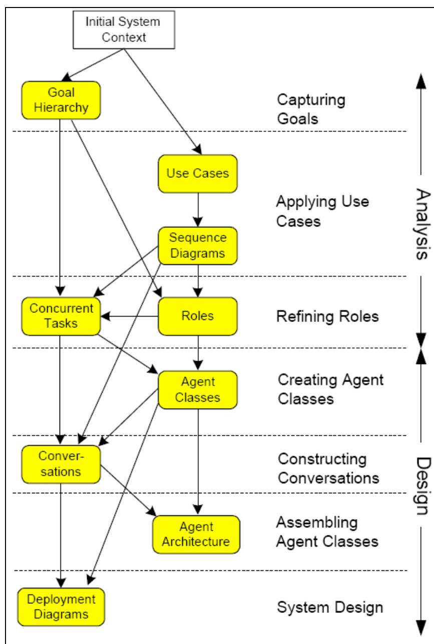
Figura 2.7 – Visão geral das fases da metodologia MaSE [DEL01].
