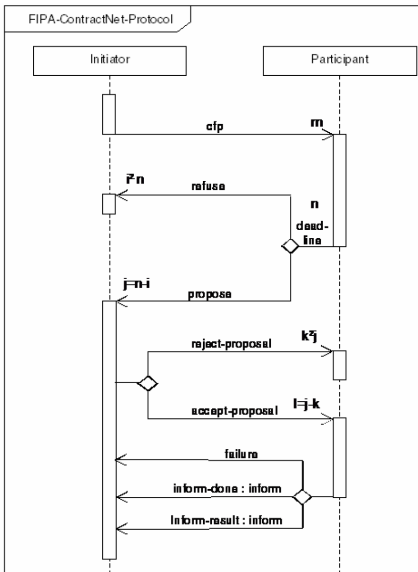
Figura 5.1 – Estrutura do protocolo Contract Net [FIP07a].
