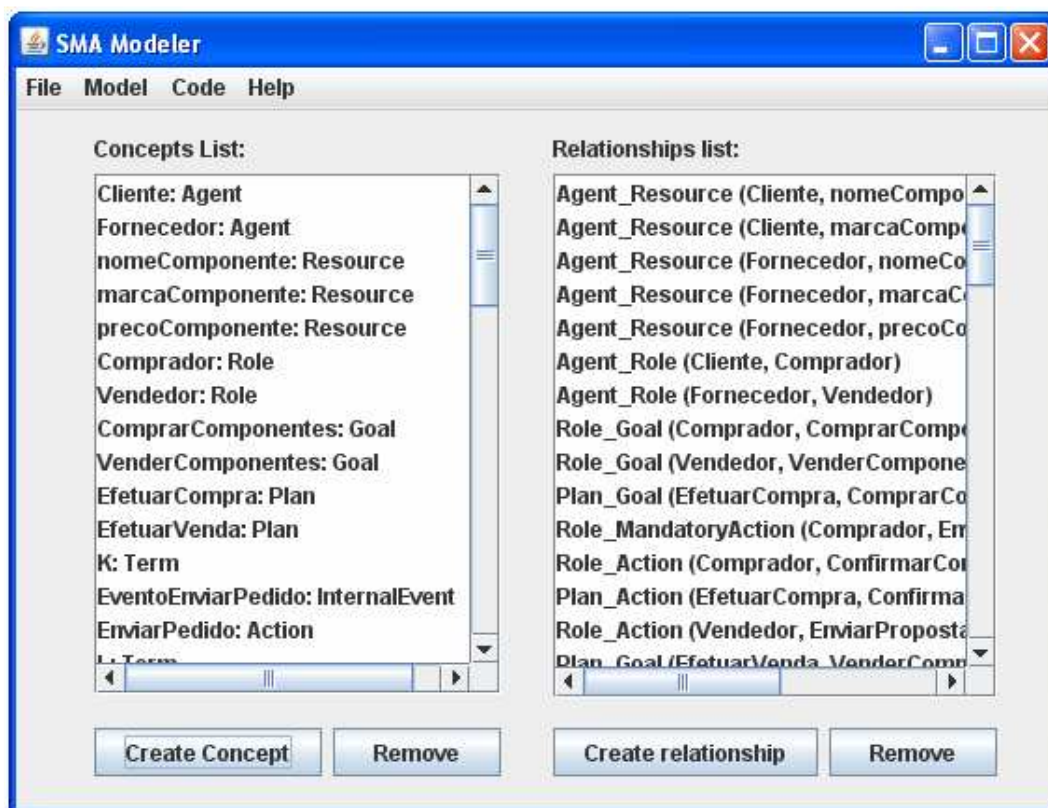
Figura 5.3 – Tela com Modelo Carregado.
