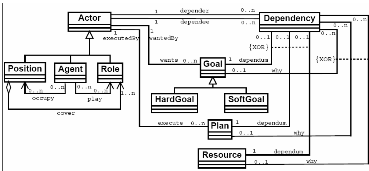
Figura 2.6 – Meta-modelo Tropos [GIO05].
