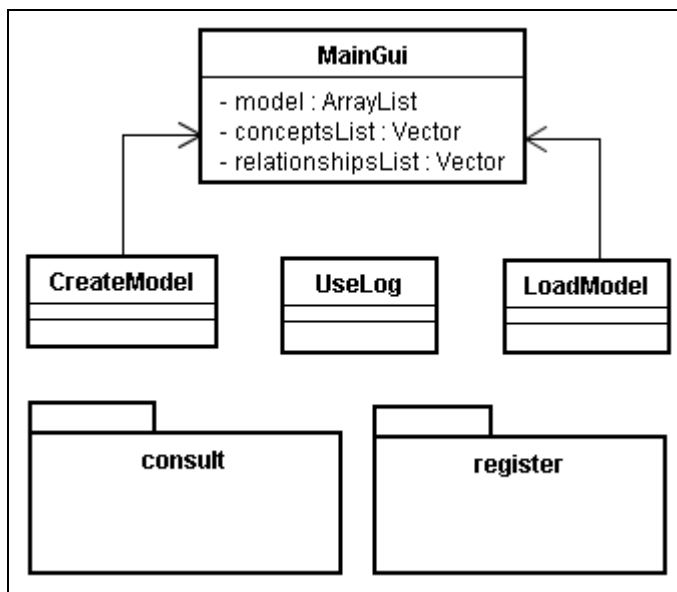
Figura 4.4 – Estrutura geral do pacote gui .
