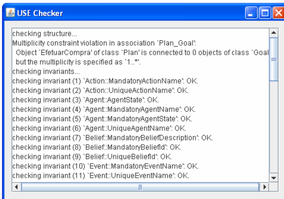
Figura 5.6 – Erro de Consistência Estrutural.
