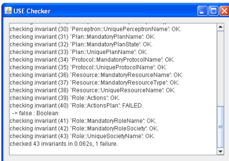
Figura 5.7 – Erro de Consistência nas Restrições de Integridade.
