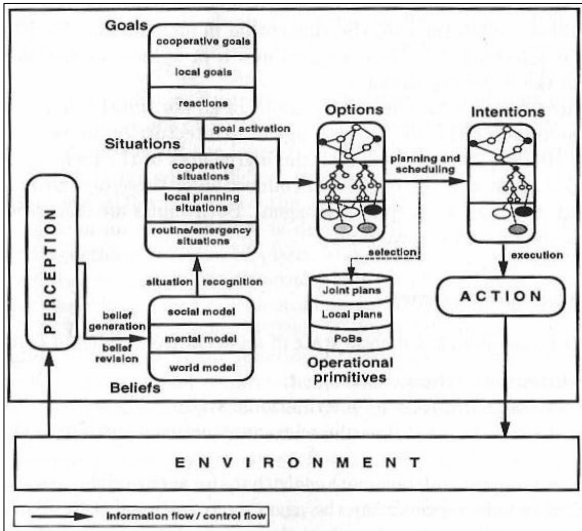
Figura 2.2 – Modelo Conceitual de um Agente INTERRAP [MÜL96].
