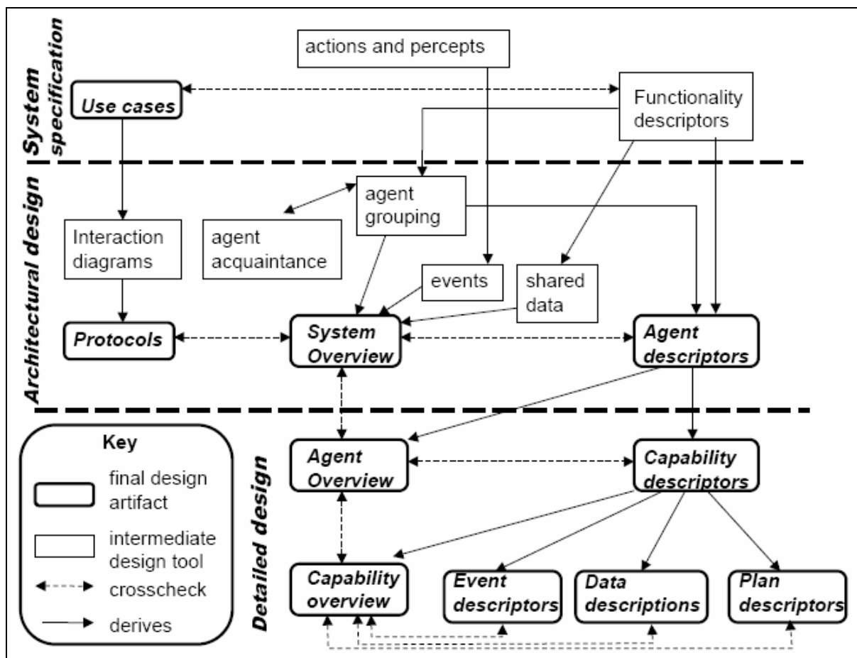
Figura 2.10 – Visão geral das fases do Prometheus [PAD02].
