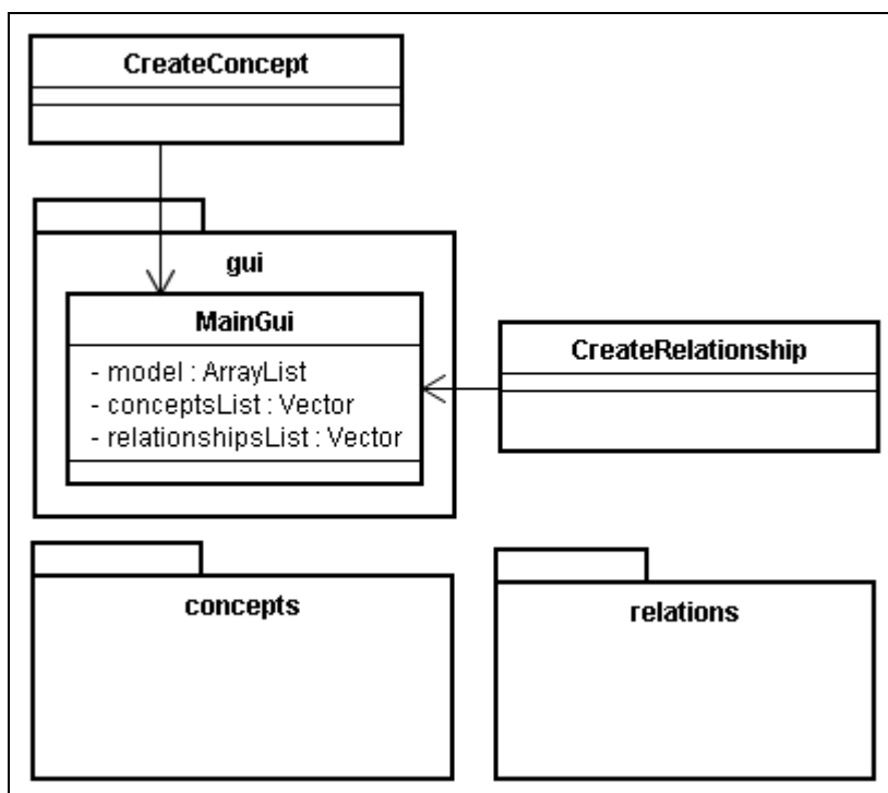
Figura 4.6 – Estrutura geral do pacote gui.register .
