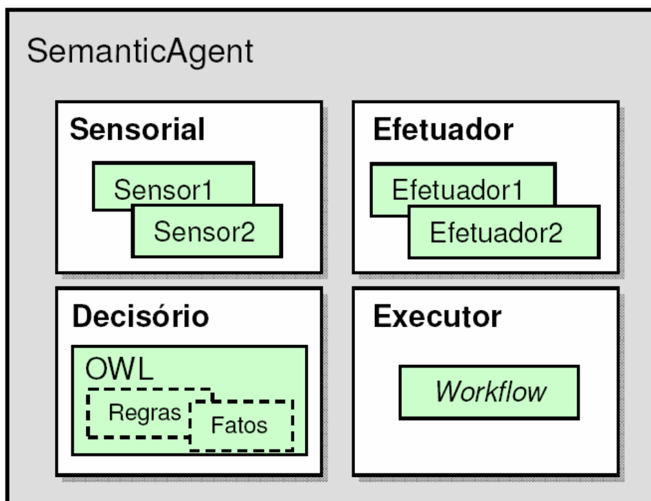
Figura 2.16 – Modelo do Agente [ESC06].
