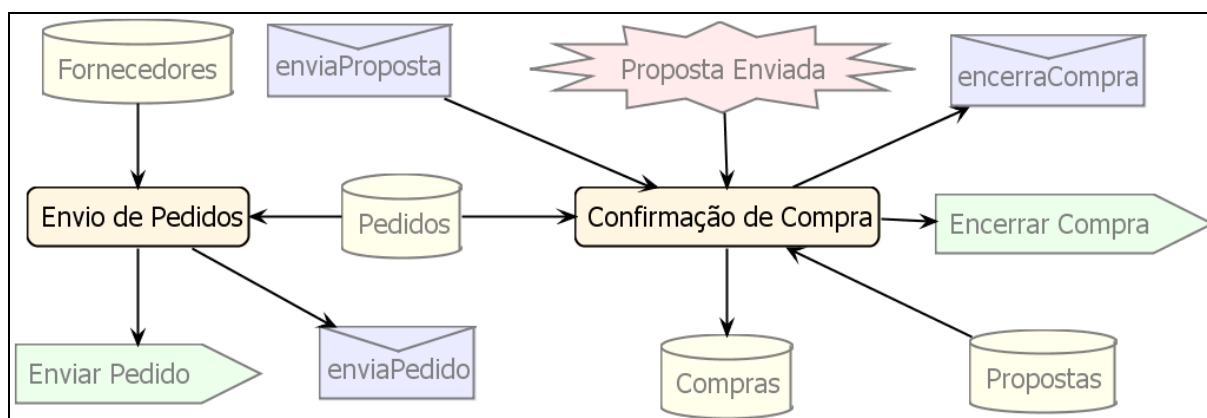
Figura 2.11 – Diagrama de Visão Geral do Agente - Agente de Compras.
