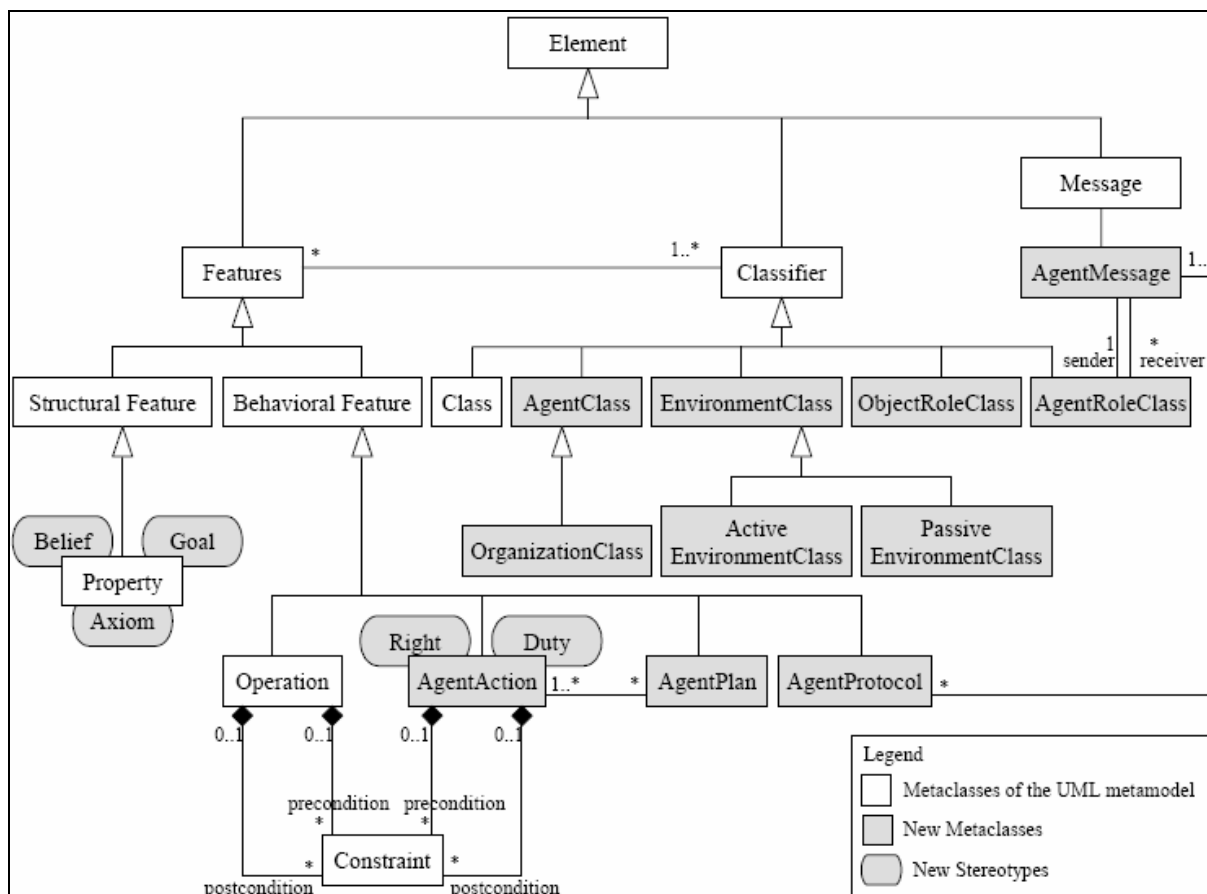
Figura 2.13 – Meta-modelo TAO/MAS-ML [SIL04a].
