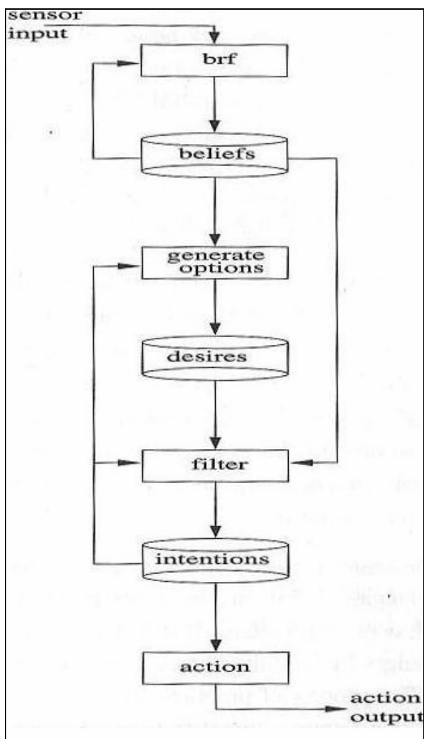
Figura 2.3 – Diagrama esquemático de uma arquitetura BDI genérica [WEI01].
