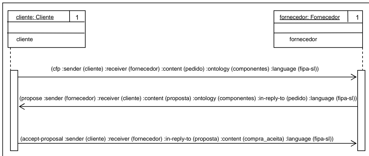
Figura 5.2 – Comunicação entre os agentes do exemplo modelado.
