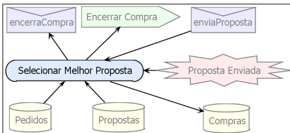
Figura 2.12 – Diagrama de Capacidade - Confirmação de Compra do Agente de Compras.
