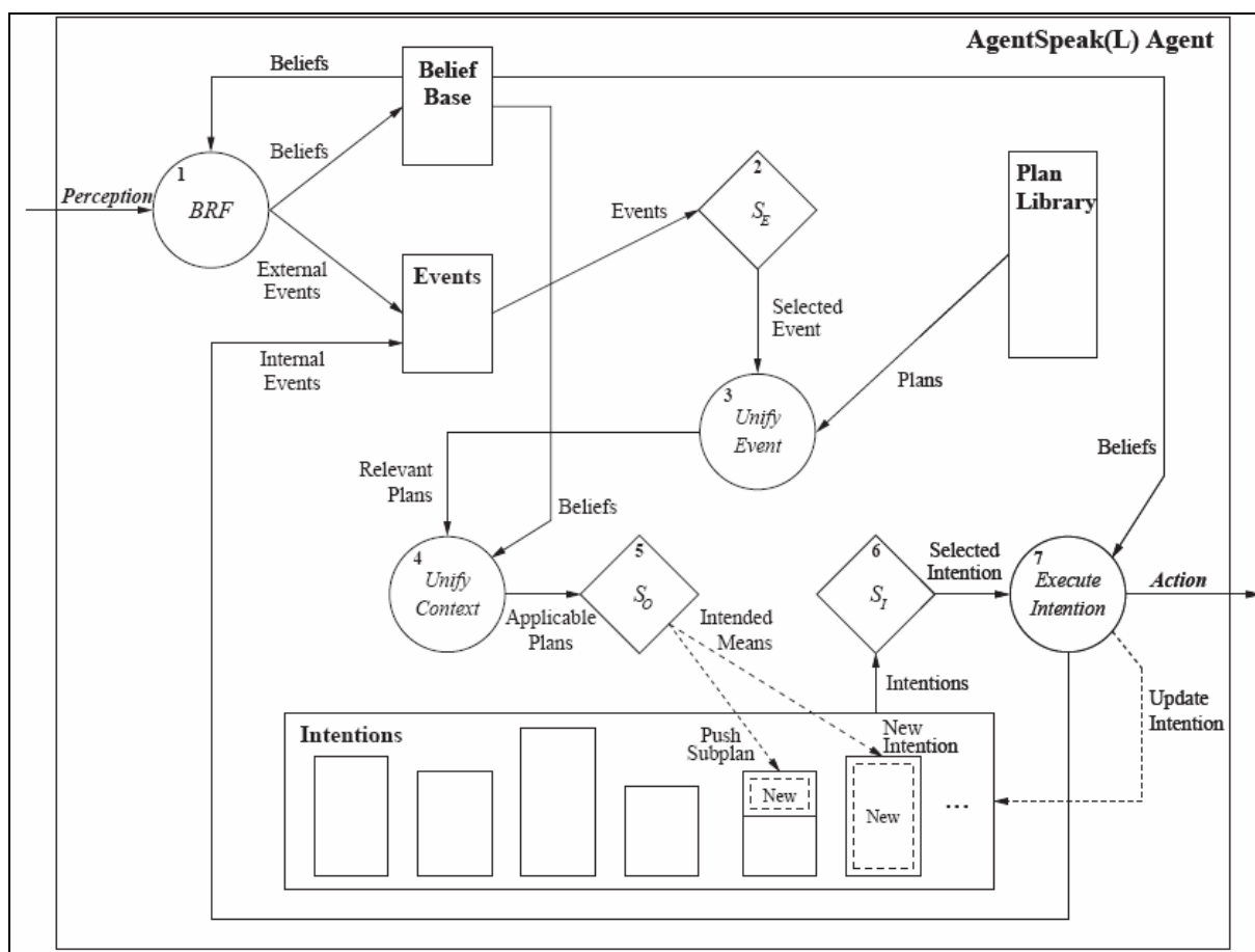
Figura 2.18 – Ciclo de Interpretação de um Programa AgentSpeak [MAC02].
