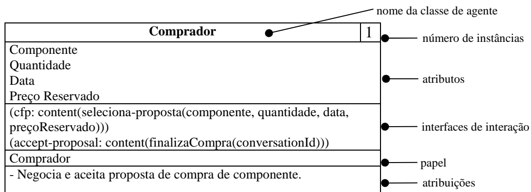
Figura 2.5 – Especificação de uma Classe de Agente.
