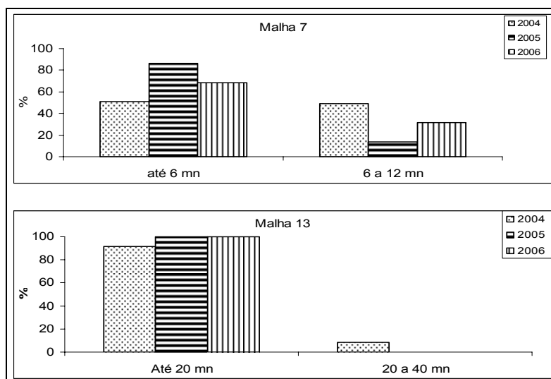
Figura 52 – Proporção anual da ocorrência de guavira em redes com malha 7 e com malha 13, por distância da costa, na frota de emalhe com desembarque em Santos, amostrada de 2004 a 2006.
