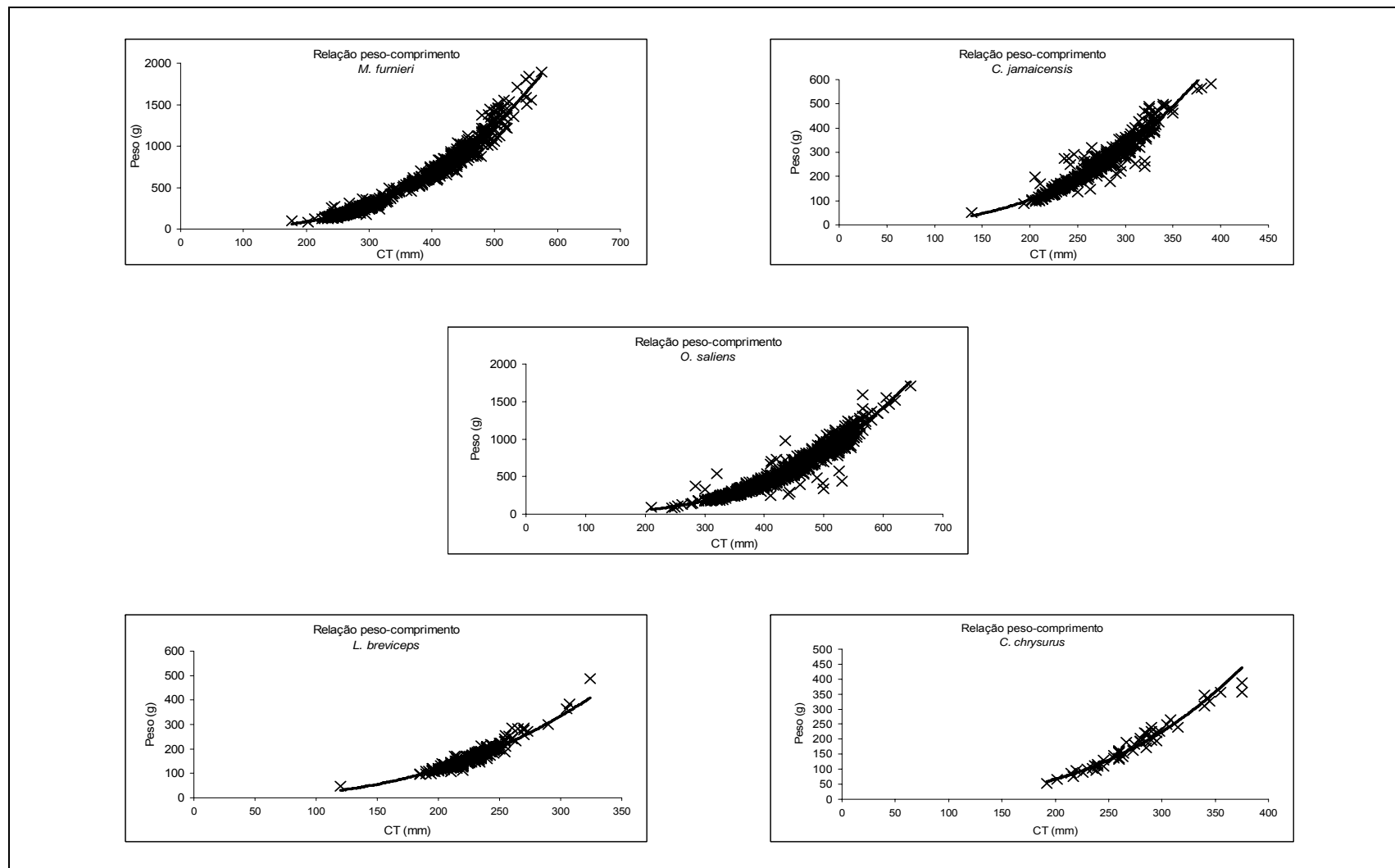
Figura 102a – Relações comprimento-peso das principais espécies capturadas na pesca de emalhe.
