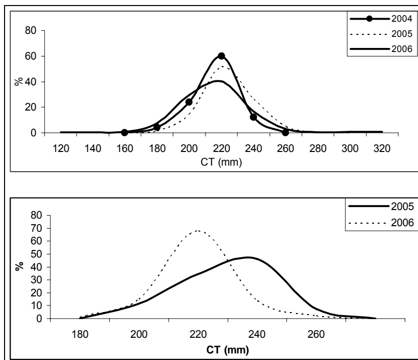
Figura 67 – Freqüências de comprimento de ovela com dados de malhas agrupadas e com dados isolados, amostrada de 2004 a 2006 nos desembarques da frota de emalhe em Santos.
