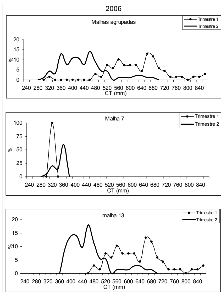
Figura 83 - Freqüência trimestral de comprimento de sororoca amostrada em 2006 nos desembarques da frota de emalhe em Santos.
