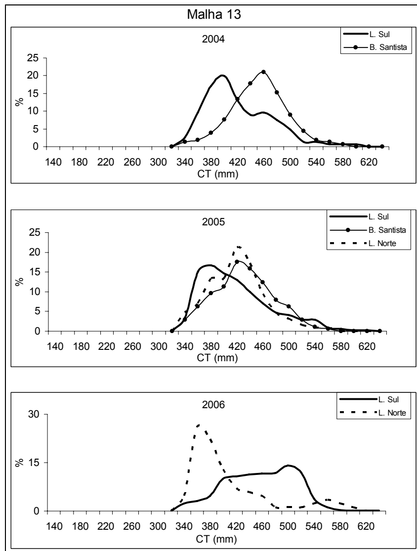
Figura 49 - Frequência de comprimento de guavira com malha 13, por área de pesca, amostrada de 2004 a 2006 nos desembarques da frota de emalhe em Santos.
