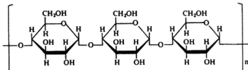
Figura 3. Estrutura molecular da amilose.
