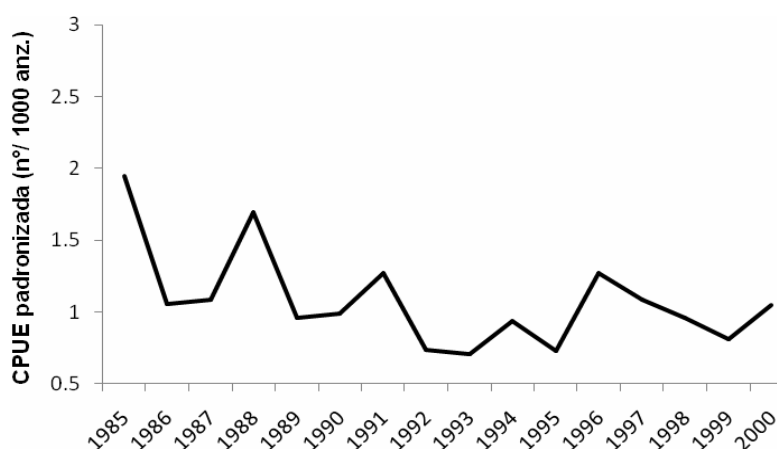
Figura 20 - Índice de abundância padronizado de tubarão-azul capturado no oeste do Atlântico Sul pela frota atuneira brasileira, estimado a partir dos coeficientes da variável “ano” do modelo Log-normal.
