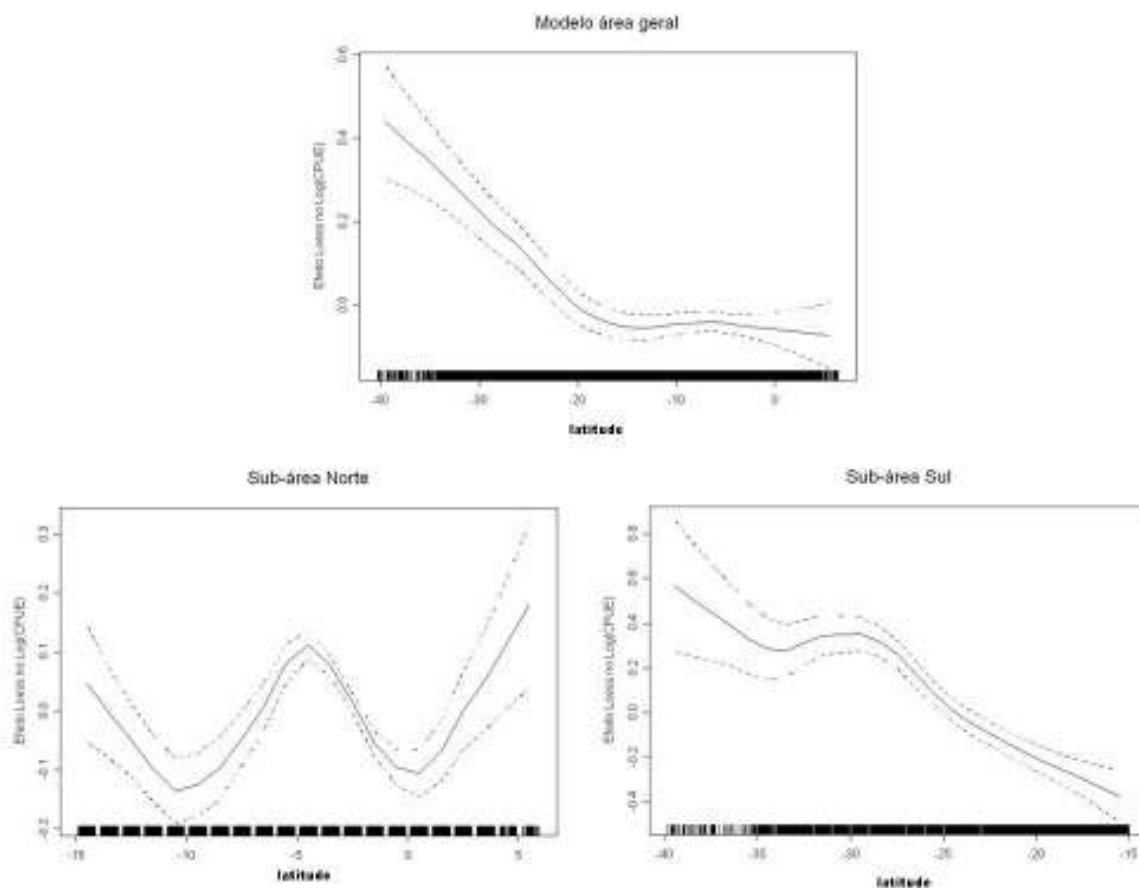
Figura 28 - Efeito da “latitude” sobre a abundância relativa de tubarão-azul, derivado de um modelo aditivo generalizado. As linhas pontilhadas representam o intervalo de confiança das estimativas.
