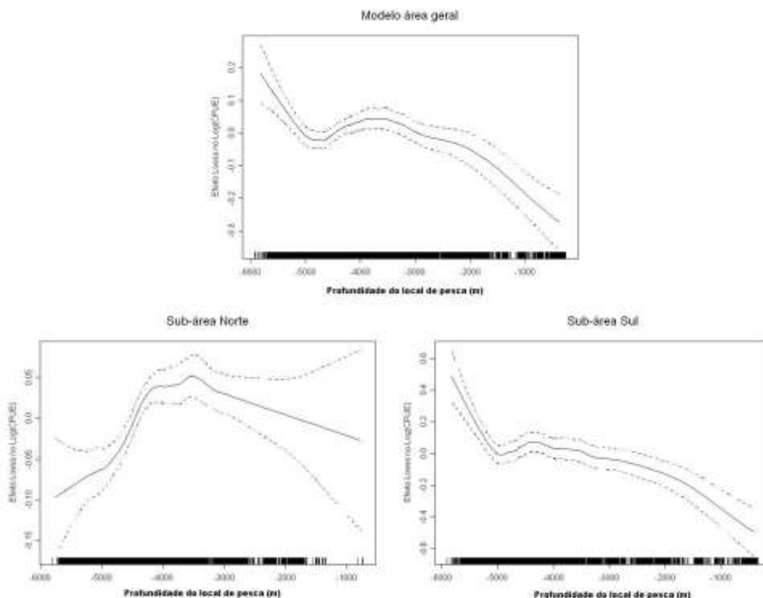
Figura 29 - Efeito da “profundidade do local de pesca” sobre a abundância relativa de tubarão-azul, derivado de um modelo aditivo generalizado. As linhas pontilhadas representam o intervalo de confiança das estimativas.
