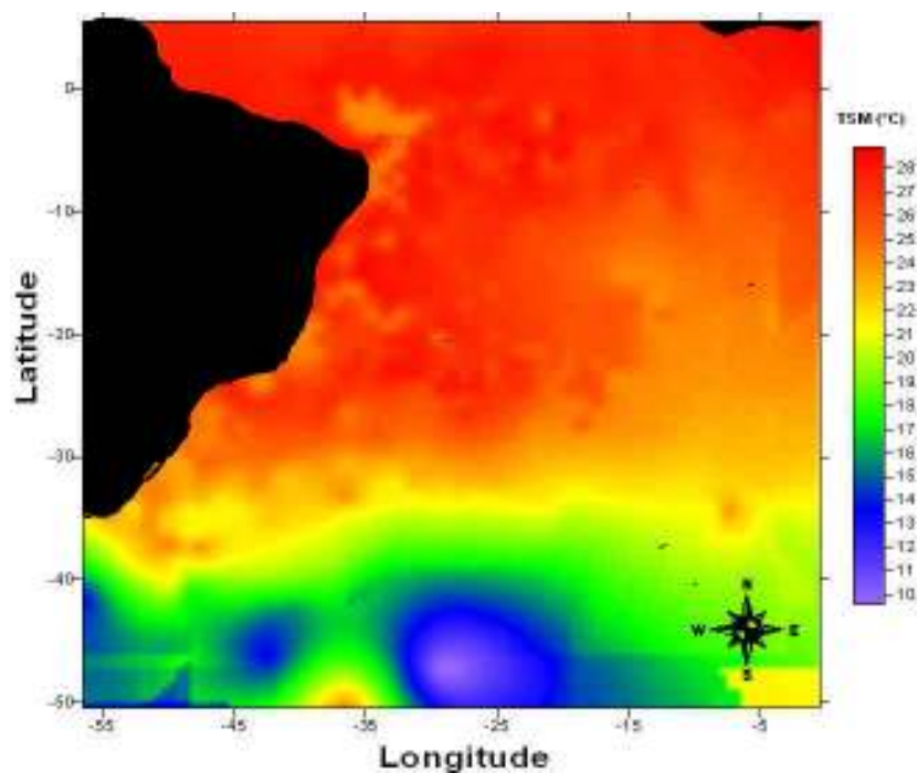
Figura 33 - Distribuição espacial da média de temperatura da superfície do mar no primeiro trimestre do ano, para o período 1985 - 2000.
