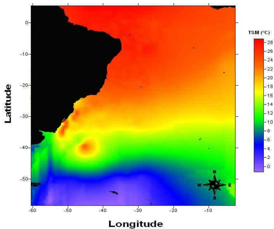
Figura 35 – Distribuição espacial da média de temperatura da superfície do mar no terceiro trimestre do ano, para o período 1985 - 2000.
