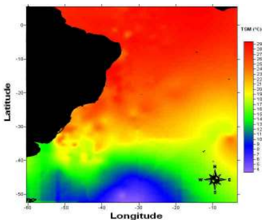
Figura 34 – Distribuição espacial da média de temperatura da superfície do mar no segundo trimestre do ano, para o período 1985 - 2000.
