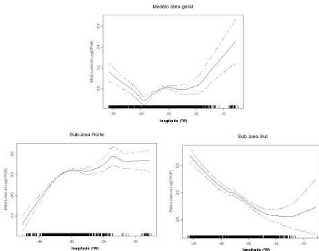
Figura 27 - Efeito da “Longitude” sobre a abundância relativa de tubarão-azul, derivado de um modelo aditivo generalizado. As linhas pontilhadas representam o intervalo de confiança das estimativas.
