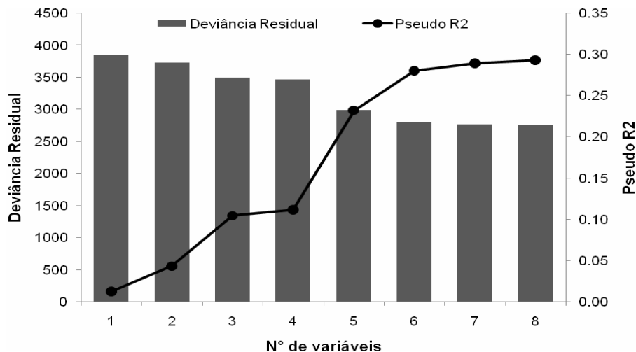
Figura 24 – Relação do número de variáveis com a deviança residual e o pseudo-r^2 do modelo aditivo generalizado para a sub-área sul.
