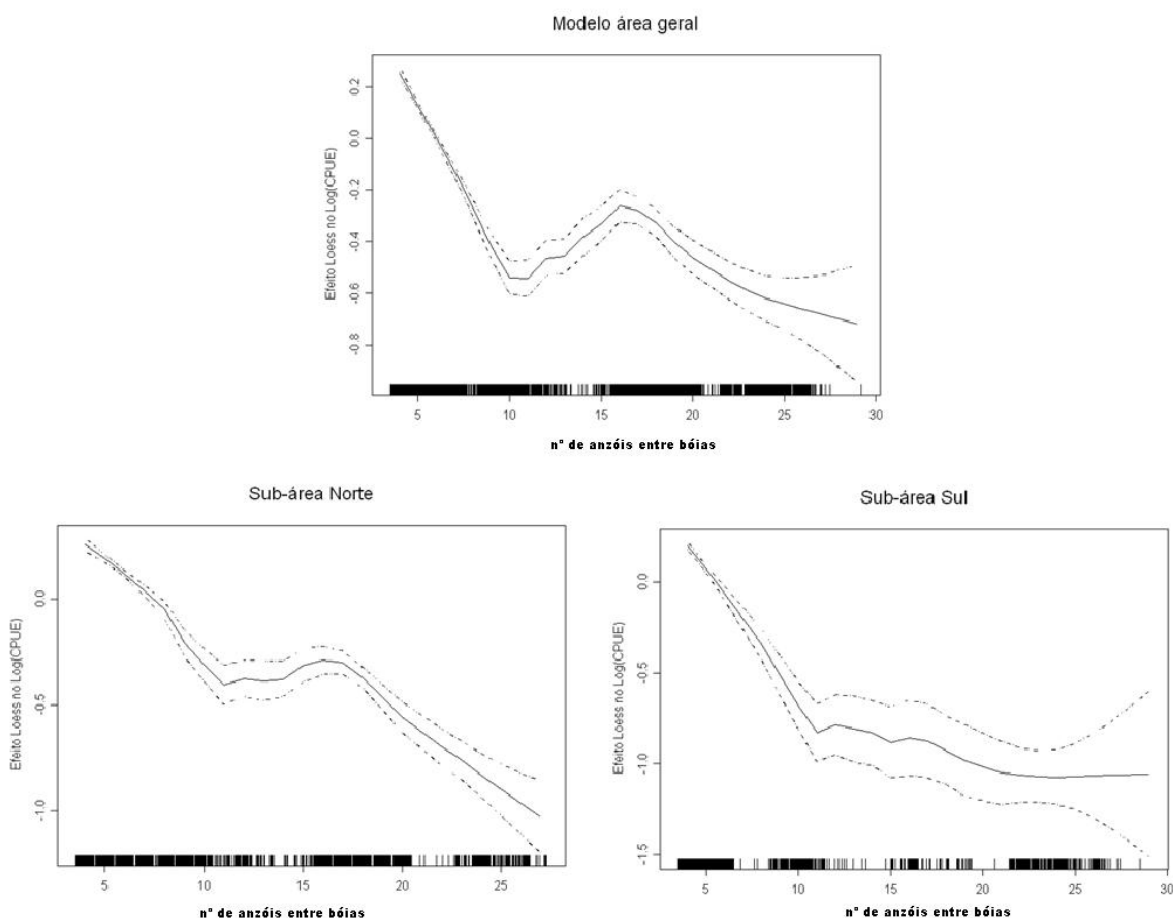
Figura 31 - Efeito do “nº. de anzóis entre bóias” sobre a abundância relativa de tubarão-azul, derivado de um modelo aditivo generalizado. As linhas pontilhadas representam o intervalo de confiança das estimativas.
