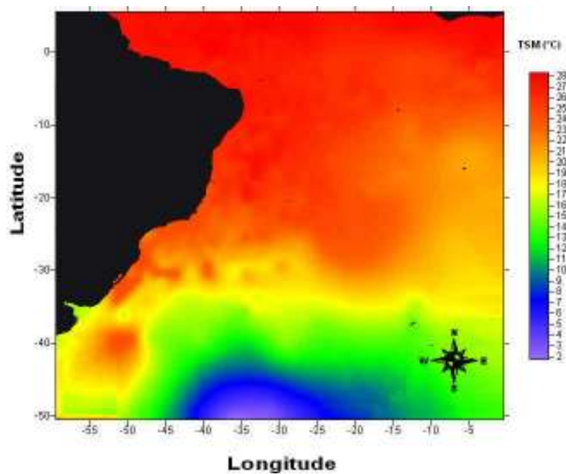
Figura 36 – Distribuição espacial da média de temperatura da superfície do mar no quarto trimestre do ano, para o período 1985 - 2000.
