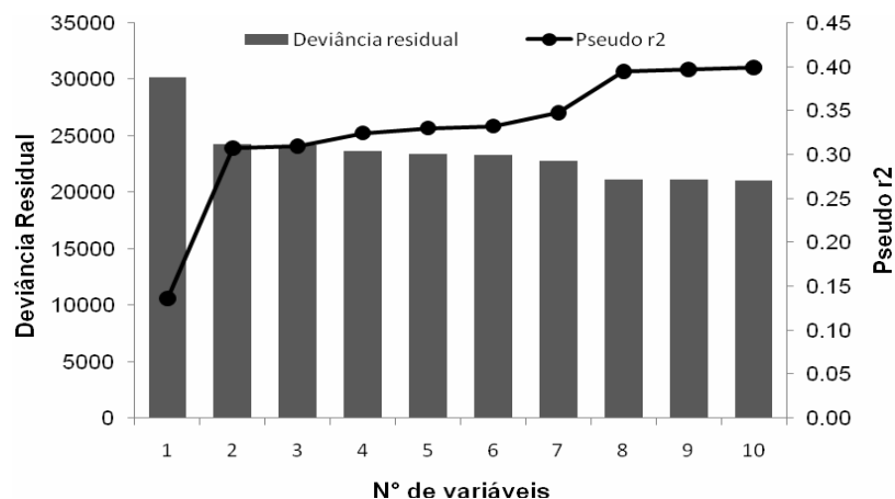
Figura 18 - Relação do número de variáveis com a deviança residual e o pseudo-r^2 do modelo aditivo generalizado referente ao modelo Binomial.
