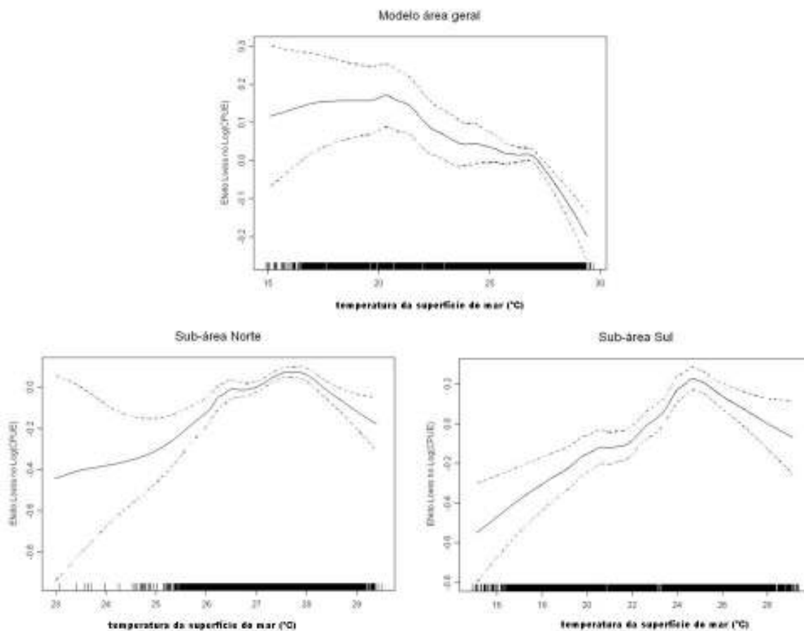
Figura 32 - Efeito da “temperatura da superfície do mar” sobre a abundância relativa de tubarão-azul, derivado de um modelo aditivo generalizado. As linhas pontilhadas representam o intervalo de confiança das estimativas.
