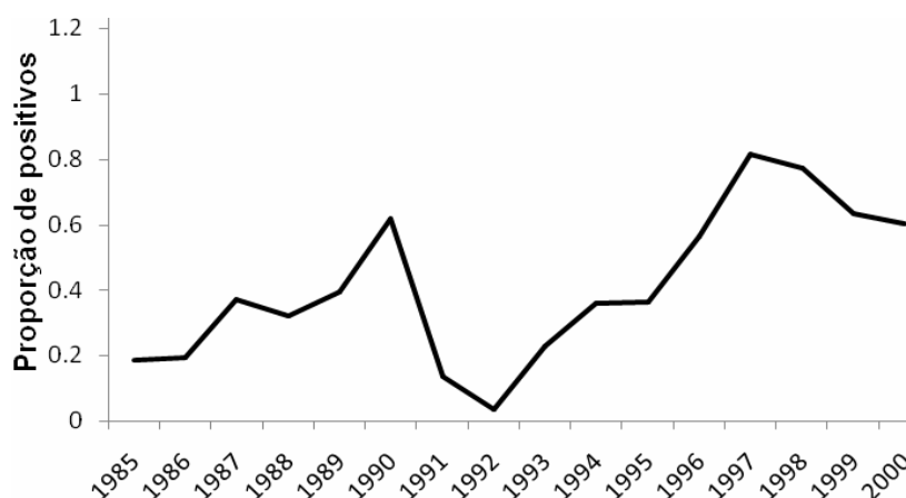
Figura 21 – Índice de abundância padronizado de tubarão-azul capturado no oeste do Atlântico Sul pela frota atuneira brasileira, estimado a partir dos coeficientes da variável “ano” do modelo Binomial.
