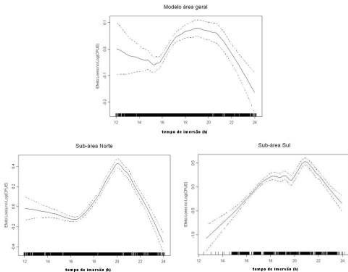
Figura 30 - Efeito do “tempo de imersão” sobre a abundância relativa de tubarão-azul, derivado de um modelo aditivo generalizado. As linhas pontilhadas representam o intervalo de confiança das estimativas.
