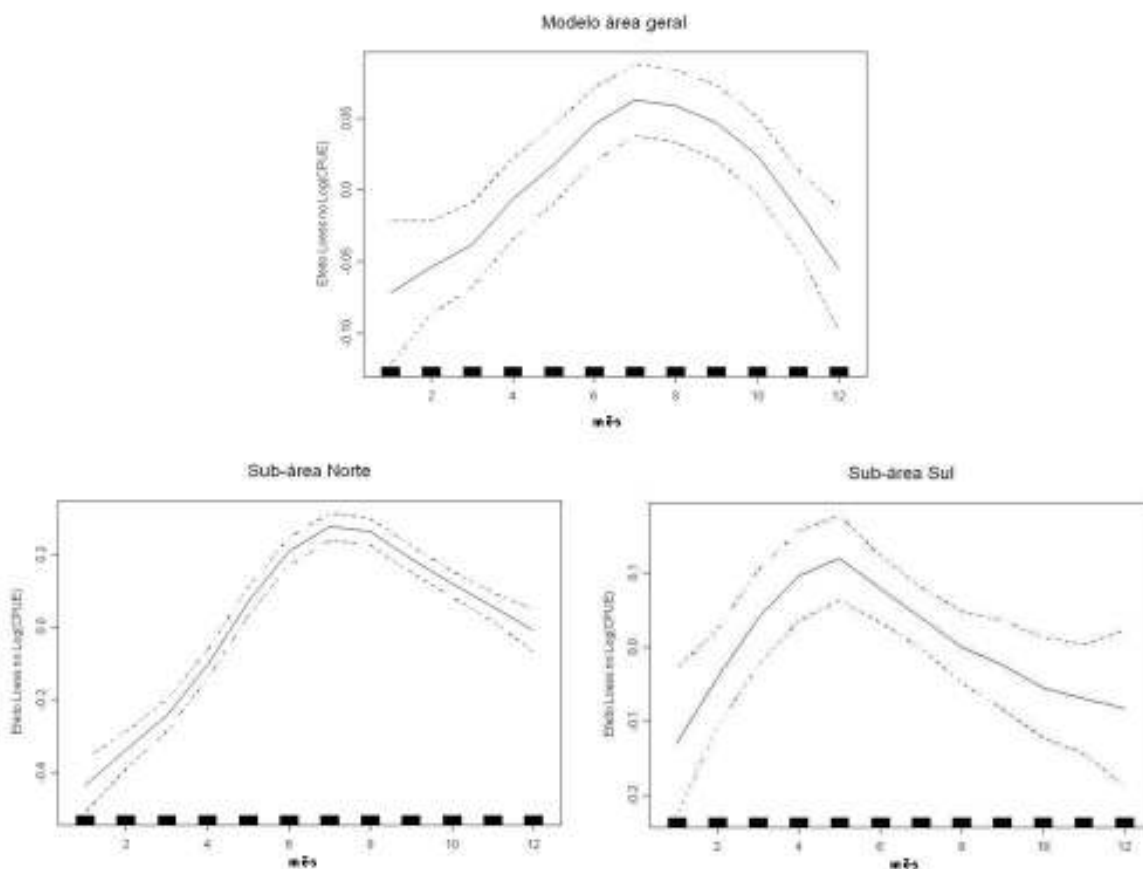
Figura 26 – Efeito de “mês” sobre a abundância relativa de tubarão-azul, derivado de um modelo aditivo generalizado. As linhas pontilhadas representam o intervalo de confiança das estimativas.
