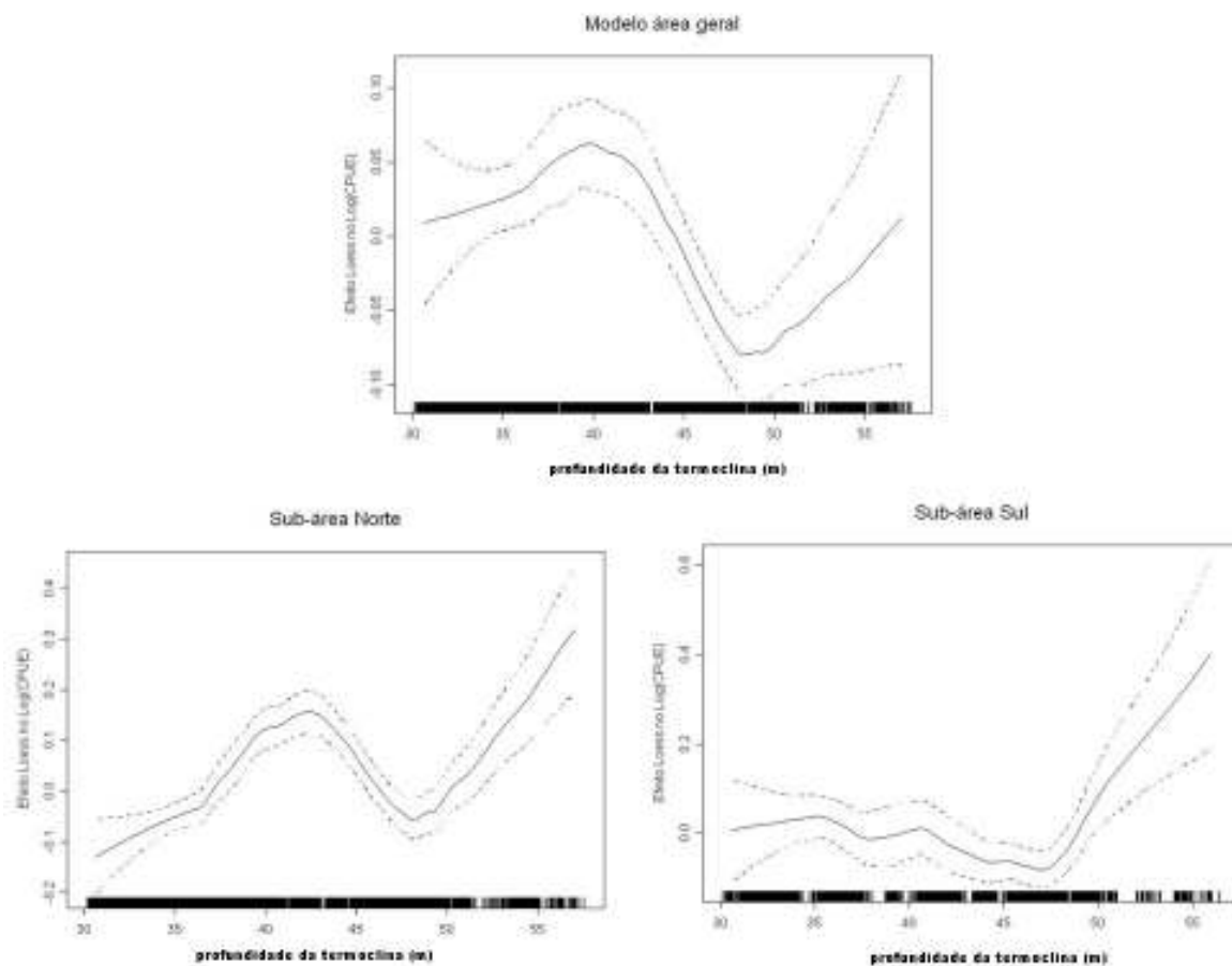
Figura 37 - Efeito da “profundidade da termoclina” sobre a abundância relativa de tubarão-azul, derivado de um modelo aditivo generalizado. As linhas pontilhadas representam o intervalo de confiança das estimativas.
