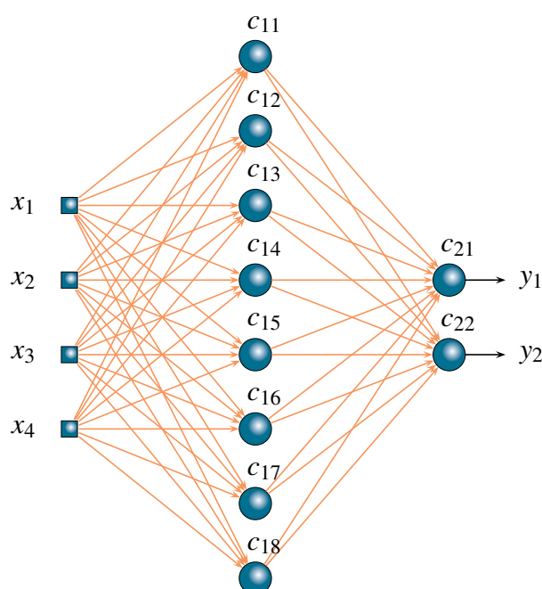
Figura 3.6: Exemplo de rede neural feedforward totalmente conectada com duas camadas.
