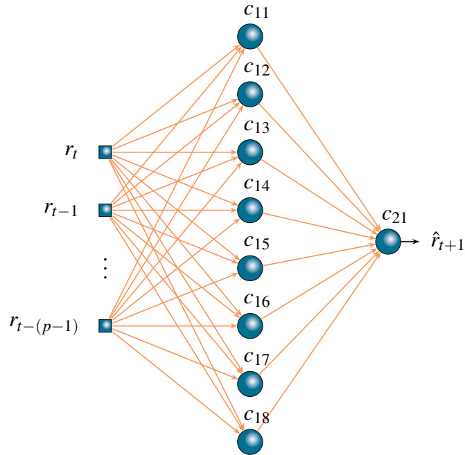
Figura 3.8: Rede Neural Auto-regressiva com duas camadas.
