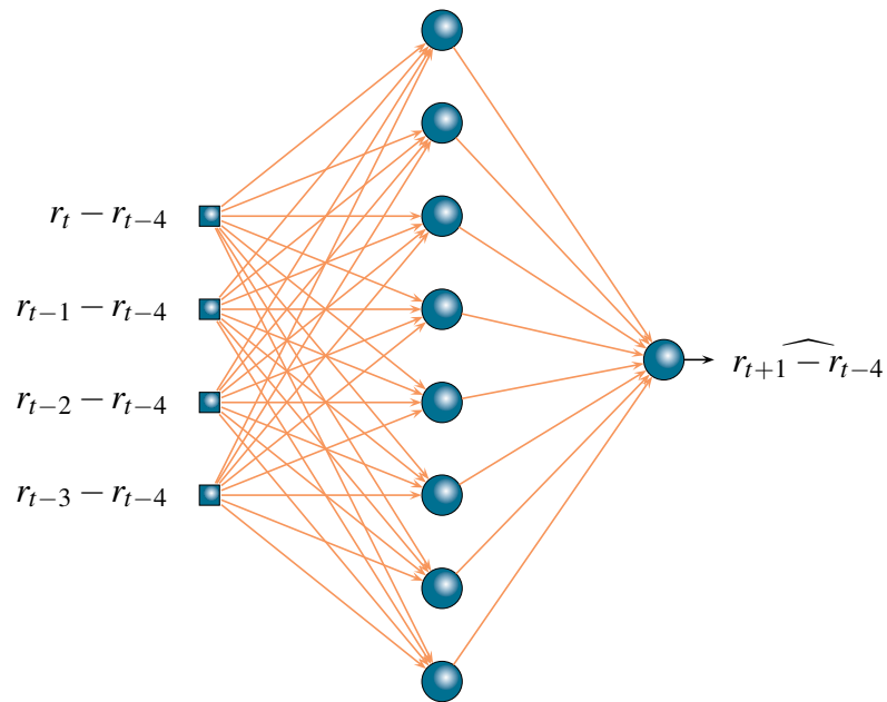
Figura 4.2: Exemplo de um preditor RNAR-RM (4,1).
