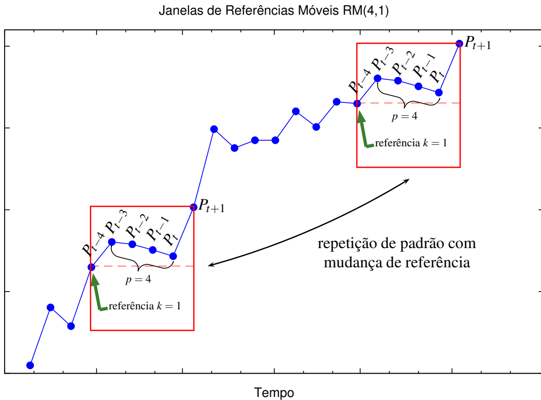
Figura 4.1: Aplicação do método das referências móveis no preditor RNAR-RM (4,1). No tempo t , a referência é dada pelo valor de P_{t-4} , e as entradas da rede são P_{t-3} - P_{t-4} , P_{t-2} - P_{t-4} , P_{t-1} - P_{t-4} , e P_t - P_{t-4} . Os padrões das janelas de referências móveis repetidas podem ser codificados nos pesos da rede neural apenas uma única vez.
