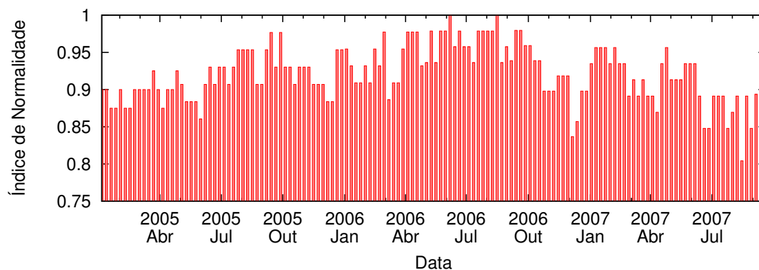
(a) Índices de Normalidade para as séries de erros de previsão
