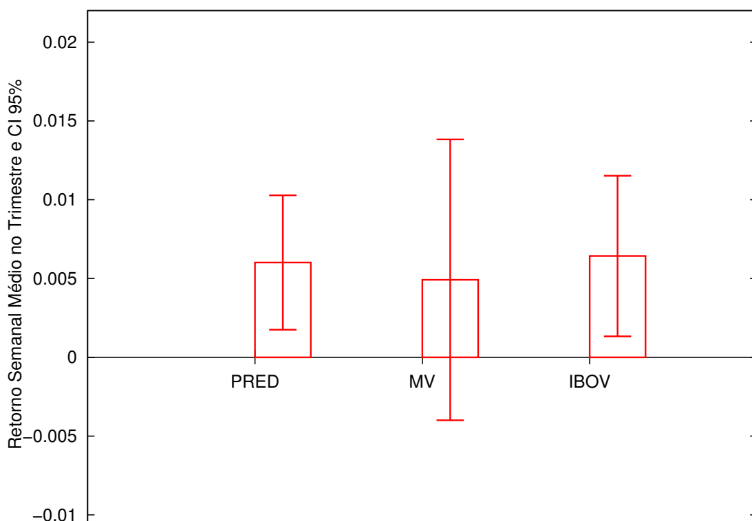
Figura 6.7: Simulação de investimento de baixo risco. Intervalos de confiança (CI) de 95% dos retornos semanais médios no trimestre para o modelo de seleção de carteiras baseado em erros de previsão (PRED), para o modelo média-variância (MV) e para o índice IBOVESPA durante as 142 semanas do período de investimento. O menor risco apresentado pelo modelo de seleção de carteiras baseado em erros de previsão é evidenciado pelo seu menor erro padrão da média, mostrado nas barras verticais.
