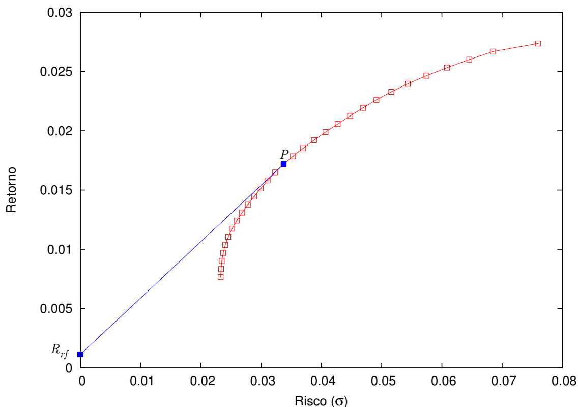
Figura 6.8: Exemplo de uma Fronteira Eficiente com ativo sem risco. Todas as combinações da participação no ativo sem risco com retorno esperado R_{rf} e da participação na carteira P , ao longo da tangente que os conecta, são eficientes.
