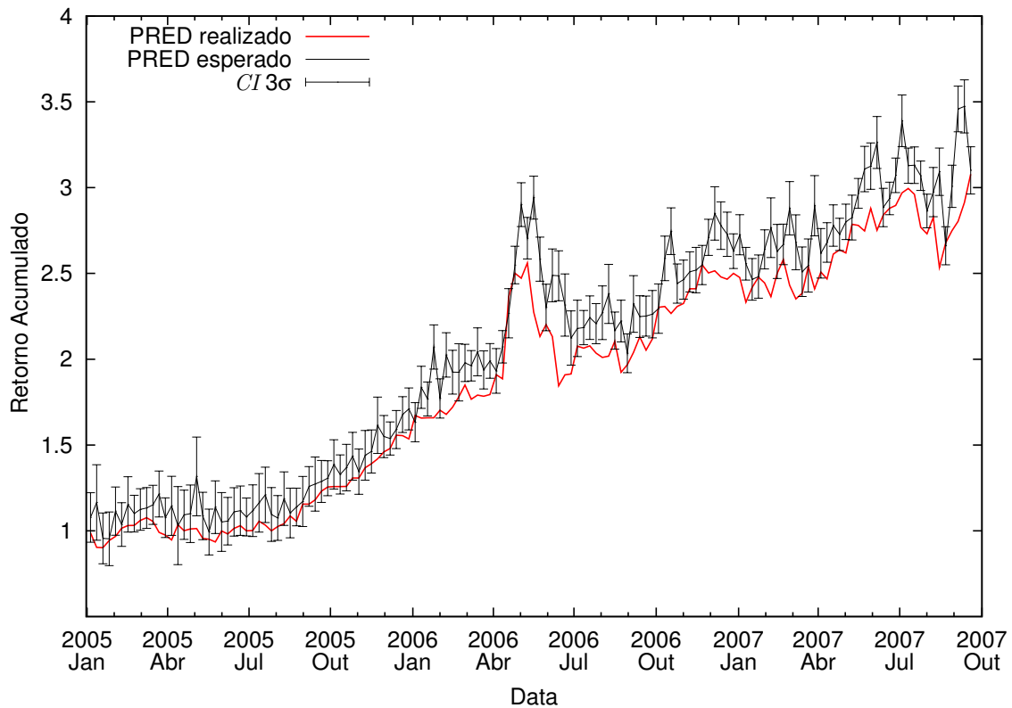
(a) Retornos acumulados e CI\ 3\sigma para o modelo de seleção de carteiras baseado em erros de previsão
