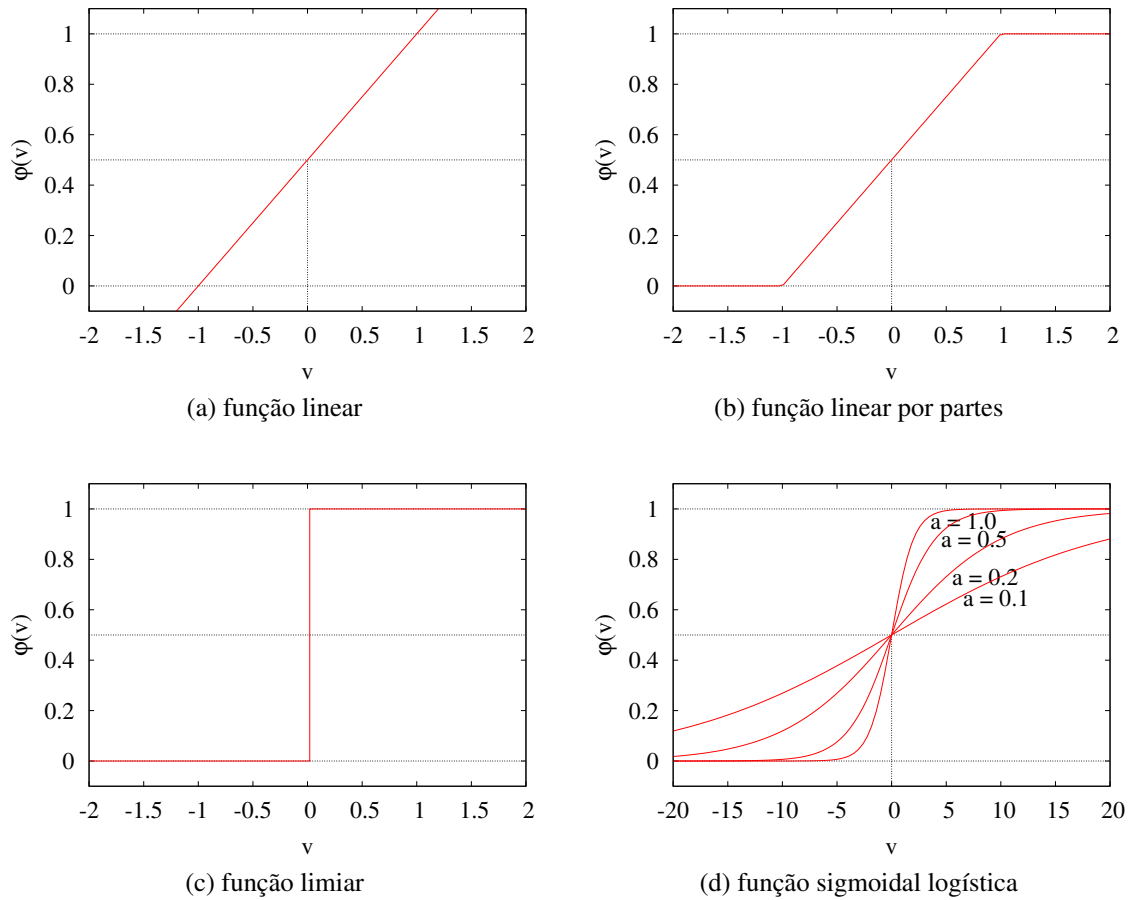
Figura 3.4: Exemplos de algumas funções de ativação. A função linear (a), a função linear por partes (b), a função limiar (c) e a função sigmoidal logística (d).
