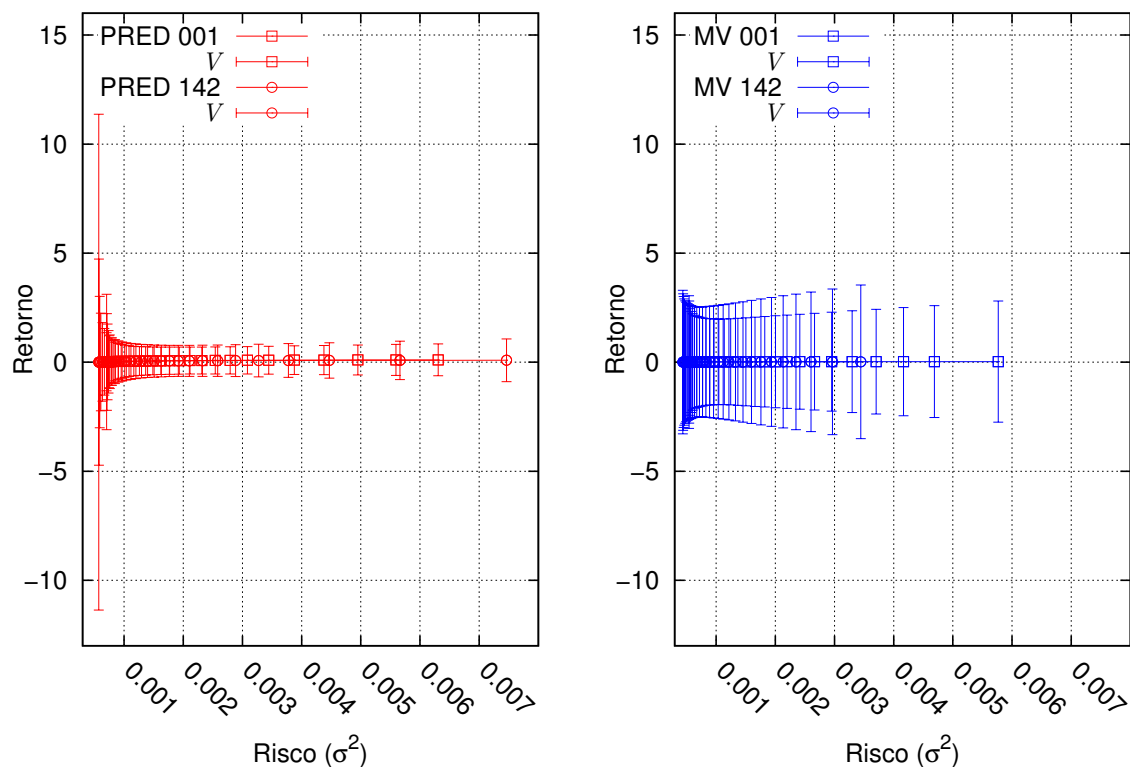
(a) Fronteiras Eficientes e coeficientes de variação para o modelo de seleção de carteiras baseado em erros de predição
