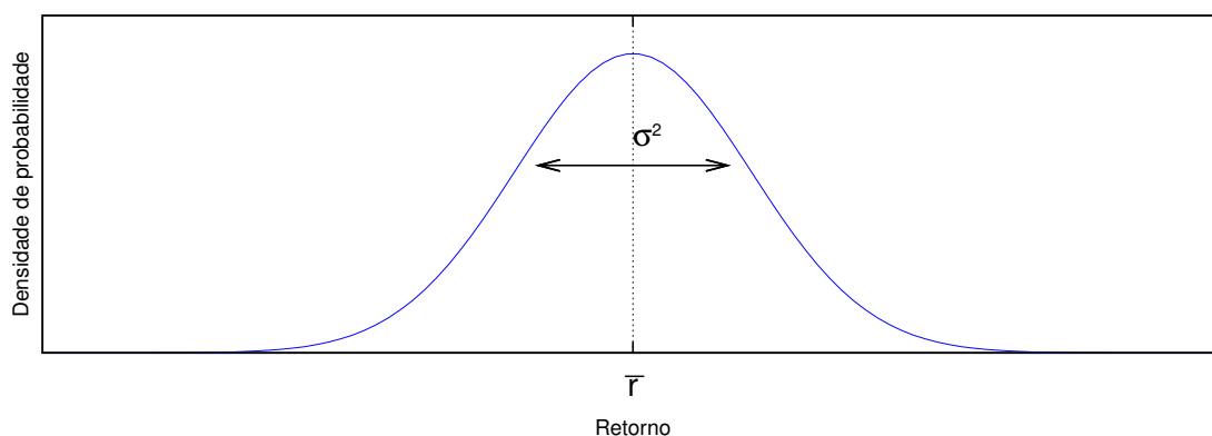
(b) Distribuição dos retornos das ações para o modelo média-variância
