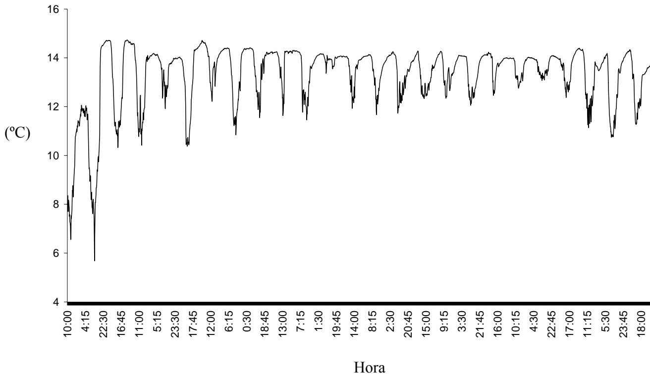
Figura 32 - Variação da diferença de temperatura registrada entre as sondas de dissipação térmica instaladas em uma mesma muda cítrica. Cada patamar corresponde a um dia. Piracicaba, 2007
