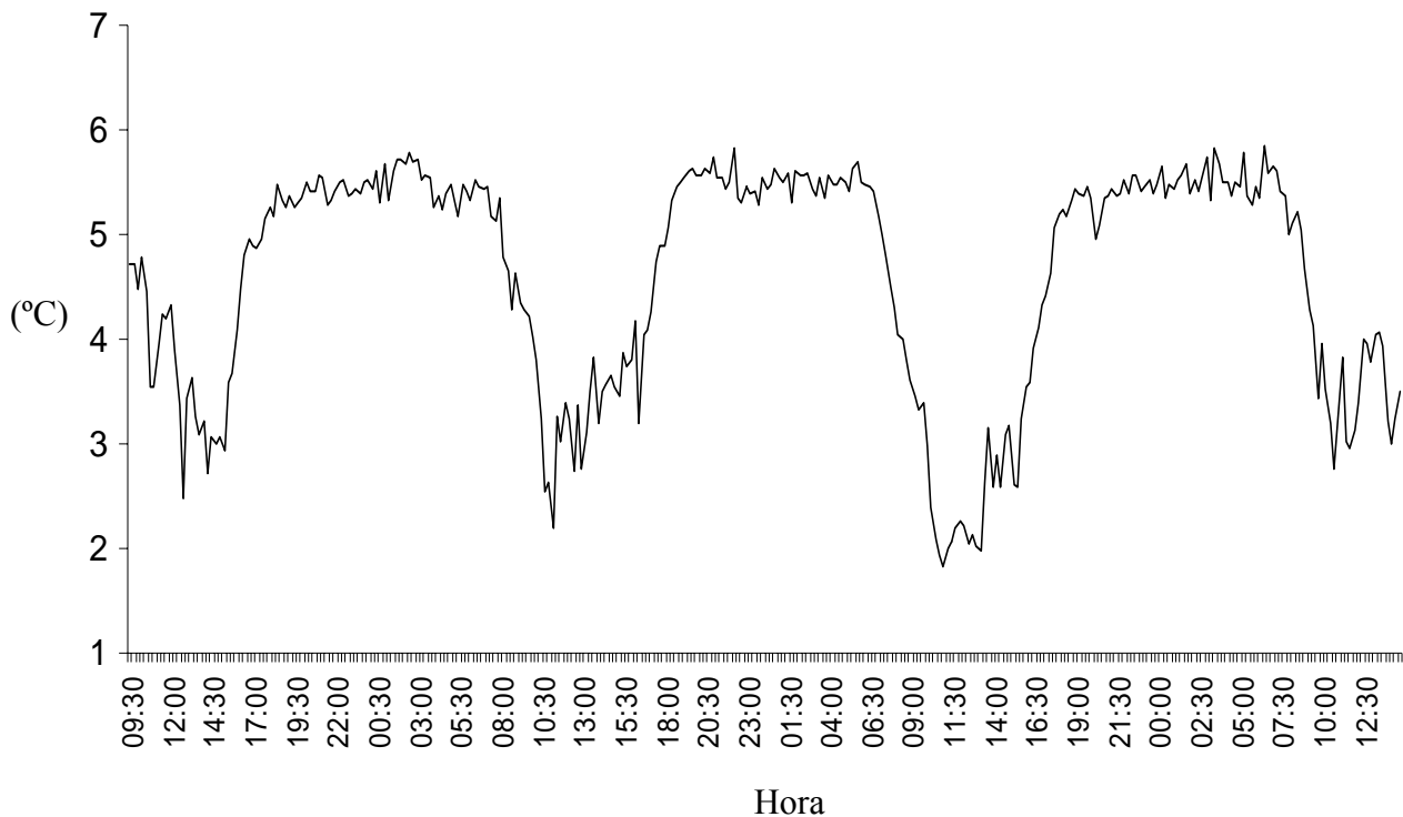
Figura 33 - Variação da diferença de temperatura registrada entre sondas de dissipação térmicas instaladas em uma mesma muda cítrica, em função da hora do dia. Patamares superiores correspondem ao período noturno (sem fluxo de seiva), depressão corresponde ao período diurno (seiva circulando). Piracicaba, 2007
