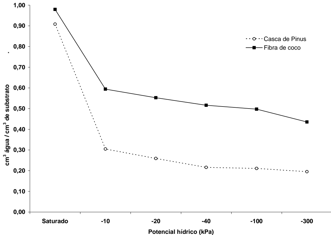
Figura 21 - Curva de retenção de água em substratos a base de casca de pinus e fibra de coco, utilizados para produção de mudas de citros. Araras, 2006
