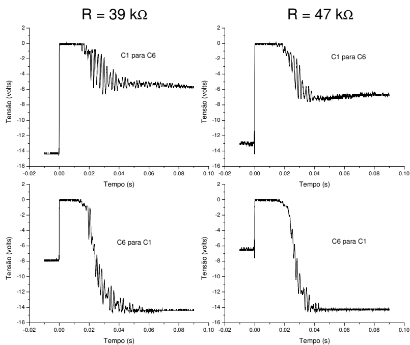
Figura 5.28: Sintonização dos lasers C1 - C6 usando resistores de 39 \text{ k}\Omega e 47 \text{ k}\Omega .
