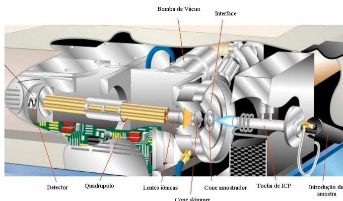
Figura 4.1. Subdivisões do espectrômetro de massas com plasma indutivamente acoplado ELAN 9000 PerkinElmer. Fonte: Adaptado de www.perkinelmer.com
