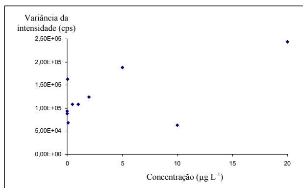
Figura 4.7. Comportamento homocedástico dos dados, para o elemento ^{57}\text{Fe} .
