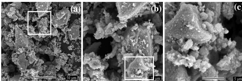
4 Figura 20. MEV da amostra \text{Sn}_{x_1} ampliado: (a) 500 x; (b) 2000 x; (c) 5000 x
