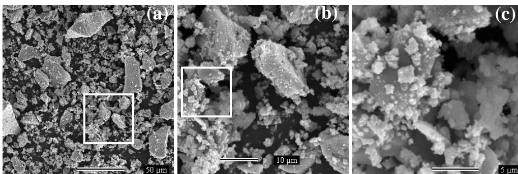
6 Figura 21. MEV da amostra \text{Sn}_{x_2} ampliado: (a) 500 x; (b) 2000 x; (c) 5000 x
