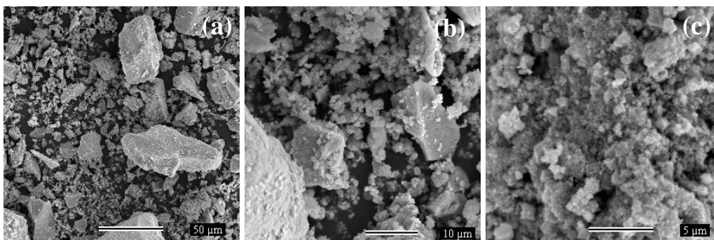
8 Figura 22. MEV da amostra \text{Sn}_{x_3} ampliado: (a) 500 x; (b) 2000 x; (c) 5000 x.
