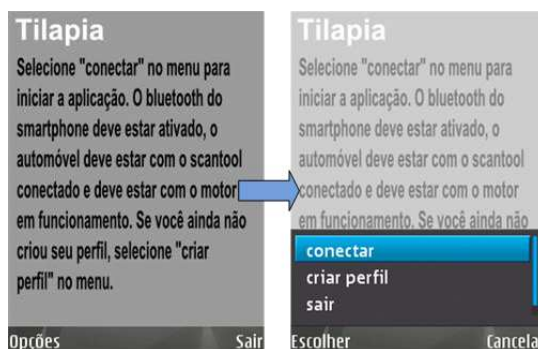
Figura 4.3: Menu inicial da interface gráfica com o usuário.
