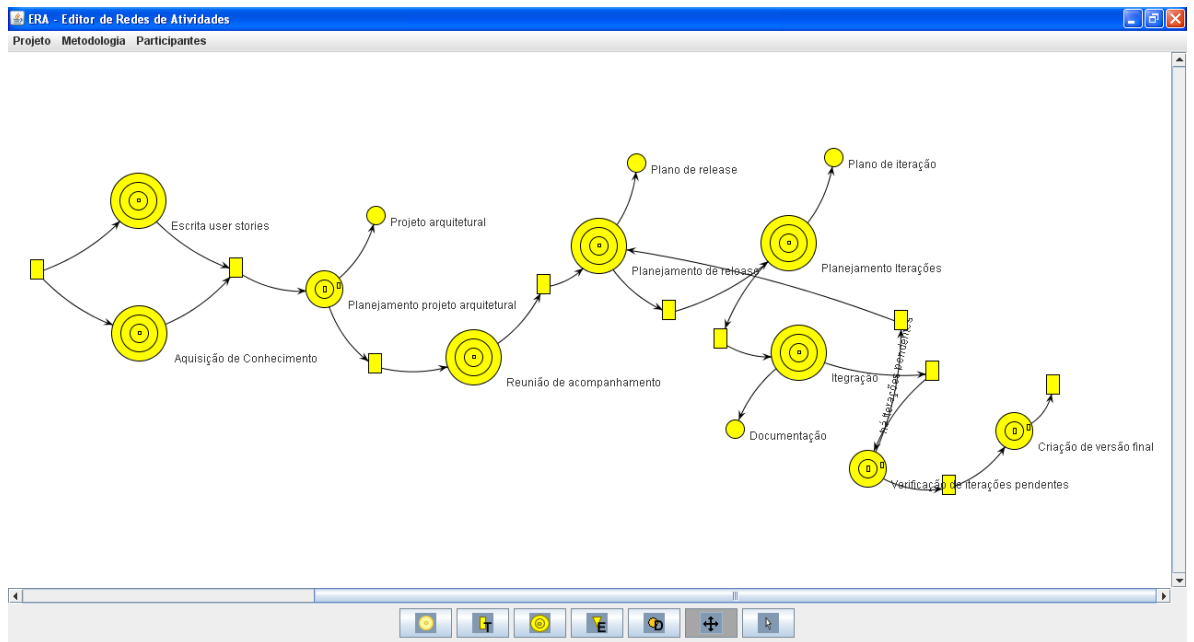
Figura 5.7. Rede de Atividades da metodologia XP1
