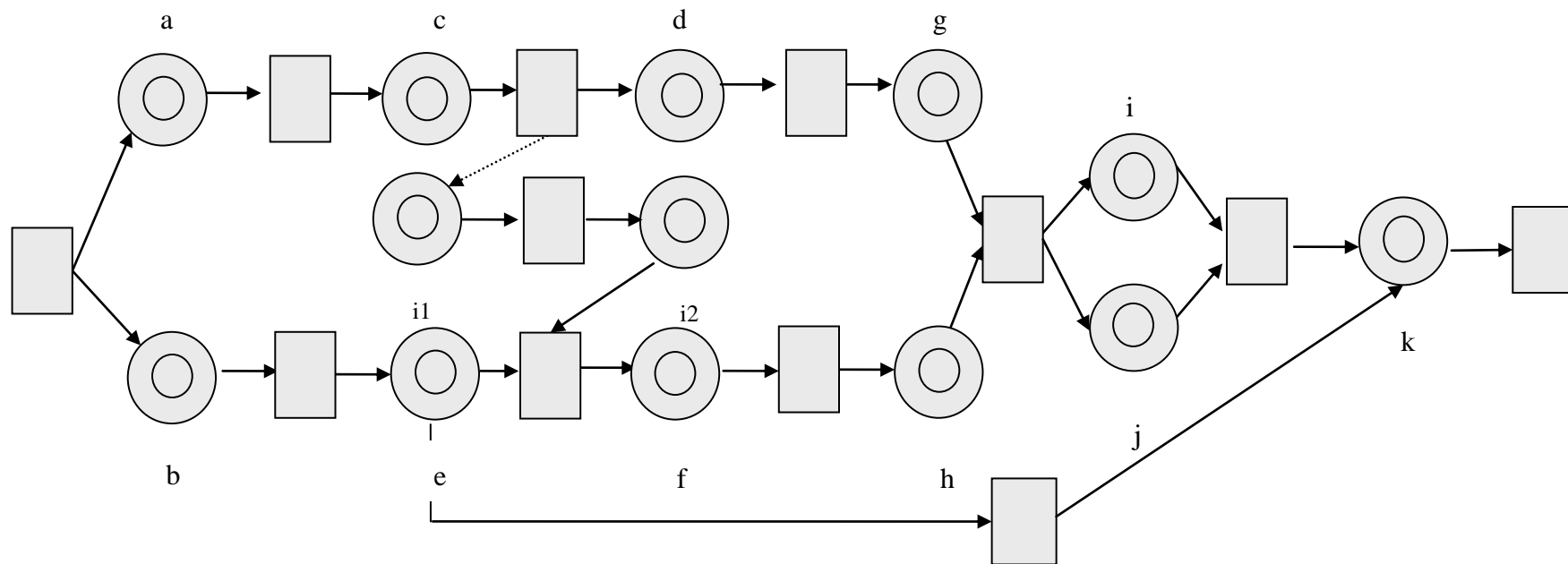
Figura 4.20.: Rede de Atividades de alto nível com encerramento do projeto na atividade 'e'.
