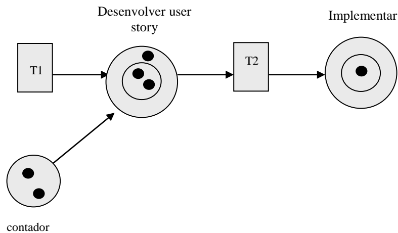
Figura 4.17.: Rede de Atividades Expandida
