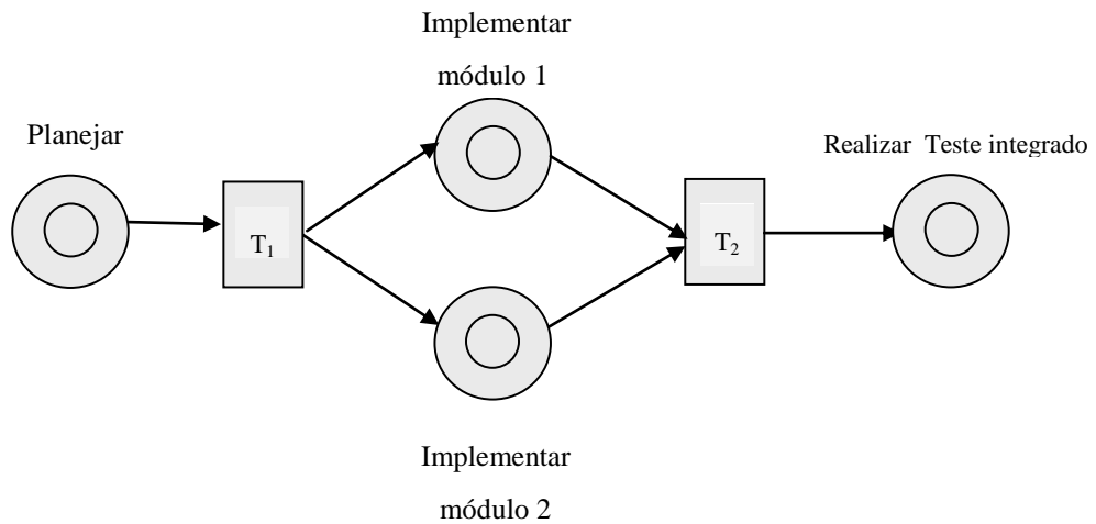
Figura 4.8: Rede de atividades com atividades paralelas
