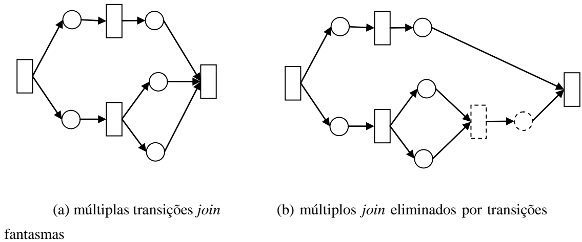
Figura 4.3: Eliminação de múltiplos joins
