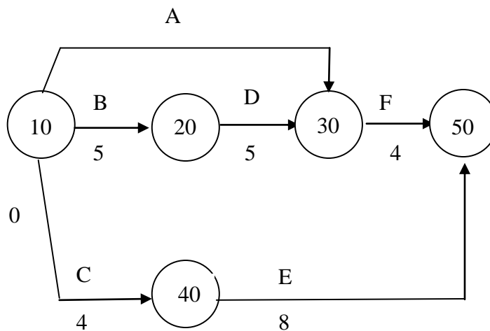
Figura 2.1: Representação de uma Rede PERT com determinação do caminho crítico
