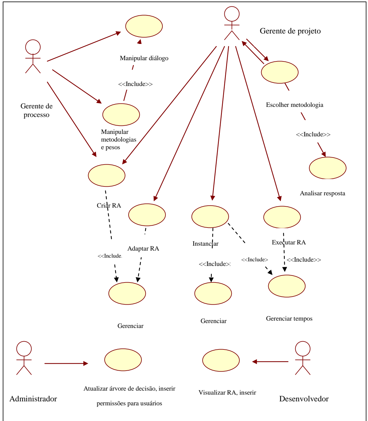
Figura 5.4: Diagrama de casos de uso – GDP
