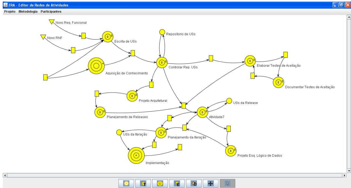
Figura 6.2: Tela de Rede de Atividades com visualização do primeiro nível da rede de XP1
