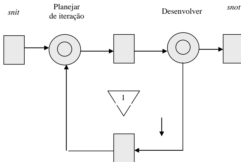
Figura 4.13: Subrede de “Desenvolver software” composta por duas iterações
