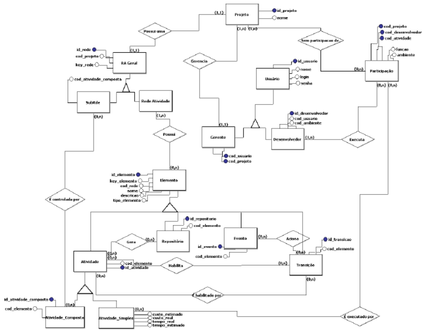
Figura 2: Modelo conceitual do ERA
