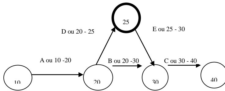
Figura 2.3: Diagrama de flechas para três atividades linearmente seqüenciais com inserção correta de uma atividade paralela
