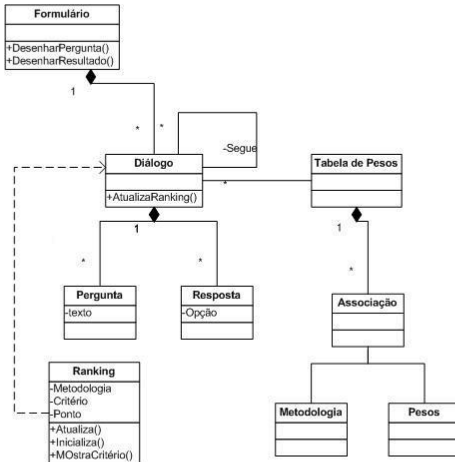
Figura 5.2: Diagrama de classes do SiSeM (Farias, 2005)
