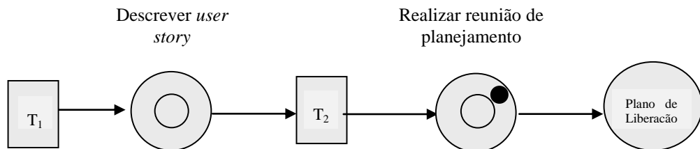
Ilustração 4.7: Rede de atividades com atividade “Realizar reunião de planejamento” finalizada
