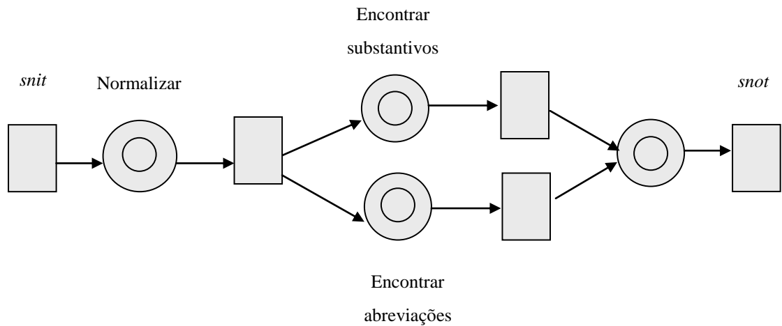
Figura 4.15: Decomposição da atividade “Indexar texto”.
