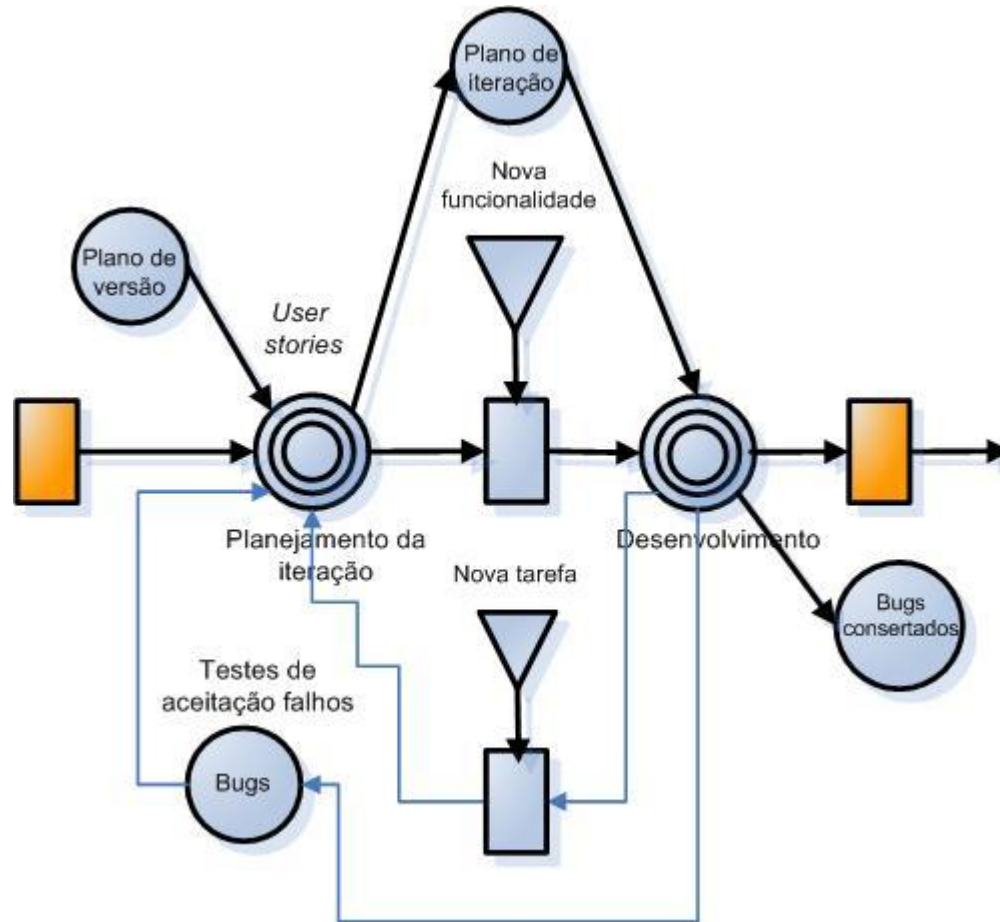
Figura 4.23: Sub-Rede da atividade composta “Planejar iteração” da Figura 4.21.
