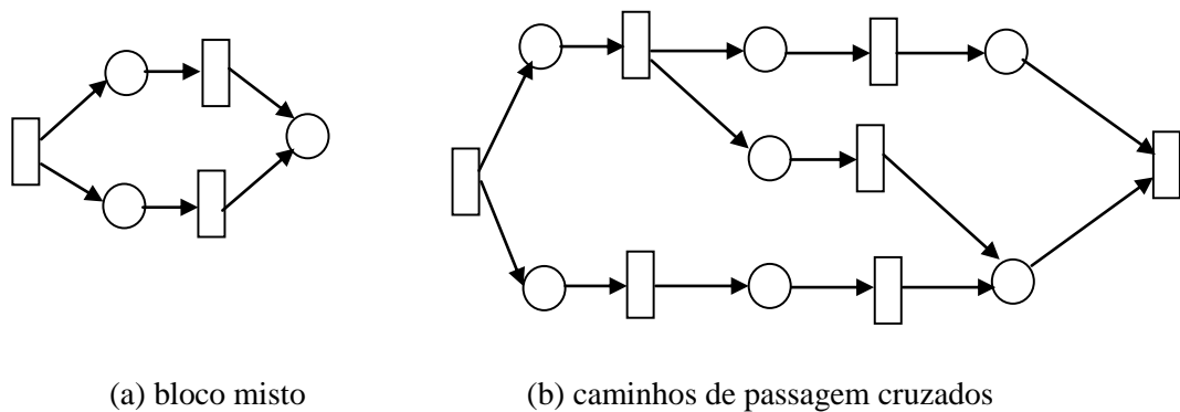
Figura 4.1: Estruturas de rede indesejadas
