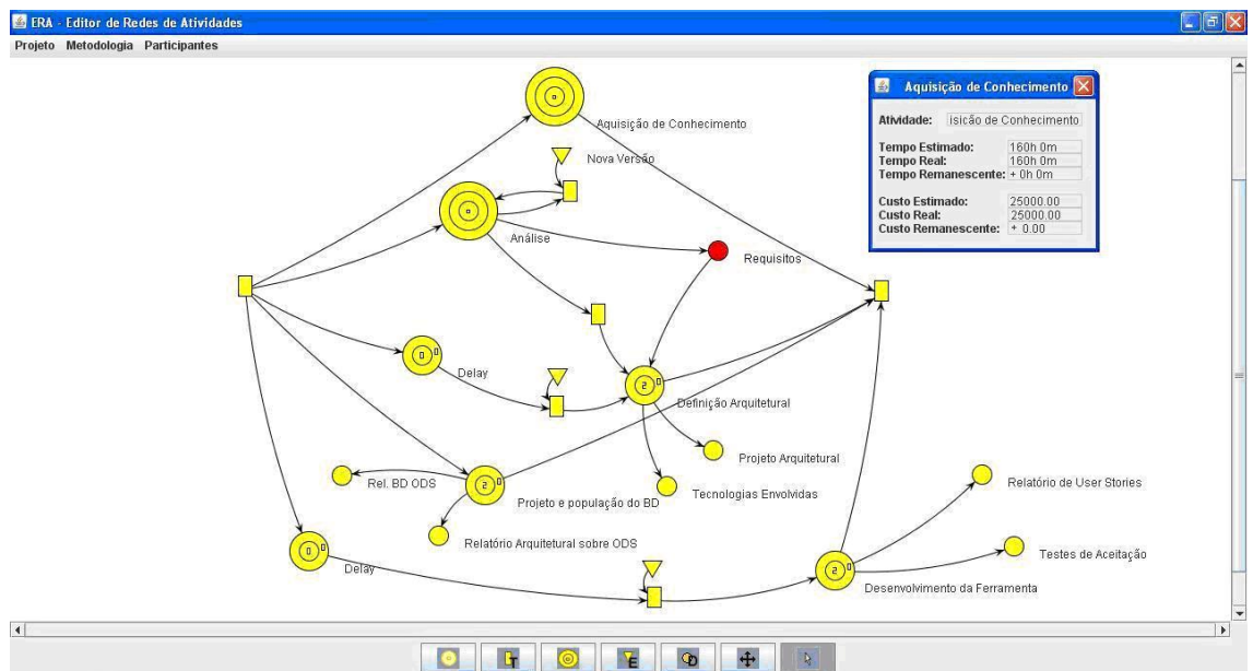
Figura 5.13: Totalização de valores de tempo e custo para a atividade “Aquisição de conhecimento”.
