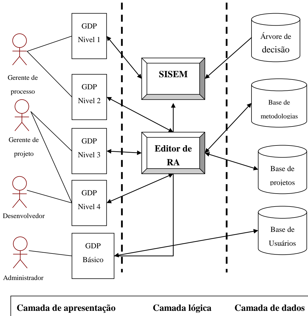
Figura 5.1: Arquitetura do sistema GDP
