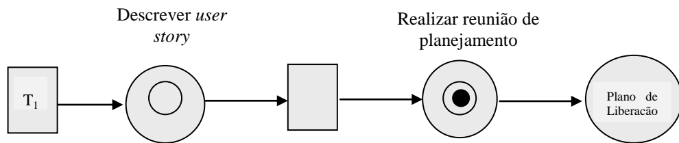
Figura 4.6: Rede de atividades com atividade “Realizar reunião de planejamento” em execução
