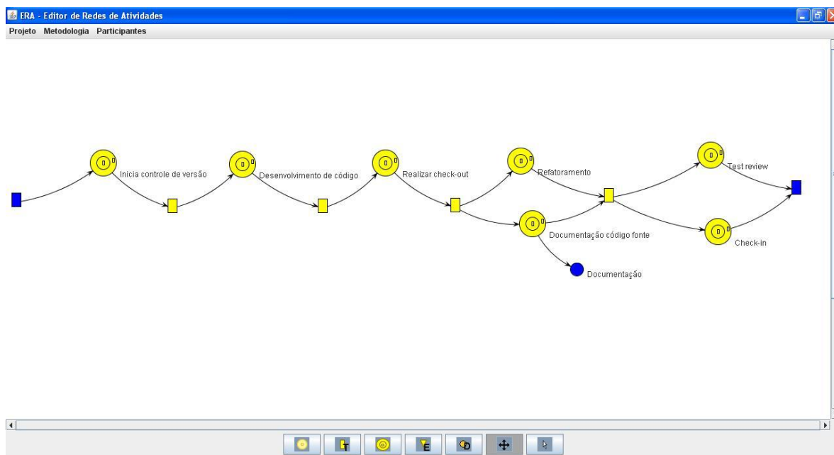
Figura 5.8. Sub-rede da etapa de integração de XP1
