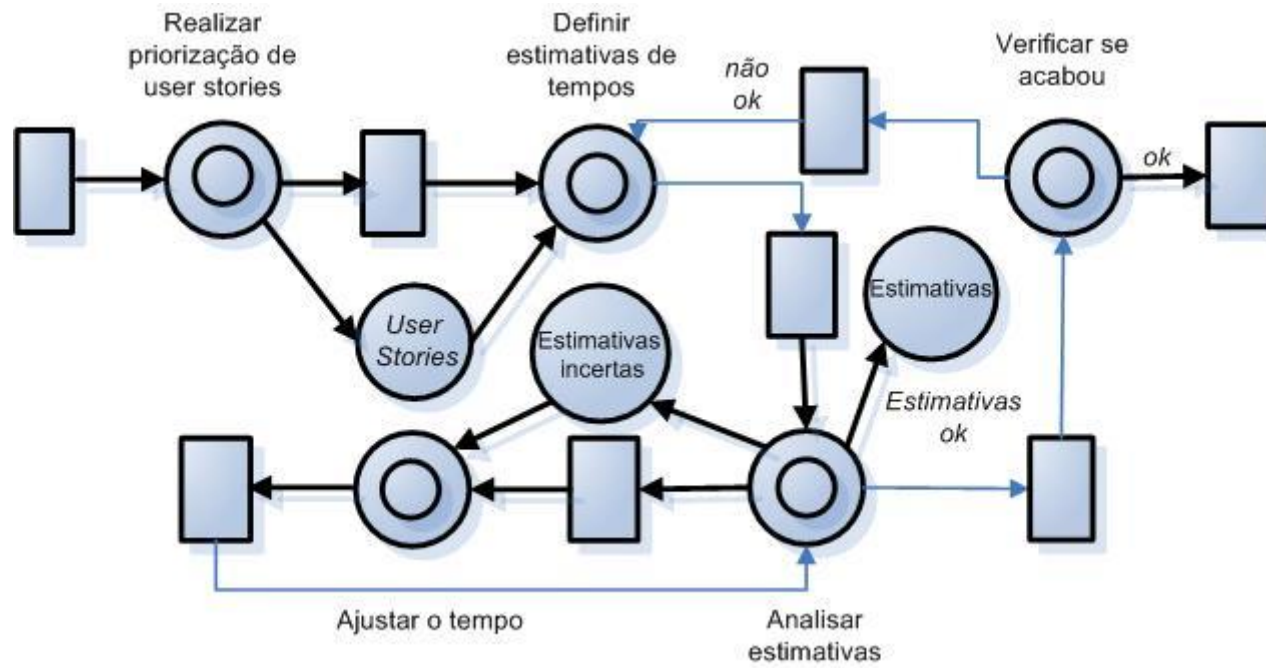
Figura 4.22: Sub-rede da atividade composta “Realizar reunião de planejamento” da figura 4.21.
