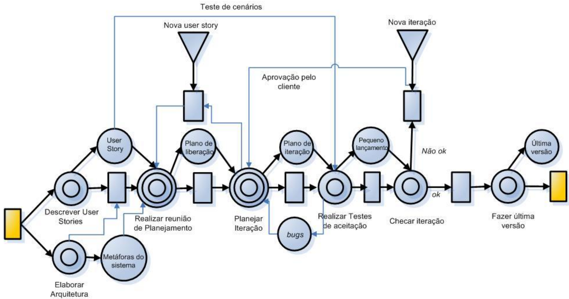
Figura 4.21: Rede de Atividades de XP
