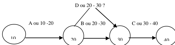
Ilustração 2.2: Diagrama de flechas para três atividades linearmente seqüenciais com inserção errada de uma atividade paralela
