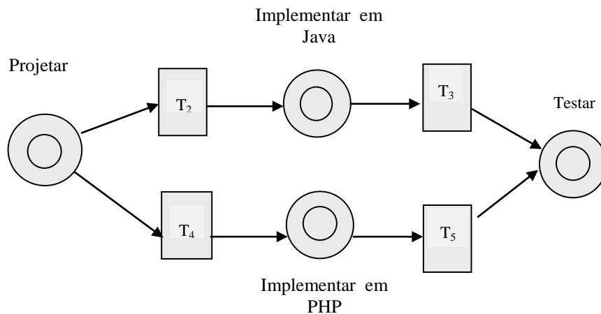
Figura 4.9: Rede de atividades com atividades alternativas Implementar em Java ou Implementar em PHP
