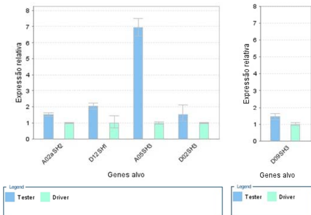
Figura 5. Expressão de genes do fungo Hydnangium sp., cultivado na presença da planta ( tester ) em relação ao fungo cultivado na ausência da planta ( driver ). O eixo x apresenta os genes alvo e o eixo y, o nível de expressão gênica correspondente à expressão dos genes alvo em relação ao calibrador ( tester ), normalizado pelo controle endógeno beta tubulina. Foram avaliados os genes que possivelmente codificam piruvato desidrogenase (A02aSH2), hidrofobina (D12SH1), ATP sintase (A05SH3), canal seletivo de íon dependente de voltagem (D02SH3) e acetil-CoA acetiltransferase (D09SH3).
