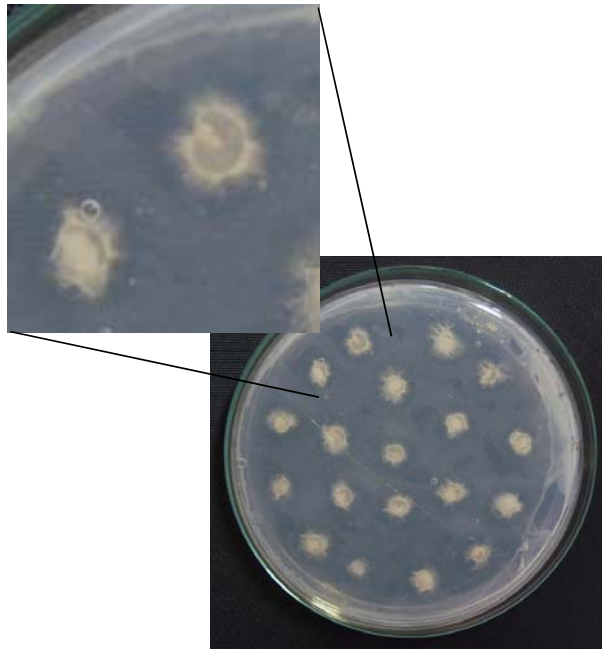
Figura 7. Inibição do crescimento da bactéria Agrobacterium tumefaciens pelo fungo Hydnangium sp. Discos de ágar contendo micélio do fungo Hydnangium sp e A. tumefaciens LBA4404, que contém o plasmídeo pCAAG3500, no meio de co-cultivo contendo meio de indução acrescido de 200 \mu M acetoseringona após 5 dias de incubação a 22 °C.
