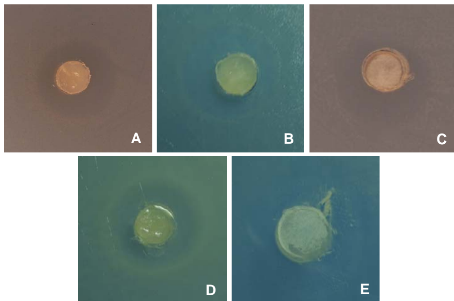
Figura 8. Inibição do crescimento das estirpes de Agrobacterium tumefaciens (A-D) e Escherichia coli \alpha hemólise por Hydnangium sp. em meio MNM contendo discos de ágar com micélio do fungo Hydnangium sp. e 200 \mu L da cultura bacteriana, após um dia de incubação a 28 °C ( A. tumefaciens ) e 37 °C ( E. coli ). A. tumefaciens LBA4404 contendo o plasmídeo pCAAG3500 (A), LBA4404 contendo o plasmídeo pBANFbar (B), AGL-1 contendo o plasmídeo pBGgHg (C) EHA105 (D) e E. coli \alpha hemólise (E).
