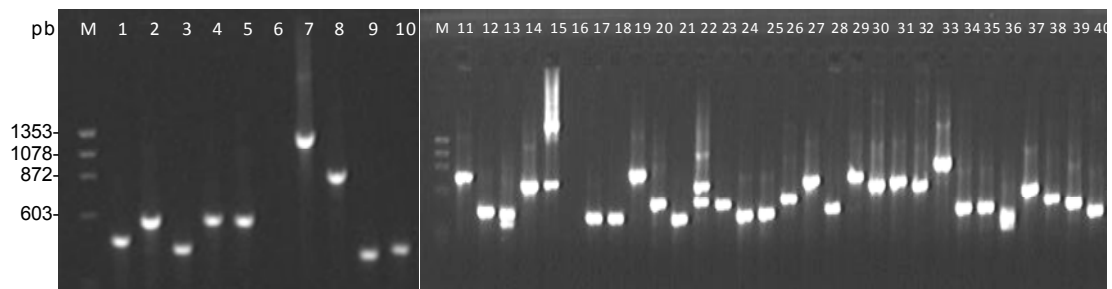
Figura 3. Polimorfismo de tamanho dos fragmentos de cDNA clonados, amplificados com os oligonucleotídeos M13F e M13R. Eletroforese em gel de agarose a 1,5 % dos produtos de amplificação. M: Marcador \phi X174/ Hae III.
