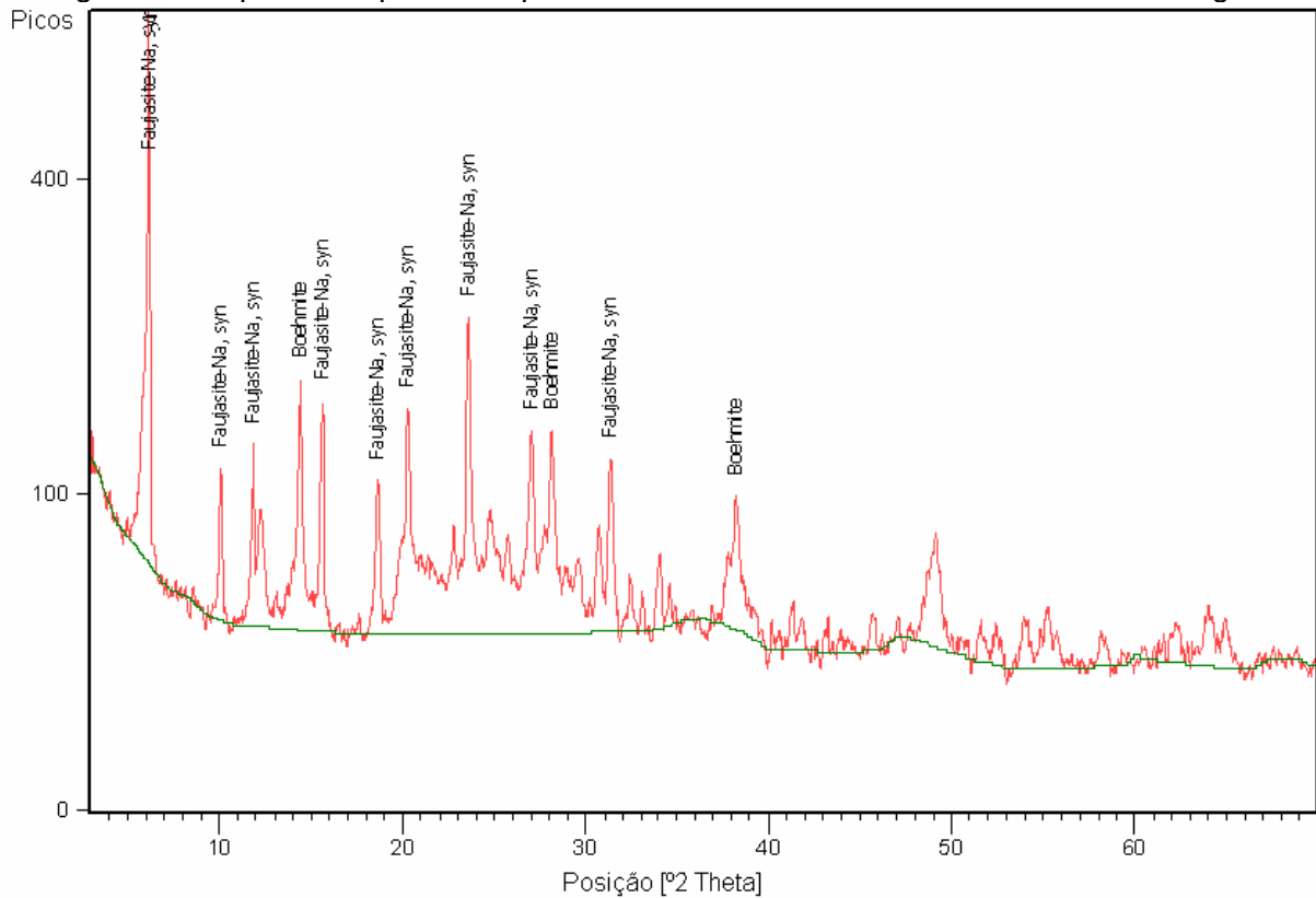
Figura 1 – Espectroscopia de Dispersão de Elétrons de amostra do catalisador virgem.
