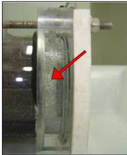
Figura 30 – Formação de H 2 na câmara catódica.
