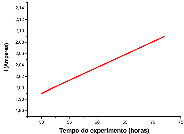
Figura 41 - Resultados do Experimento 5 – i (Âmperes) x tempo (horas).
