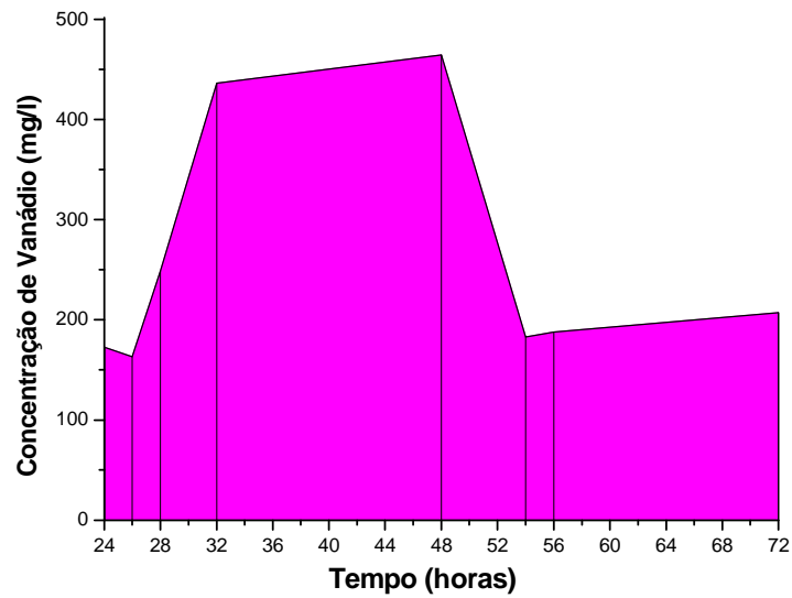
Figura 37 – Resultados do experimento 4 – Concentração de vanádio (ppm) x tempo (horas) no ponto 5 do reator.
