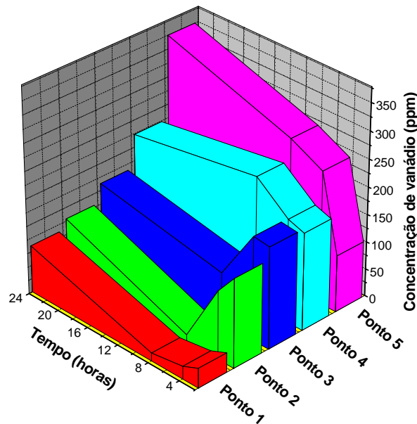
Figura 32 - Resultados do experimento 2 – Concentração de Vanádio (ppm) x tempo (horas) x Pontos.
