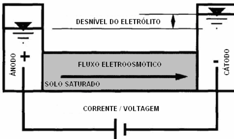
Figura 11 - Diagrama esquemático do transporte pela eletrosmose em um fluido em um solo saturado.
