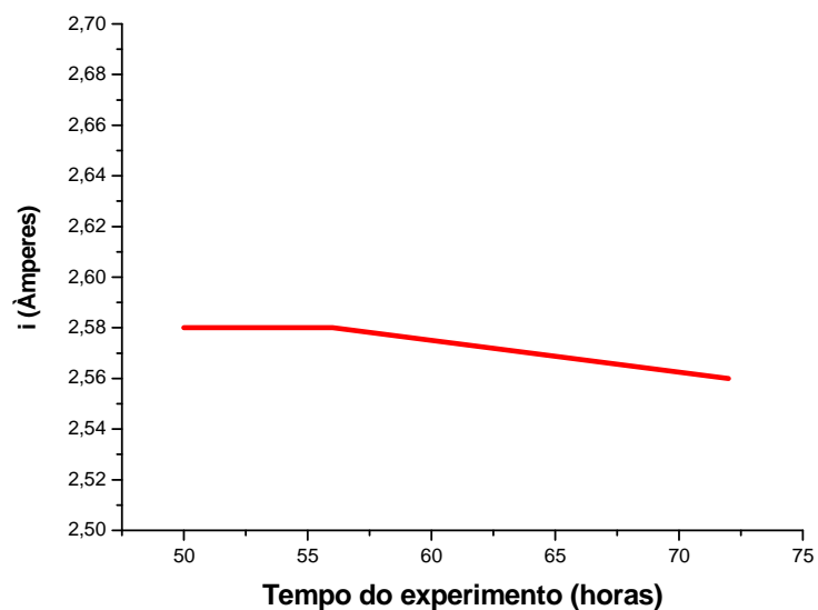
Figura 44 - Resultados Experimento 6 – i (Âmperes) x tempo (horas).
