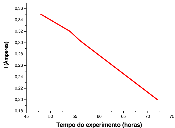
Figura 38 - Resultados Experimento 4 – i (Âmperes) x tempo (horas).
