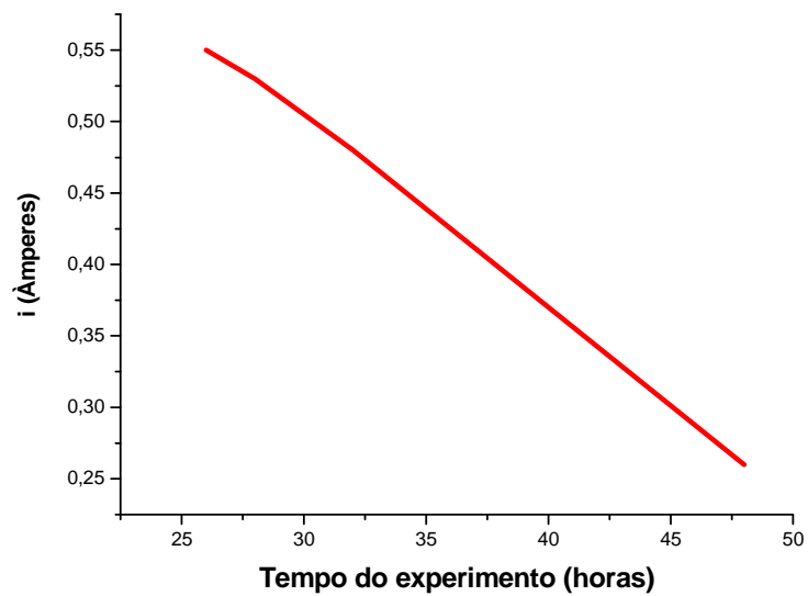
Figura 35 – Resultados do Experimento 3 – i (Âmperes) x tempo (horas).
