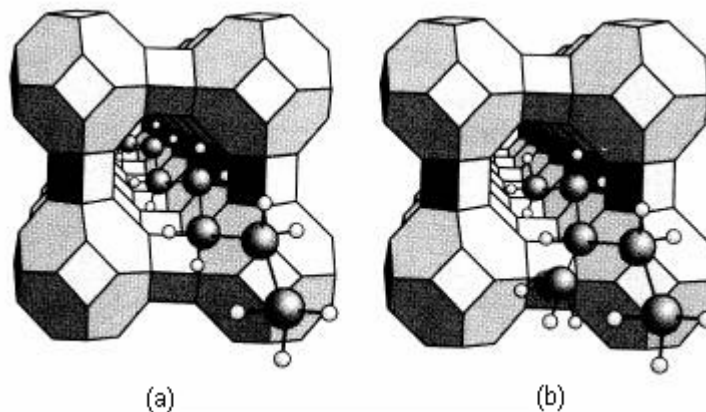
Figura 2 – Exemplos de peneiras moleculares: (a) moléculas lineares são adsorvidas pela zeólita (b) o volume excessivo da molécula ramificada impede a penetração nos poros da zeólita.
