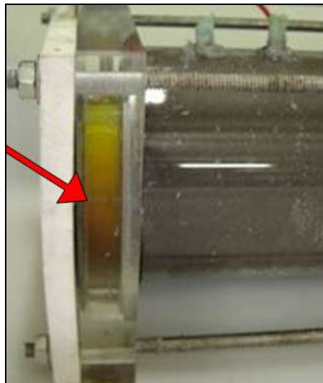
Figura 29 – Ataque ao eletrodo de aço na câmara anódica.
