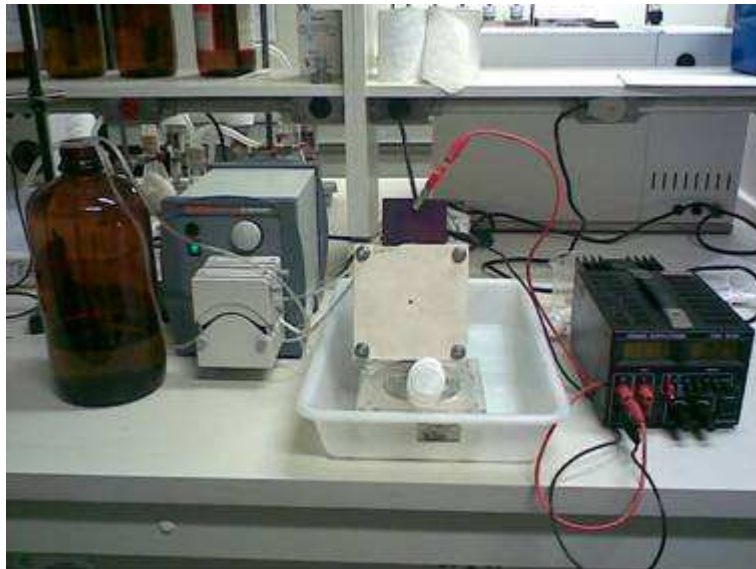
Figura 15 – Experimento montado – vista frontal – da esquerda para direita o reservatório de eletrólito, a bomba peristáltica, o reator sob bandeja e a fonte.
