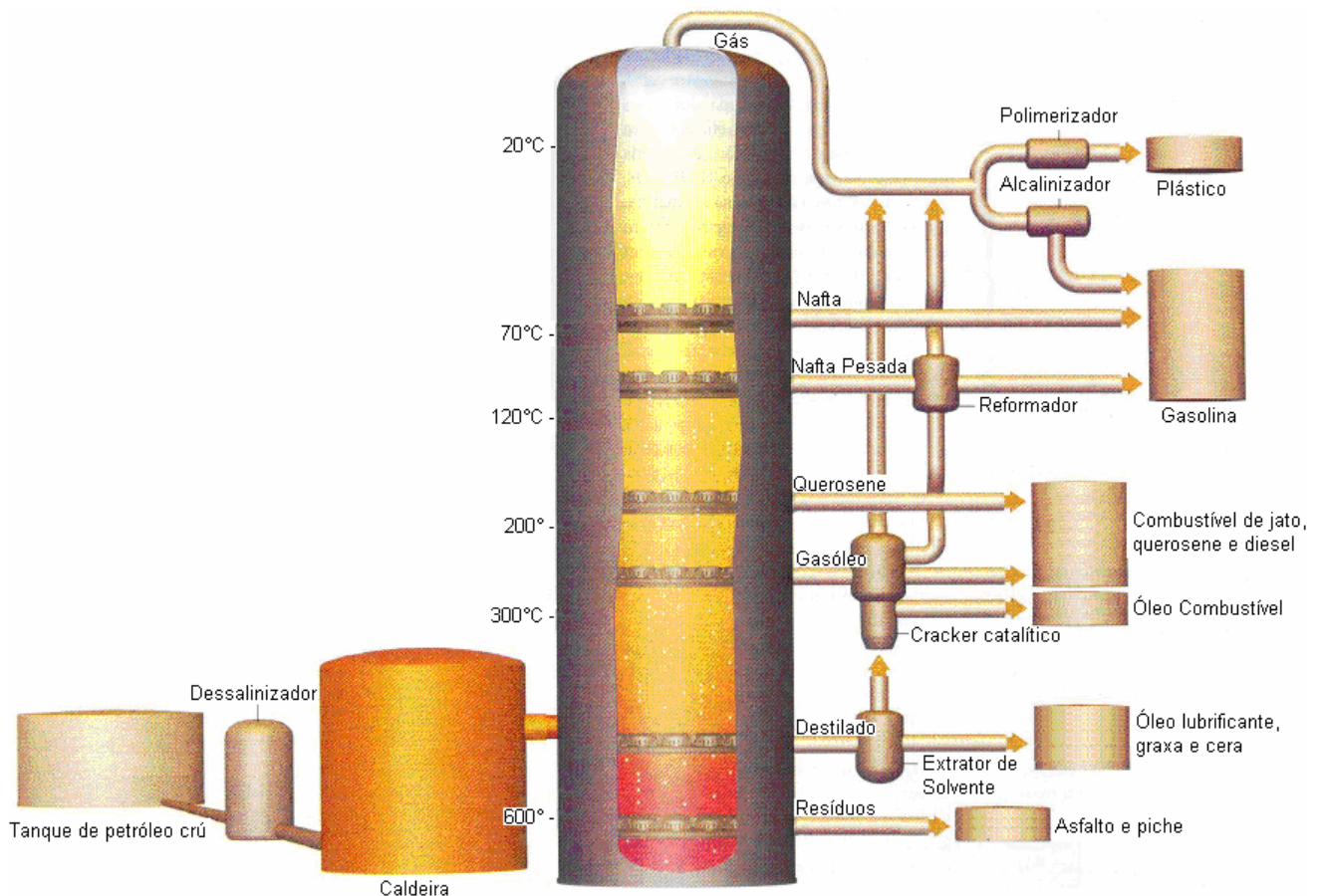
Figura 1 – Esquema de coluna fracional de destilação no processo de refino.
