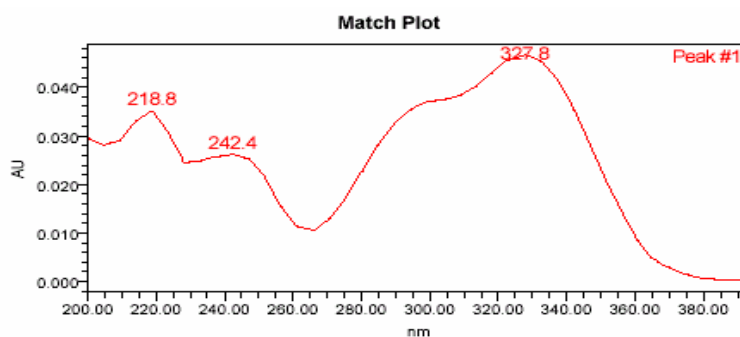
Figura 35 - Cromatograma (CLAE) da fração contendo a substância P1, obtida a partir de PS40. Coluna Shim-pack CLC-ODS (M) RP-18, fase móvel metanol:ácido fosfórico 0,16 M (53:47 v:v) fluxo 0,6 mL/min e espectro obtido por detecção no UV com arranjo de fotodiodos (Waters Alliance).
