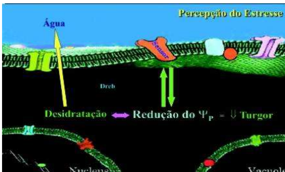
Figura 2. Esquema da percepção do estresse hídrico pelas plantas. Nepomuceno et al. (2001).
