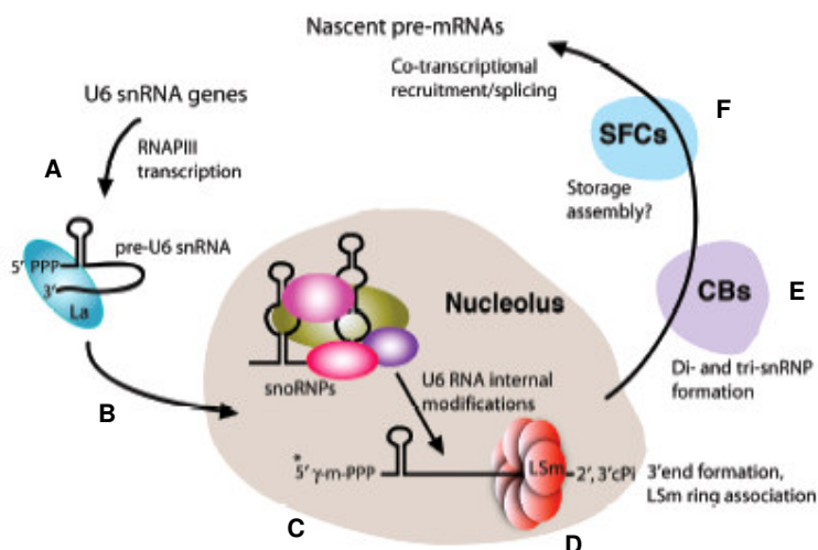
Figura 21: Biogênese de U6 snRNP em mamíferos. A) Transcrição de U6 snRNA. B) Ligação de La sinaliza para entrada no nucléolo. C) Adição do grupo metil ao cap . D) Ligação das proteínas LSm. E) Transporte para fora do nucléolo e formação dos complexos U4/U6 e U4/U6.U5. F) Armazenamento e liberação das snRNPs para montagem do spliceossomo. RNAPIII: RNA polimerase III. Patel & Bellini 2008.
