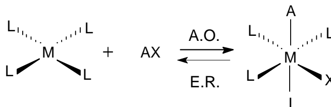
Figura 2. Adição oxidativa e eliminação redutiva em um complexo metálico.
