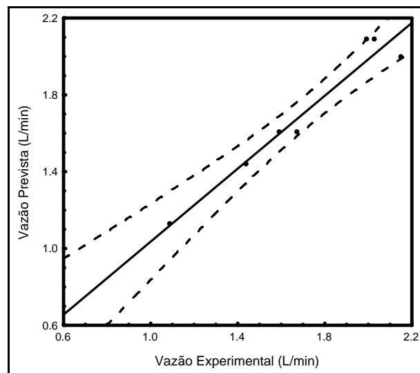
Figura 18- Vazões experimentais versus previstas para um intervalo de confiança de 98%.
