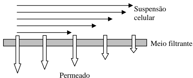
Figura 6- Filtração tangencial. A suspensão celular é alimentada tangencialmente à membrana, evitando o acúmulo de resíduos sobre a mesma (VOISARD, 2003).
