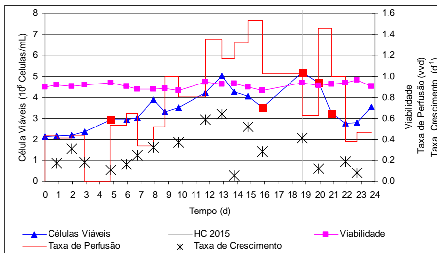
Figura 35- Progressão do cultivo em perfusão de CHO EPO utilizando os hidrociclones 2517 e 2015 em meio livre de SFB em biorreator agitado de 300L (0<t<10dias) e 150L (10<t<24). Os pontos vermelhos representam dias onde ocorreram problemas que poderiam influenciar na estabilidade do cultivo. A linha vertical mostra o momento em que o hidrociclone 2517 foi substituído pelo 2015.
