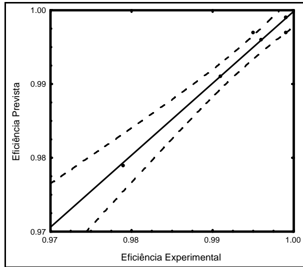
Figura 19- Eficiência de separação obtida versus previstas (Equação 4) para um intervalo de confiança de 98%.
