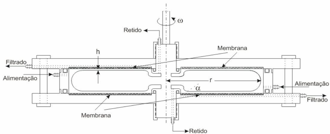
Figura 8- Esquema da unidade de filtro de disco rotativo (RDF) (CASTILHO e MEDRONHO, 2002).
