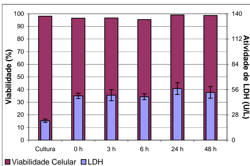
Figura 23- Dados da viabilidade celular e da concentração de LDH na cultura de CHO-GMCSF antes (Cultura) e após (0, 3, 6, 24 e 48 horas) a passagem pelo HC 1010.
