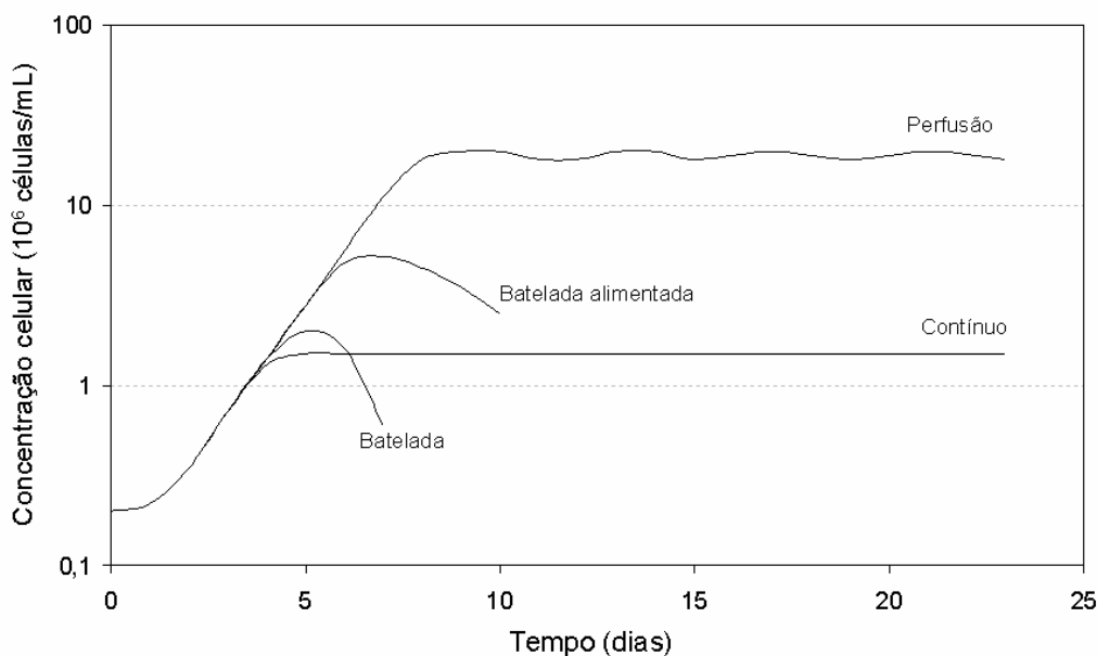
Figura 5- Comparação das concentrações celulares obtidas em função do modo de operação empregado (adaptado de Griffiths, 1992).
