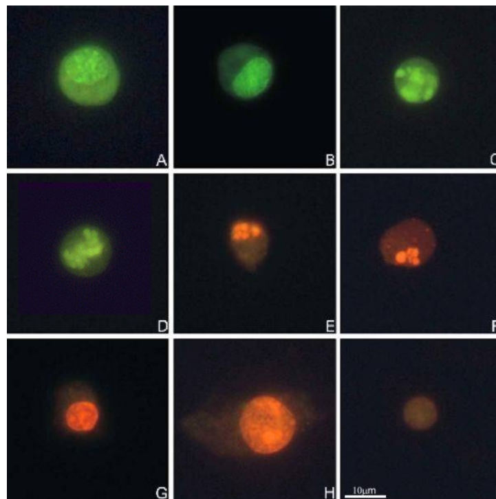
Figura 24- Morfologias observadas em microscopia de fluorescência com LA/BE. A e B, células viáveis não apoptóticas; C e D, células viáveis apoptóticas; E e F, células não viáveis apoptóticas; G e H, células necróticas; e I, célula livre de cromatina.
