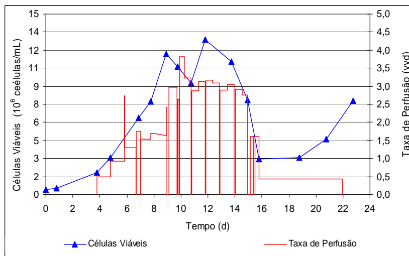
Figura 33- Progressão do cultivo em perfusão de CHO-EPO utilizando spin-filter em meio livre de SFB em biorreator agitado de 300L. Acompanhamento da concentração e taxa de perfusão em volume de vaso por dia.
