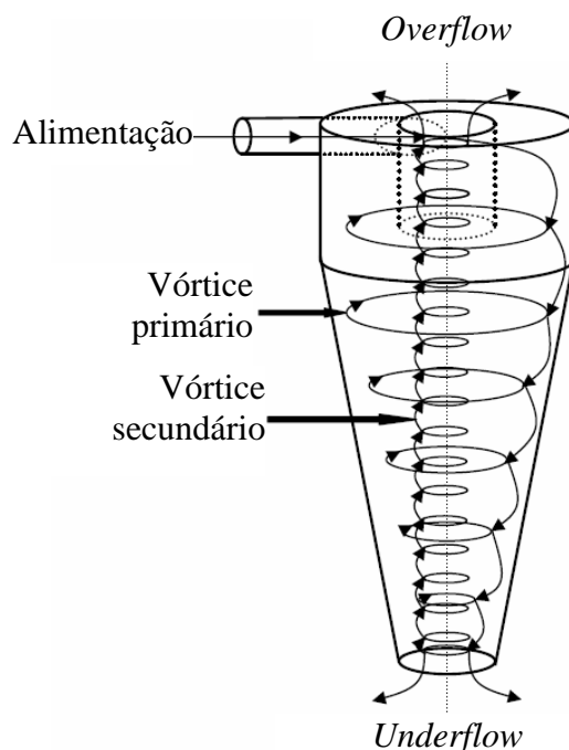
Figura 11- Vista em perspectiva de um hidrociclone e seu padrão de fluxo interno (CASTILHO e MEDRONHO, 2002).
