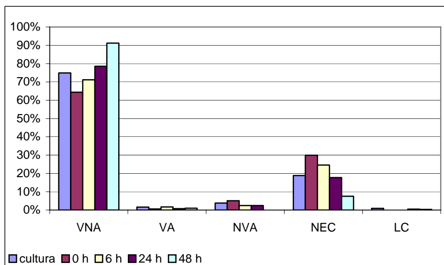
Figura 26- Acompanhamento da possível indução de apoptose na cultura de CHO.K1 após a passagem pelo HC 3020. VNA, células viáveis não apoptóticas; VA, viáveis apoptóticas; NVA, não viáveis apoptóticas; NEC, necróticas; e LC, livre de cromatina.
