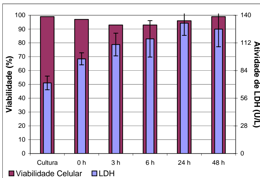
Figura 21- Dados da viabilidade celular e da concentração de LDH na cultura de CHO.K1 antes (Cultura) e após (0, 3, 6, 24 e 48 horas) a passagem pelo hidrociclone 3020.
