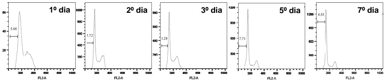
Figura 40- Acompanhamento da indução de apoptose por citometria de fluxo com iodeto de propídio em cultivo de pequena escala em roller bottles da linhagem CHO-EPO. Durante os sete dias de acompanhamento, os níveis de células apoptóticas permaneceram baixos.
