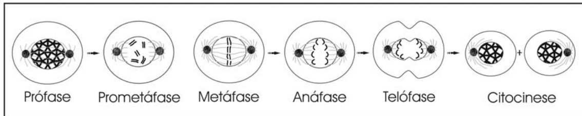
Figura 1- Os processos de divisão nuclear presentes na fase M duram menos de uma hora. Esta fase pode ser dividida em 6 etapas distintas, de acordo com o grau de progressão da divisão nuclear (prófase, prometáfase, metáfase, anáfase, telófase e citocinese). Adaptado de Alberts et al. (2002).
