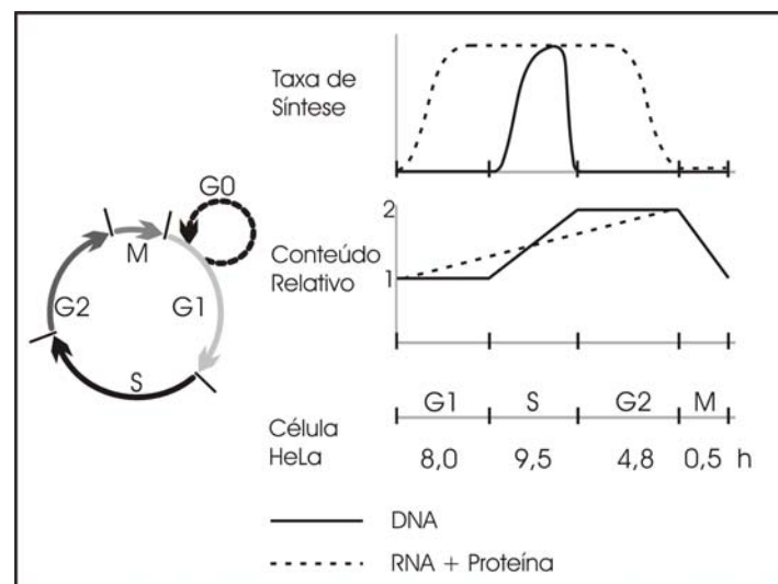
Figura 2- As fases do ciclo celular, correlacionadas com a síntese e concentração de macromoléculas na célula, assim como sua duração média no caso da linhagem tumoral HeLa (adaptado de Griffiths, 1984).
