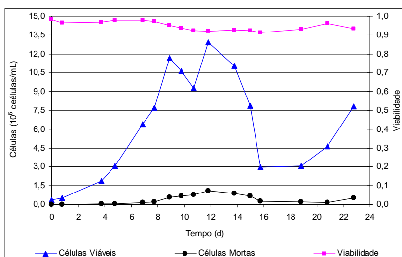
Figura 32- Progressão do cultivo em perfusão de CHO-EPO utilizando spin-filter em meio livre de SFB em biorreator agitado de 300L. Acompanhamento da concentração e viabilidade celular por azul de trypan.
