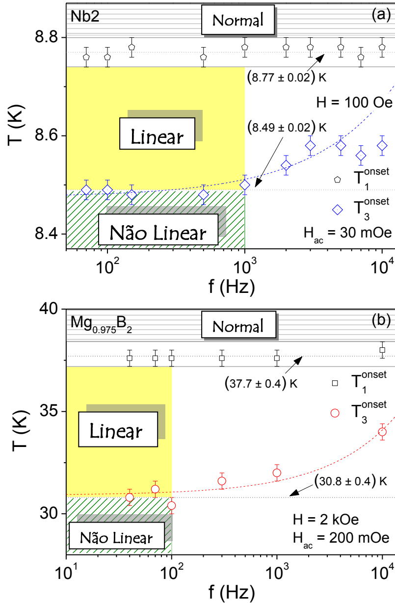
Figura 7.5. Dependência de T_1^{onset} e T_3^{onset} com f . A linha tracejada é um ajuste da equação (7.1) aos dados experimentais. Os parâmetros, T_3^{onset}(f \rightarrow 0) e \delta , obtidos foram: (a) T_3^{onset}(f \rightarrow 0) = (8.48 \pm 0.02) K e \delta = (0.73 \pm 0.04) para o sistema Nb_2 e, (b) T_3^{onset}(f \rightarrow 0) = (30.9 \pm 0.2) K e \delta = (0.67 \pm 0.03) para a amostra Mg_{0.975}B_2 . Apontamos, nas figuras, os valores aproximadamente constante de T_1^{onset} e assintótico de T_3^{onset} , obtidos mediante uma média aritmética. Note a similaridade entre o valor de T_3^{onset}(f \rightarrow 0) ajustado.
