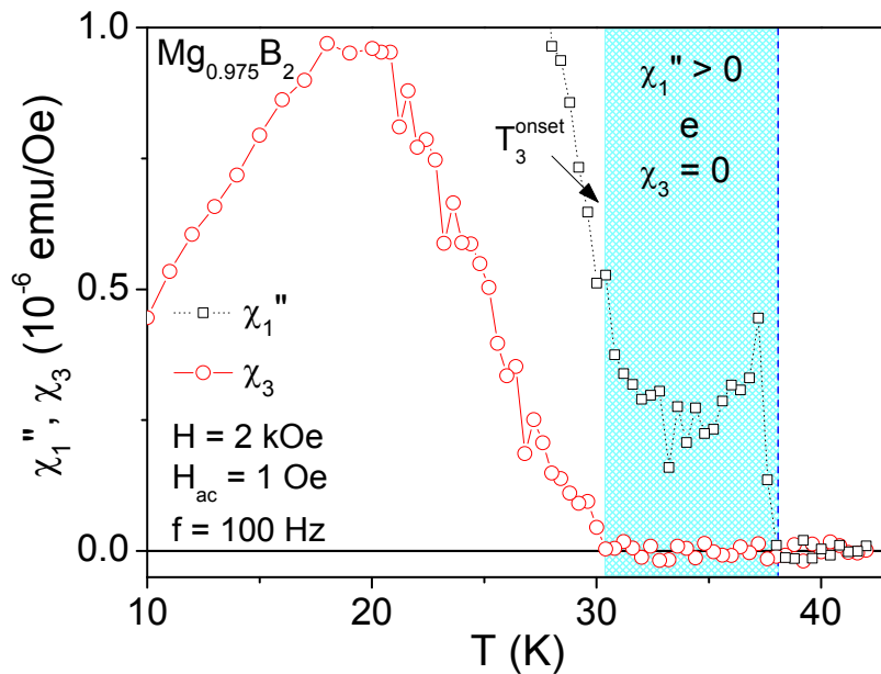
Figura 7.6. Curvas de \chi_1''(T) e \chi_3(T) para a amostra Mg_{0.975}B_2 . Os parâmetros de medida foram: H_{ac} = 1\text{ Oe} , f = 100\text{ Hz} e H = 2\text{ kOe} . Destacamos no painel a existência de um intervalo de temperaturas onde a dissipação é linear, i.e. \chi_1'' > 0 e \chi_3 = 0 .
