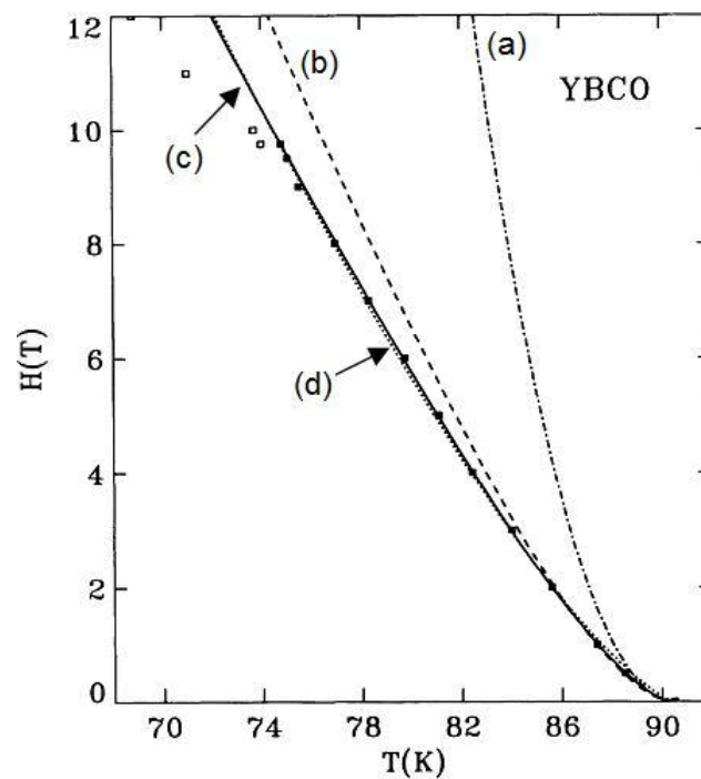
Figura 2.3. Linhas de fusão calculadas por meio do critério de Lindemann. (a) A equação (2.13) possui um intervalo de aplicabilidade muito limitado (somente próximo a T_c ). (b) A equação implícita (2.12), proposta por A. Houghton et al. [47], proporciona um bom ajuste aos dados experimentais em altas temperaturas (neste caso, c_L = 0.27 ). (c) Considerando as correções quânticas, podemos verificar uma excelente concordância entre o modelo proposto teoricamente (equação (2.14)) e os pontos experimentais. Essa adequação foi obtida para campos de até 10 T se c_L \approx 0.3 e \nu \approx 4 . (d) Ajuste da lei de potência: H_m \propto (1 - T/T_c)^n , com n \approx 1.35 .
