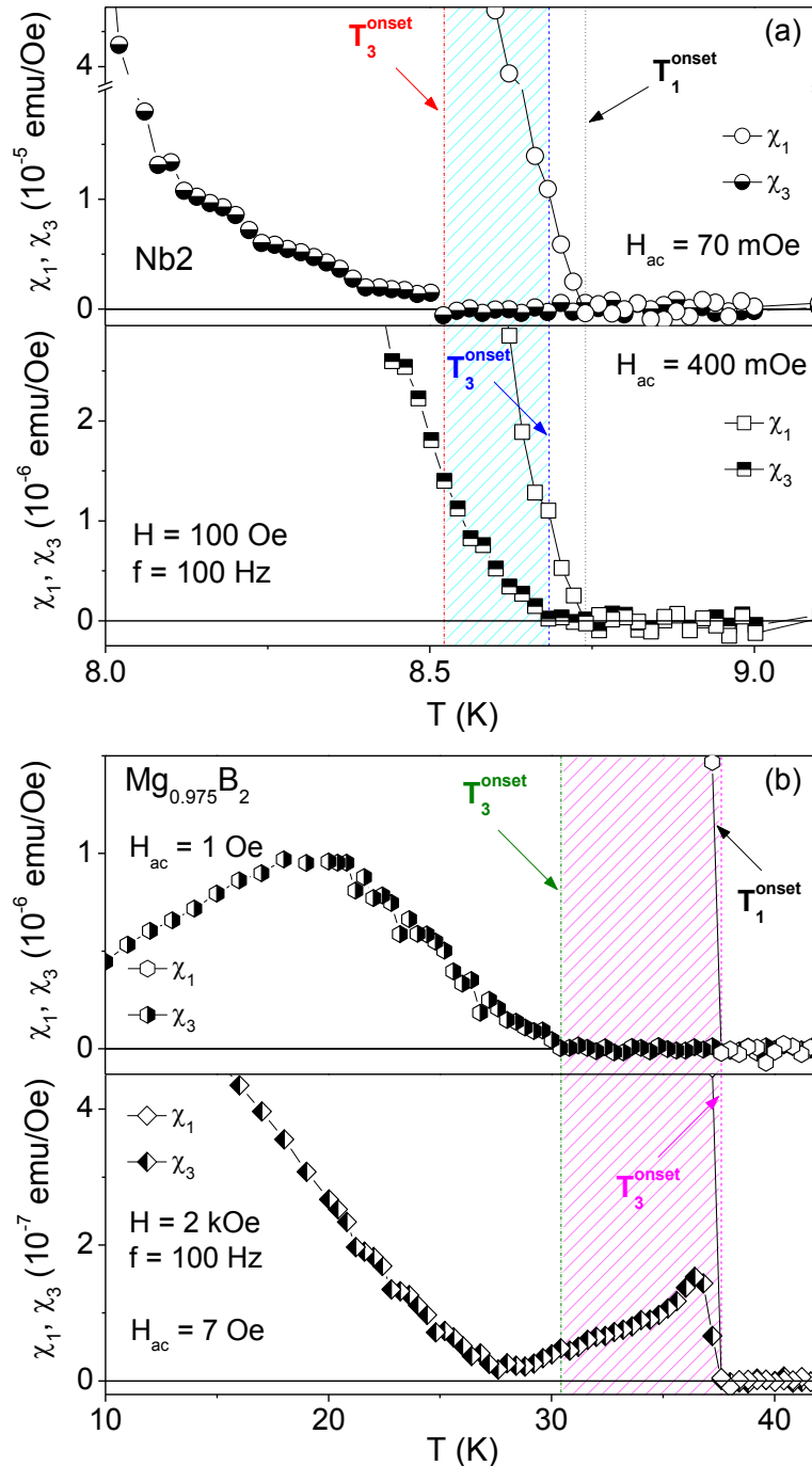
Figura 7.1. Curvas de \chi_1(T) e \chi_3(T) , para as amostras Nb_2 (a) e Mg_{0.975}B_2 (b), em diferentes amplitudes do campo ac, f = 100 Hz e H = 100 Oe (a) e 2 kOe (b). Note a diferença em T_3^{onset} à medida que H_{ac} é incrementado.
