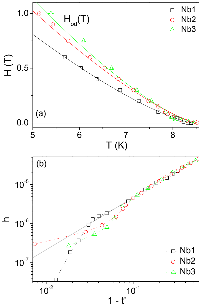
Figura 8.2. (a) Os limiares OD, H_{od}(T) , para o conjunto de amostras de Nb. As linhas sólidas são ajustes da equação (8.1) com \gamma \approx 1.3 (modelo vortex-glass ). Os parâmetros que otimizam tais ajustes são: H_0 = (26.8 \pm 0.3) \text{ kOe} e T_3^{onset}(0) = (8.43 \pm 0.02) \text{ K} para Nb1, H_0 = (33.1 \pm 0.5) \text{ kOe} e T_3^{onset}(0) = (8.54 \pm 0.04) \text{ K} para Nb2 e H_0 = (37.1 \pm 0.8) \text{ kOe} e T_3^{onset}(0) = (8.48 \pm 0.06) \text{ K} para Nb3. O painel (b) mostra as linhas OD colapsadas em uma única curva, correspondente a região de baixas temperaturas/altos campos. Em altas temperaturas, os pontos experimentais desviam desta tendência.
