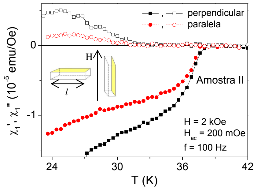
Figura 6.4. Curvas de \chi_1(T) para a Amostra II em duas diferentes geometrias: paralela e perpendicular. Os parâmetros de medição foram: H = 2 \text{ kOe} , H_{ac} = 200 \text{ mOe} e f = 100 \text{ Hz} .
