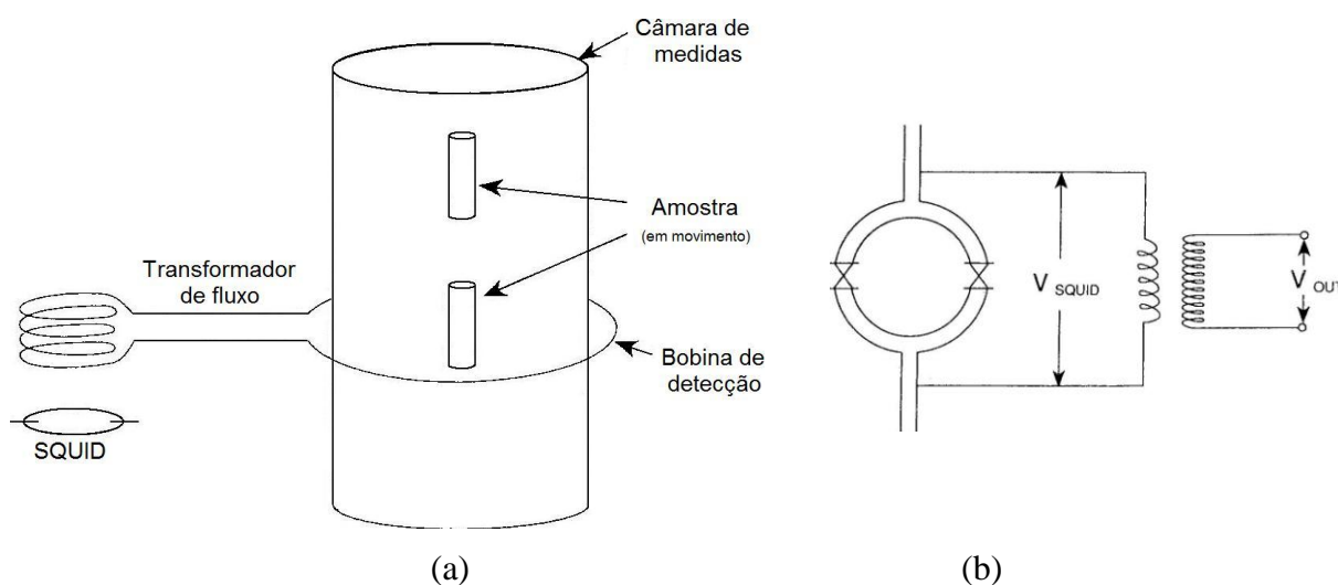
Figura 5.1. (a) Ilustração esquemática de um sistema dotado de um SQUID . (b) SQUID de duas junções em paralelo.
