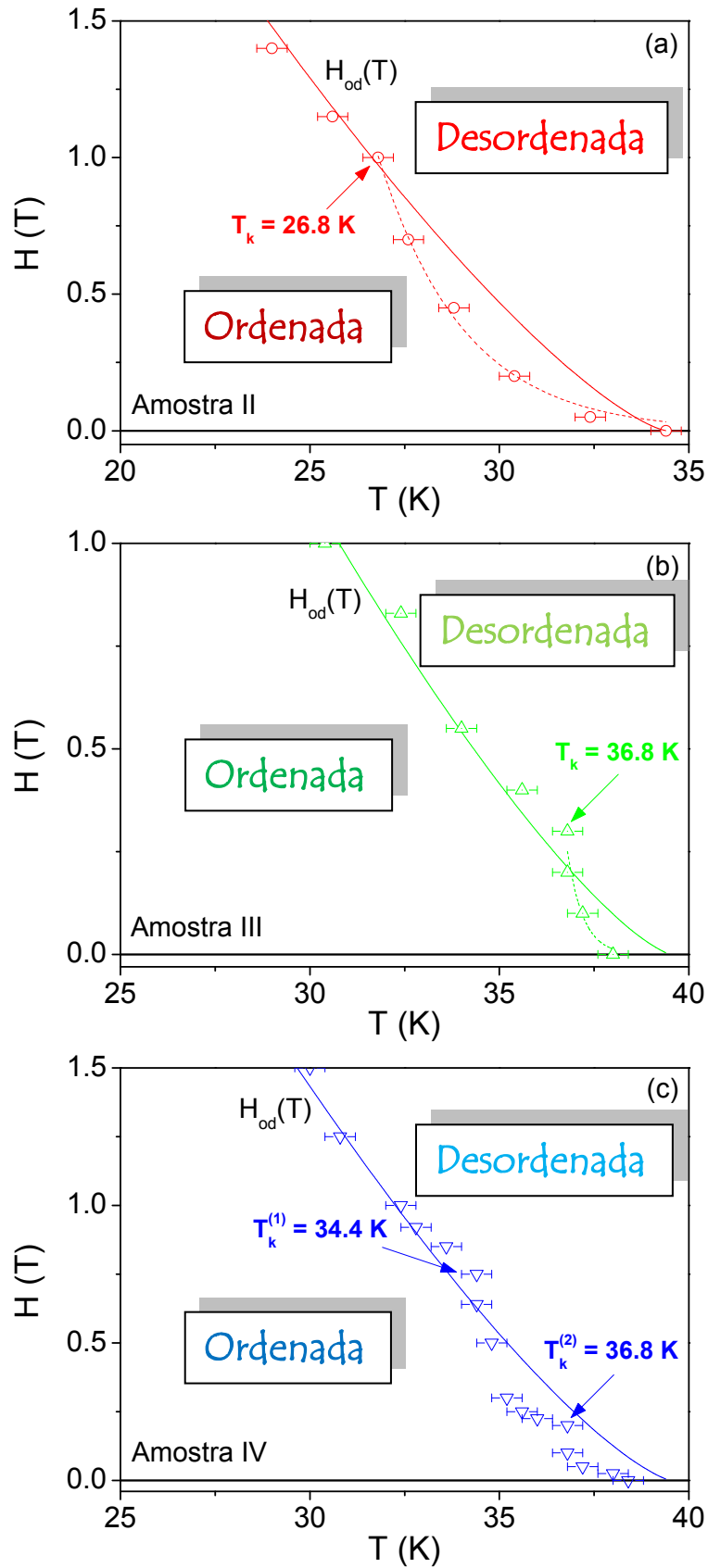
Figura 9.4. Ampliação do diagrama de fases HT ilustrado na Figura 9.1(a). A linha tracejada é um ajuste da equação (8.2) aos dados de altas temperaturas com: (a) A = (1.37 \pm 0.03) 10^7 0e/K^2 e T_0 = (1.94 \pm 0.09) K , (b) A = (1.7 \pm 0.2) 10^{40} 0e/K^2 e T_0 = (0.4 \pm 0.1) K . A temperatura T_k está indicando o início da Transição de Depinning Induzida Termicamente .
