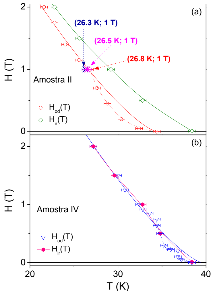
Figura 9.6. Comparação entre os limiares H_{od}(T) e H_{ir}(T) obtidos para as amostras II (a) e IV (b). Para a determinação de H_{ir}(T) , empregamos a técnica M(T) .
