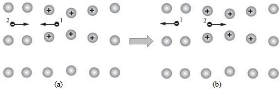
Figura 1.4. Representação esquemática da interação elétron-fônon. (a) O elétron 1 produz uma região polarizada na rede cristalina ao se mover através do material. (b) Na porção deformada da rede haverá um acúmulo de cargas positivas que atrairá o elétron 2.
