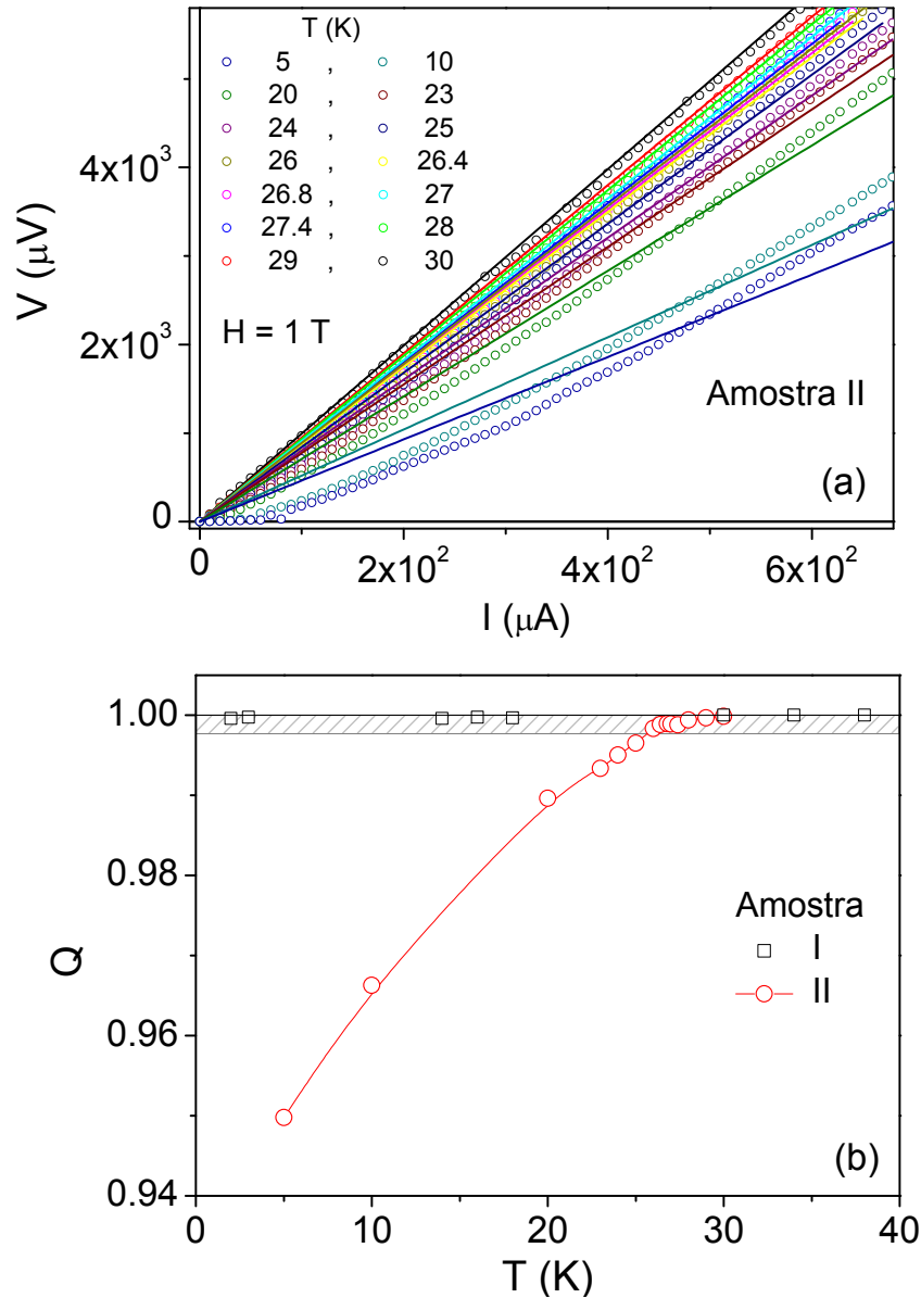
Figura 9.8. (a) Diagrama IV , obtido em H = 1 T, para a Amostra II. (b) Qualidade dos ajustes, mostrados em (a) e na Figura 9.9, em função de T .
