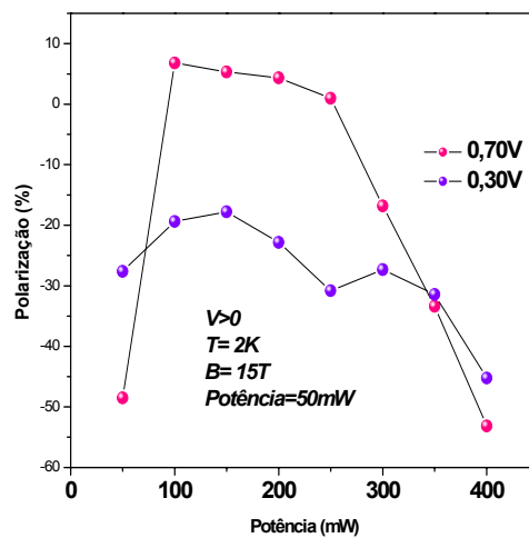
Figura 4.1.8: Efeito da Polarização com a potência em tensões fixas de 0,30 e 0,70V à 15T.
