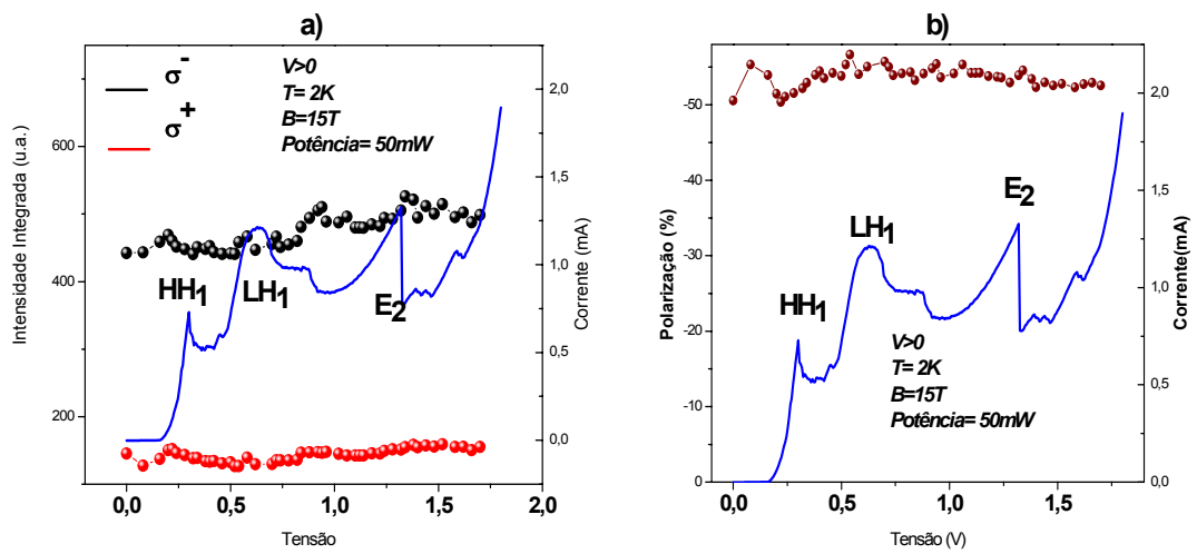
Figura 4.2.20 : Curvas de a) intensidade integrada e b) polarização para a emissão da região do contato GaAs em função da voltagem aplicada , com B=15T e sob excitação do laser de 50mW.
