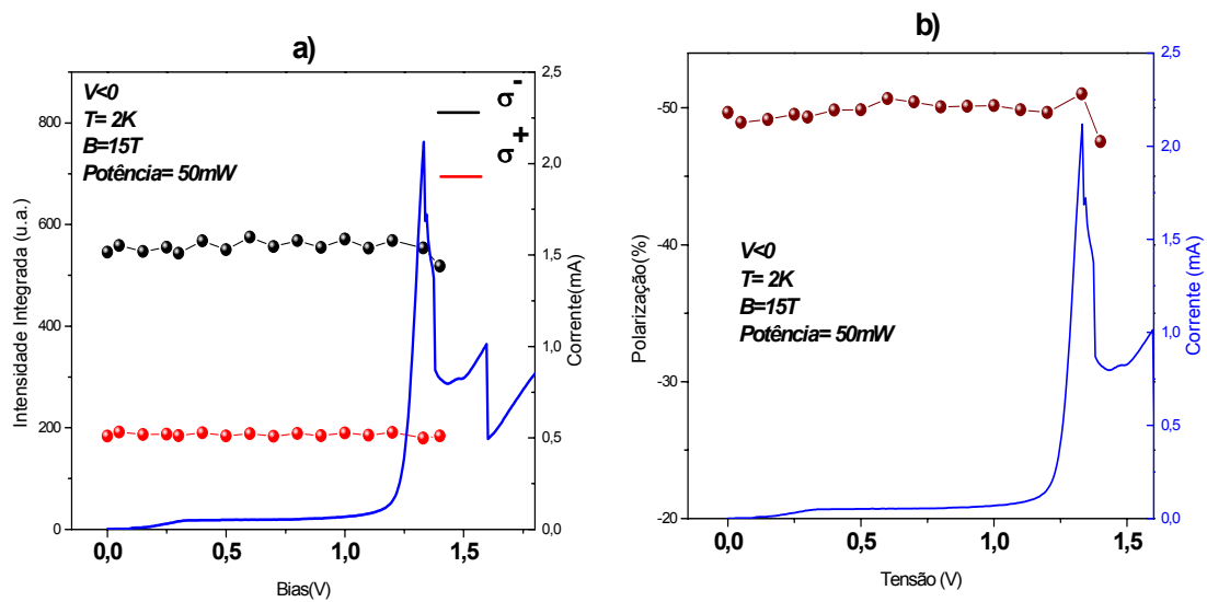
Figura 4.2.28: Curvas de a) intensidade integrada e b) polarização, em função da voltagem aplicada e para potência de 50mW.
