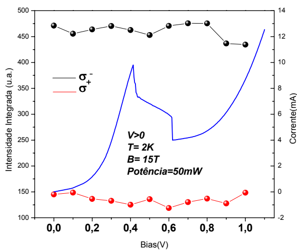
Figura 4.1.11: Curvas de Intensidade Integrada em função da tensão aplicada.
