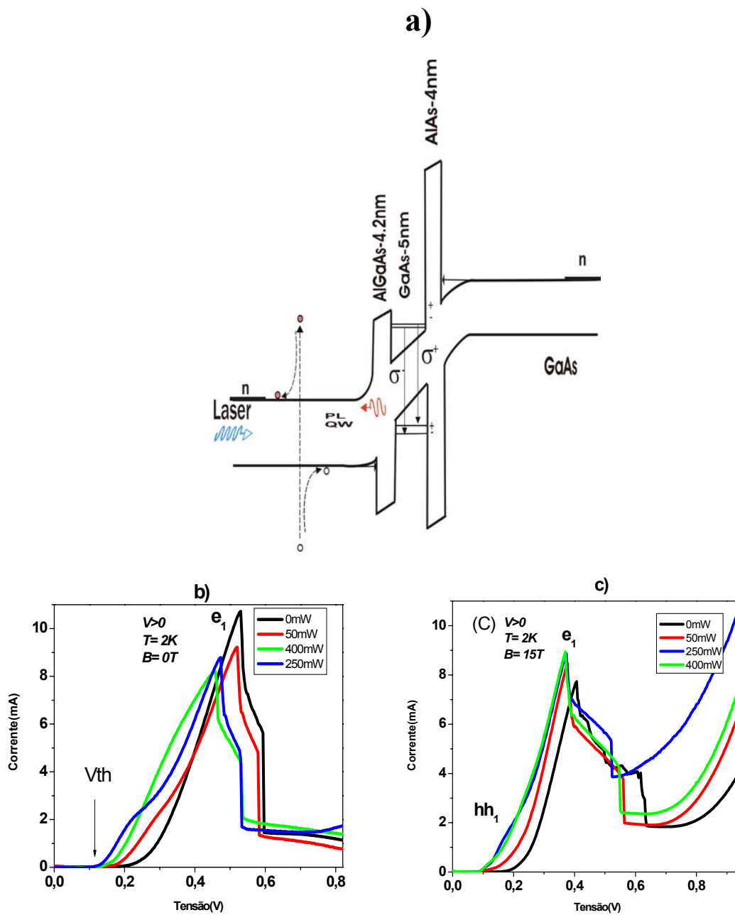
Figura 4.1.1: a) Esquema do perfil de potencial da amostra NU454; b) Curvas de corrente e tensão para diversas potências de excitação do laser sem campo magnético aplicado; c)
