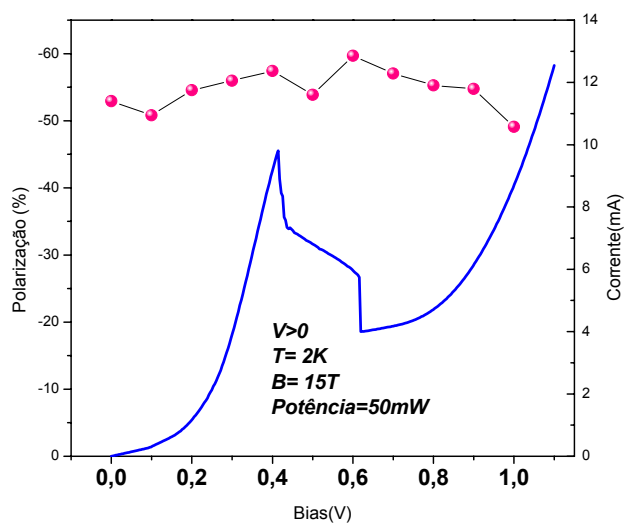
Figura 4.1.12: Polarização em função da tensão aplicada para potência de 50mW e B=15T .
