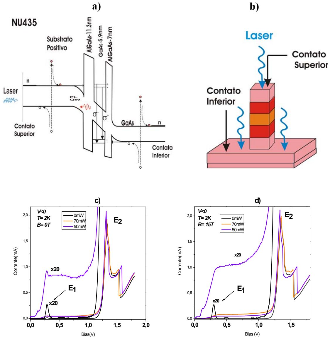
Figura 4.2.7: a) Ilustração da incidência de luz no diodo b) Esquema do perfil de potencial da amostra NU454 quando submetida a um potencial negativo (substrato positivo); c) Curvas de corrente e tensão para diversas potências de excitação do laser sem campo magnético aplicado; d) Curvas de corrente e tensão para diversas potências de excitação do laser com campo magnético aplicado.
