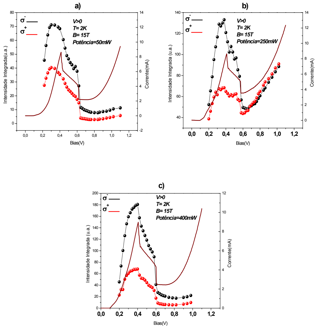
Figura 4.1.6: Curvas de Intensidade Integrada em função da voltagem aplicada para potências de a)50mW, b)250mW e c) 400mW.
