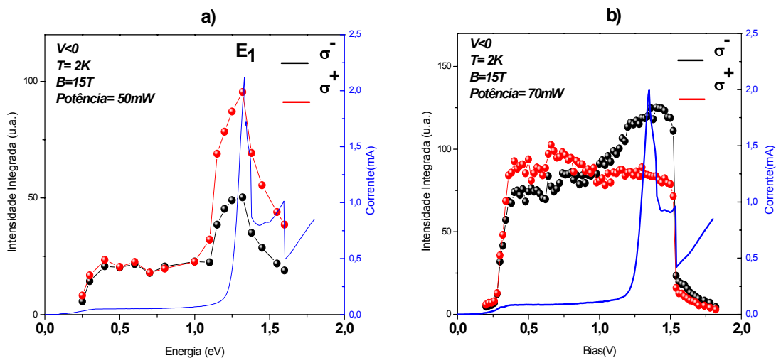
Figura 4.2.24 : Curvas de intensidade integrada em função da voltagem aplicada para potências de a)50mW e b)70mW.
