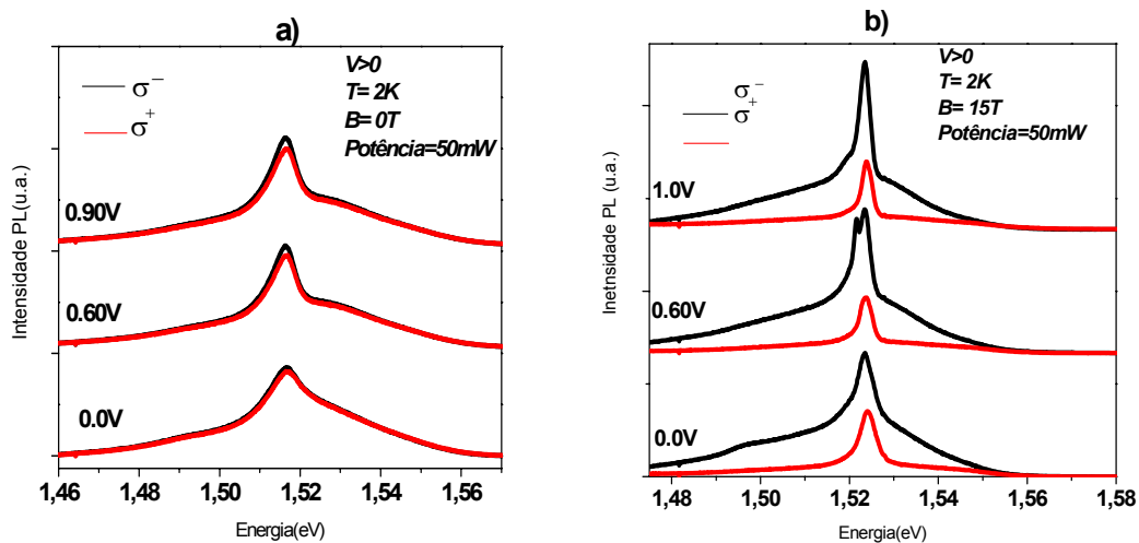
Figura 4.1.9: Espectros de PL da emissão do contato GaAs para diferentes voltagens aplicadas, sob excitação de 50mW e (a) B=0T e (b) B=15 .
