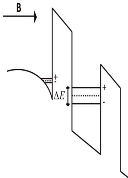
Figura 2.1.11: Esquema dos níveis eletrônicos da estrutura sob a aplicação de campo magnético e considerando o spin dos portadores nas duas regiões de confinamento.
