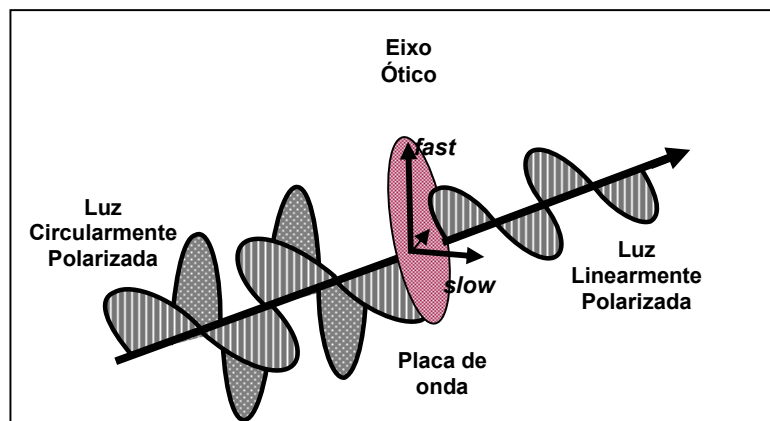
Figura 5: Ilustração de uma luz circularmente polarizada sendo transformada em luz linearmente polarizada através de uma placa de um quarto de onda ( \lambda/4 ).
