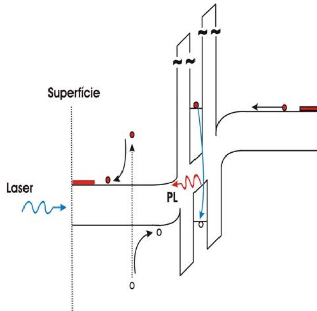
Figura 2.1.12: Esquema do perfil de potencial de um DTR, com dopagem n-i-n, quando submetido a um potencial positivo (substrato negativo) e incidência de laser.
