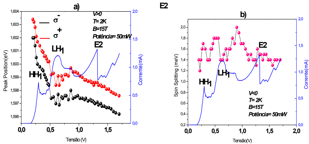
Figura 4.2.11: a) Varição da posição dos picos dos espectros de PL em função da voltagem e b) Spin-Splitting em função da voltagem, para potência de excitação do laser de 50mW e B=15T .
