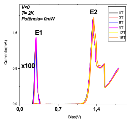
Figura 4.2.8 : Curva I(V) para diferentes valores de campo magnético na ausência de excitação óptica.
