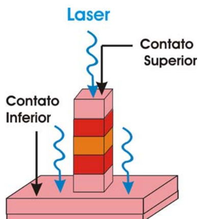
Figura 4.2.1: Ilustração da incidência de luz no diodo.
