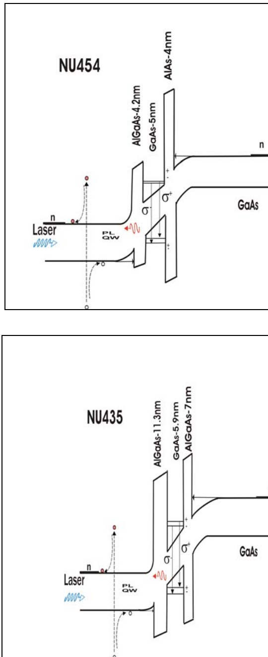
Figura 3.1.1: Perfil de Potencial de diodos de dupla barreira do tipo n-i-n: (a) Cada barreira é formada de materiais diferentes ( AlGaAs e AlAs), ocasionando uma assimetria em suas alturas. (b) Barreiras de AlGaAs, mas com diferentes larguras (11.3 e 7nm)
