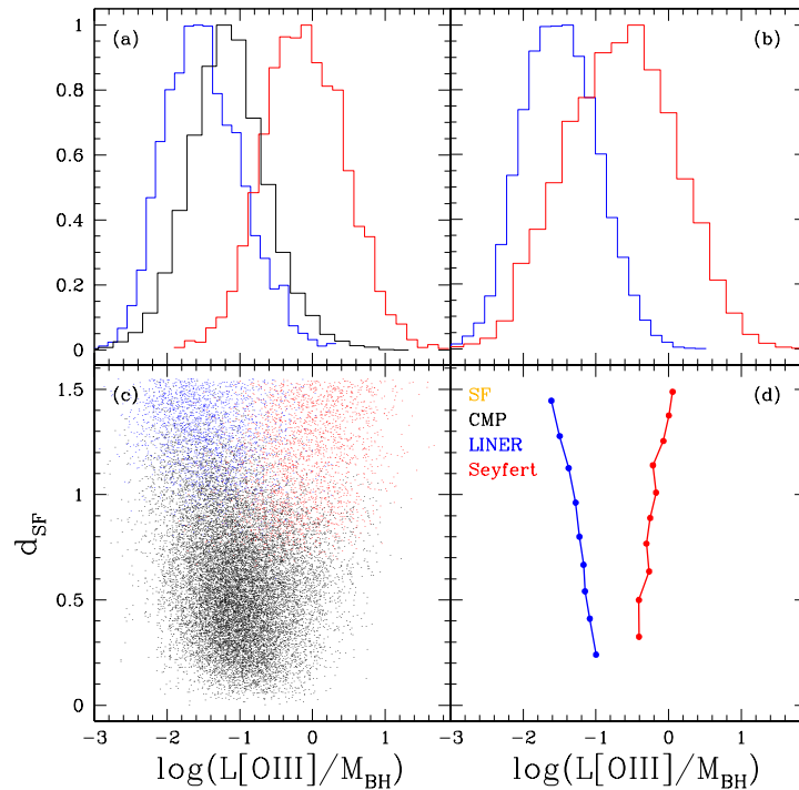
Fig. 3.18: Assim como na figura 3.6, aqui para \log(L_{[\text{OIII}]} / M_{\text{BH}}) , em unidades de L_{\odot} / M_{\odot} .
