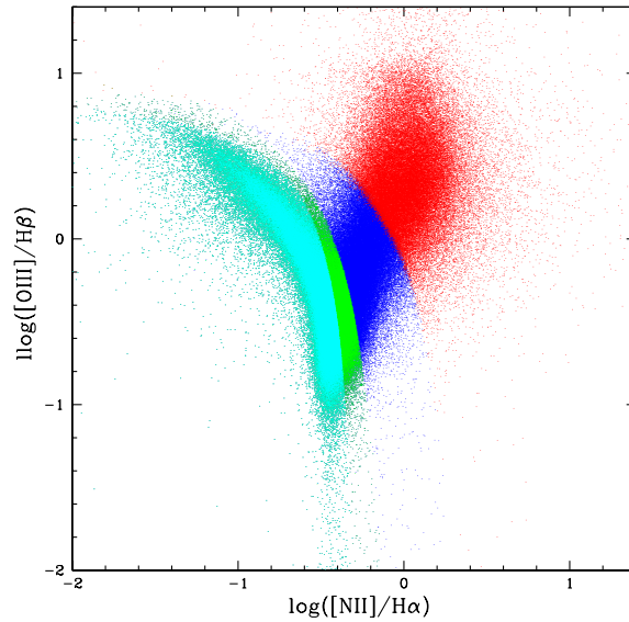
Fig. 1.3: Diagrama BPT para as galáxias do SDSS. Exigimos S/N > 3 nas linhas [N II] , H\alpha , [O III] e H\beta . As diferentes cores marcam a classificação das galáxias conforme descrito no texto.
