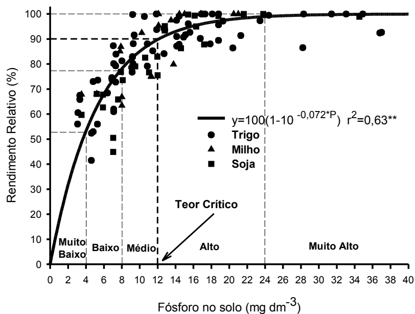
FIGURA 31. Teor crítico de fósforo no solo, determinado por Mehlich -1 , na média de rendimentos de trigo, milho e soja sob sistema plantio direto, amostrado na profundidade de 0-10 cm. Todos os experimentos (M1, M2, I1, I2, AP1, AP2 e PJC). ** Significativo ( P < 0,01 ).
