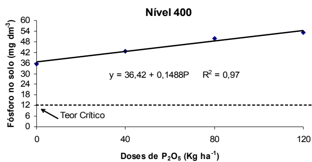
FIGURA 83. Teor de P extraído por Mehlich 1 , equações de resposta do solo a aplicação de \text{P}_2\text{O}_5 nos diferentes níveis criados, experimento AP2 soja, na safra 2005/2006.
