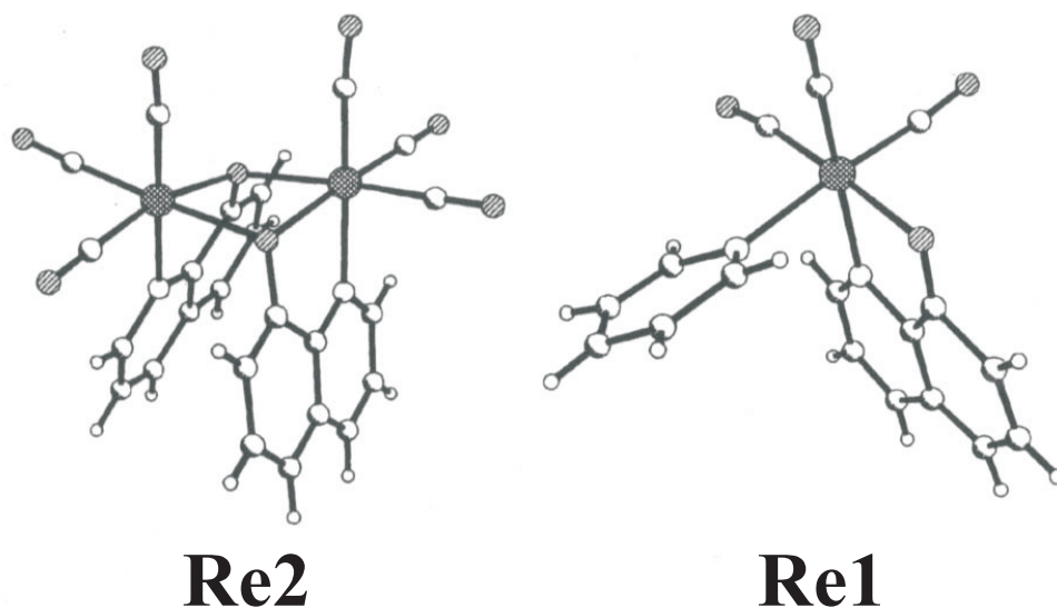
Figura A.1: Estruturas dos complexos Re(I)(tricarboxyl)(8\text{-quinolato}) dimérico (esquerda) e monomérico em piridina (direita). Figura extraída da referência [84].
