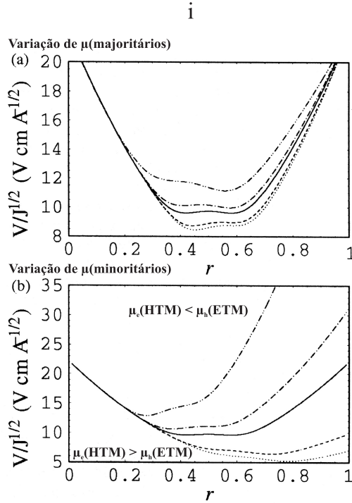
Figura 1. Condição de otimização para n = n' = 6 . A linha contínua em (a) e (b) representa as mobilidades: \mu_c(0) = 10^{-3} \text{ cm}^2 \text{ V}^{-1} \text{ s}^{-1} ; \mu_h(0) = 10^{-6} \text{ cm}^2 \text{ V}^{-1} \text{ s}^{-1} ; \mu_c(1) = 10^{-3} \text{ cm}^2 \text{ V}^{-1} \text{ s}^{-1} ; \mu_h(1) = 10^{-6} \text{ cm}^2 \text{ V}^{-1} \text{ s}^{-1} . Para as outras curvas em (a), \mu_c(0) muda para 5 \times 10^{-3} \text{ cm}^2 \text{ V}^{-1} \text{ s}^{-1} (---), 10^{-2} \text{ cm}^2 \text{ V}^{-1} \text{ s}^{-1} (---), 5 \times 10^{-4} \text{ cm}^2 \text{ V}^{-1} \text{ s}^{-1} (---) e 10^{-4} \text{ cm}^2 \text{ V}^{-1} \text{ s}^{-1} (---). Para as outras curvas em (b) \mu_c(1) muda para 5 \times 10^{-6} \text{ cm}^2 \text{ V}^{-1} \text{ s}^{-1} (---), 10^{-5} \text{ cm}^2 \text{ V}^{-1} \text{ s}^{-1} (---), 5 \times 10^{-7} \text{ cm}^2 \text{ V}^{-1} \text{ s}^{-1} (---) e 10^{-7} \text{ cm}^2 \text{ V}^{-1} \text{ s}^{-1} (---).
