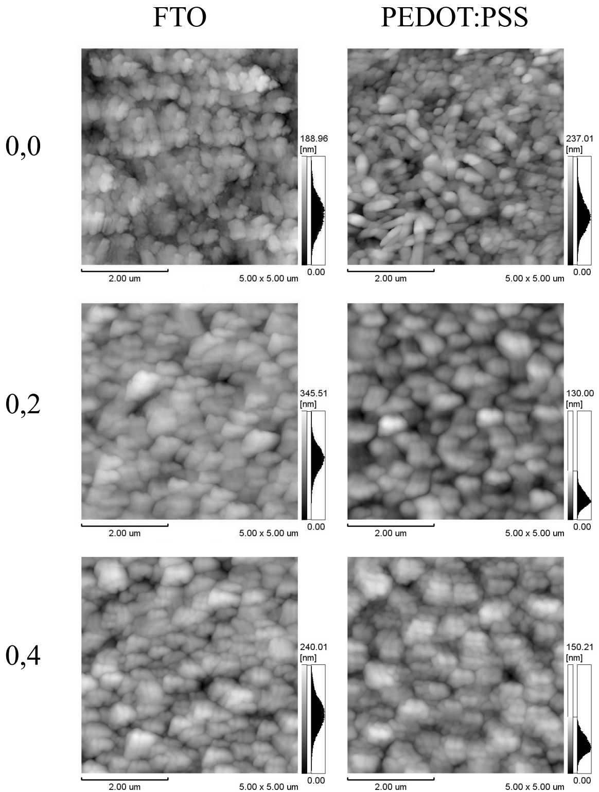
Figura 3.12: Imagens de AFM obtidas no modo dinâmico de filmes 0,0, 0,2 e 0,4 [Alq 3 ] em substratos de FTO e PEDOT:PSS. A área das imagens é 5 μm × 5 μm.
