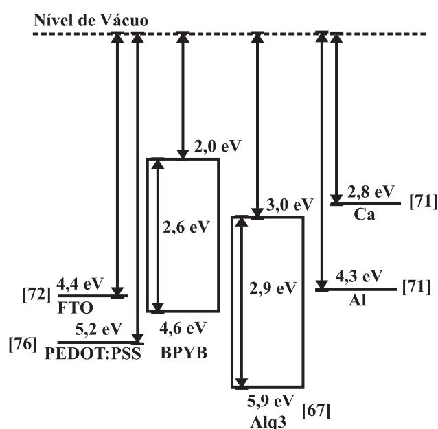
Figura 3.5: Diagrama de energias proposto para a molécula BPYB, além do diagrama do Alq 3 e das funções trabalho dos eletrodos utilizados.
