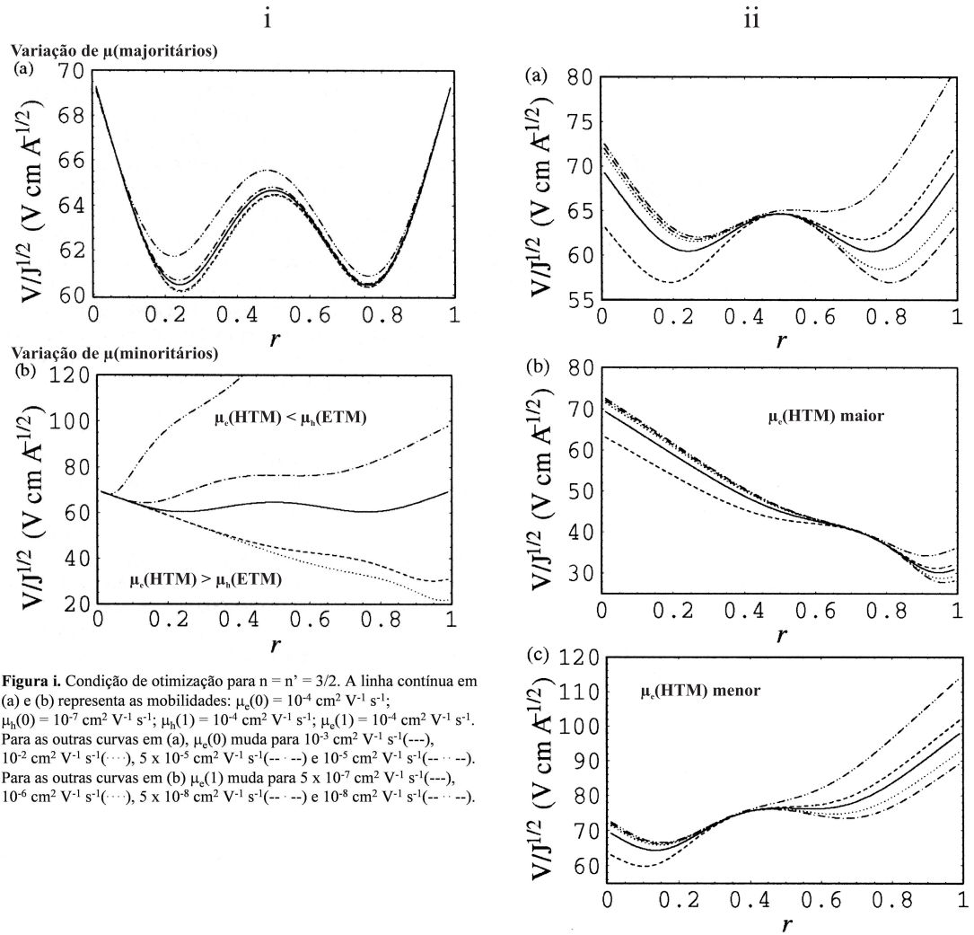
Figura ii. Condição de otimização para n = n' = 3/2 e diferentes B_c e B_a , sendo B_c/B_a = 0,9995/0,0005 (---); 0,9999/0,0009 (- · - ·); 0,9992/0,0002 (.....); 0,9991/0,0001 (- - - -); 0,999/0,004 (- · - · -). Em (a) todas as curvas são calculadas considerando as mesmas mobilidades para a linha contínua na figura i(a). Em (b) e (c) \mu_c(1) muda, respectivamente, para 5 \times 10^{-7} \text{ cm}^2 \text{ V}^{-1} \text{ s}^{-1} e 5 \times 10^{-8} \text{ cm}^2 \text{ V}^{-1} \text{ s}^{-1} .
