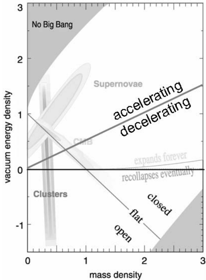
Figura 3.7: Parâmetros de densidade do Universo [41].
